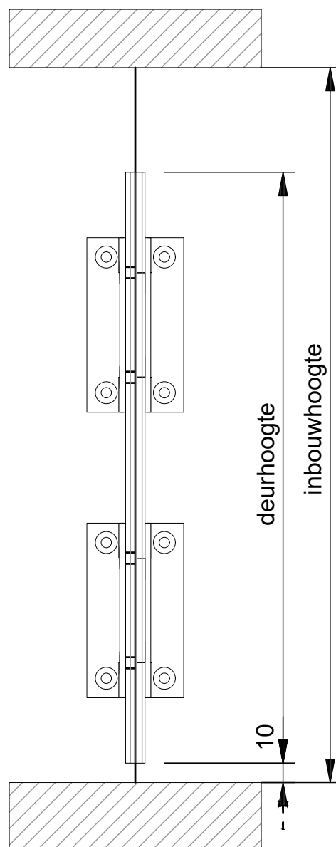
VERTICALE DOORSNEDE type DOD-1
