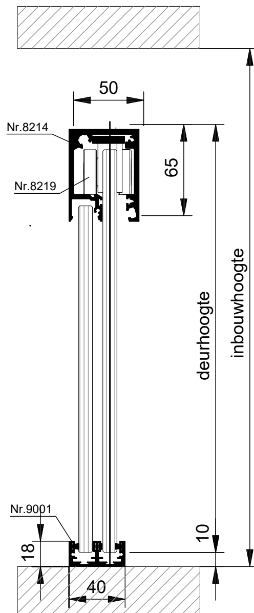
VERTICALE DOORSNEDE type DSD-1
