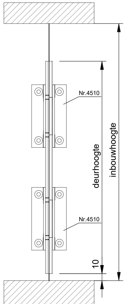
VERTICALE DOORSNEDE type DOD-21
