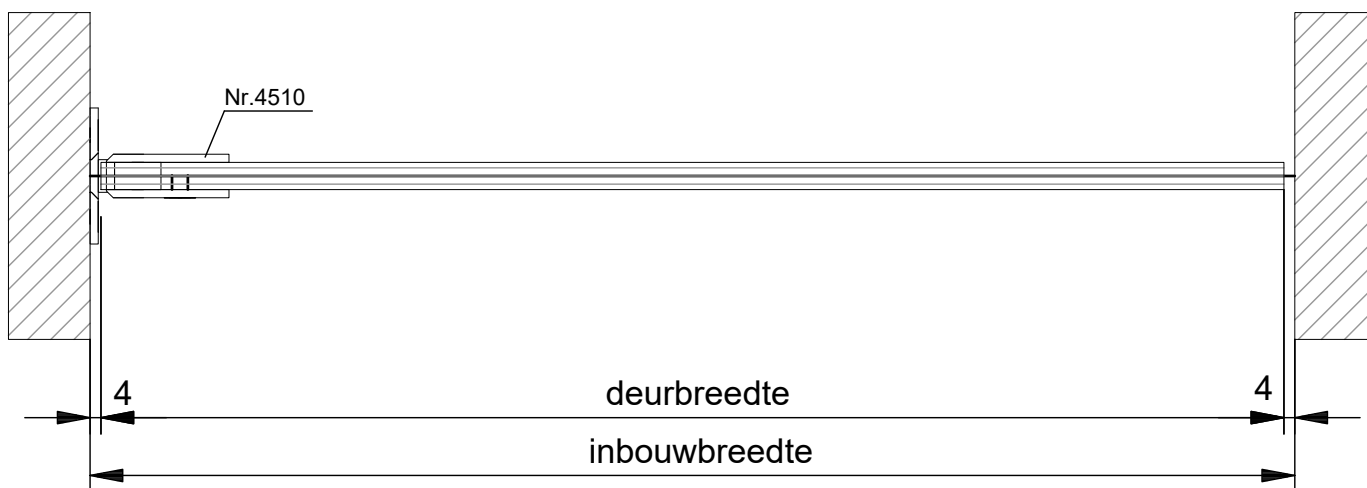
HORIZONTALE DOORSNEDE type DOD-1
