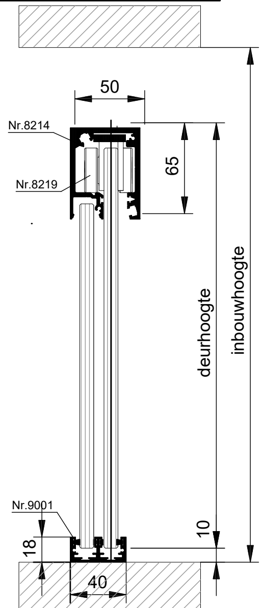
VERTICALE DOORSNEDE type DSD-11
