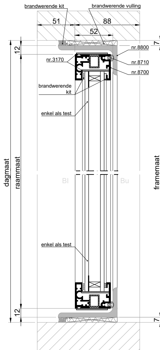
VERTICALE DOORSNEDE type AMD-12
