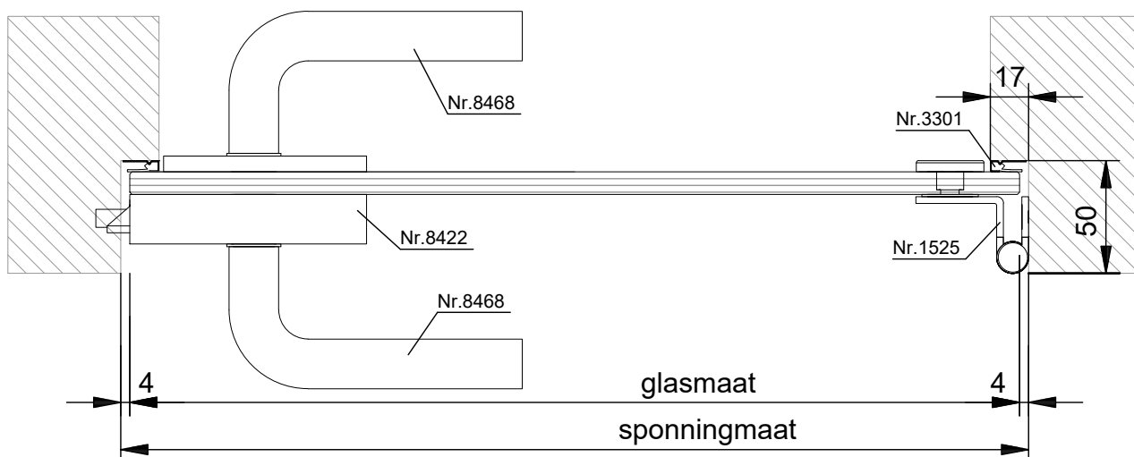
HORIZONTALE DOORSNEDE type TGD-1A
