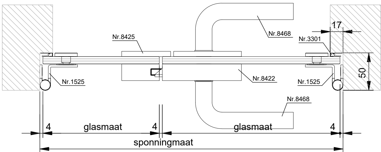
HORIZONTALE DOORSNEDE type TGD-14A
