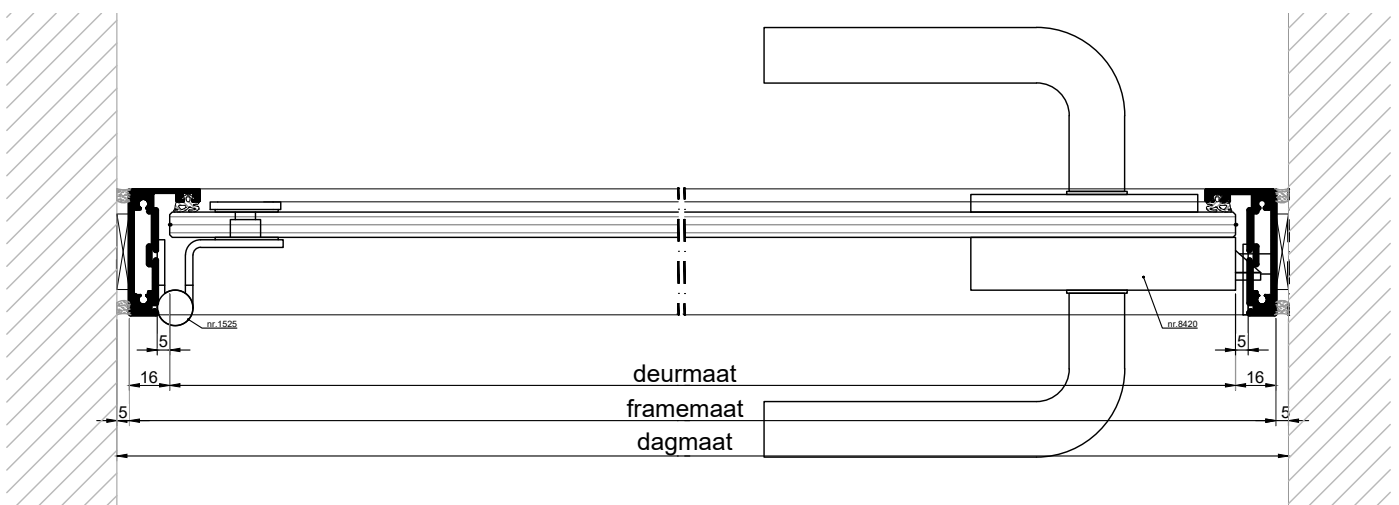
HORIZONTALE DOORSNEDE type TGDS-1B
