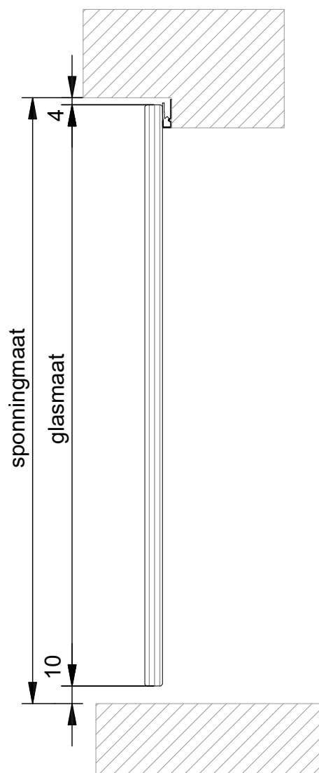
VERTICALE DOORSNEDE type TGD-1A
