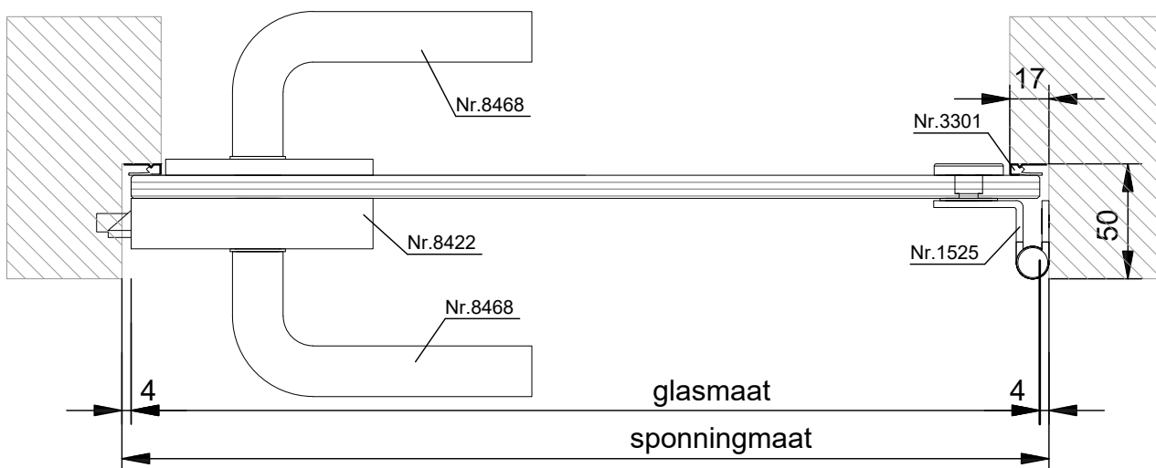
HORIZONTALE DOORSNEDE type TGD-1B
