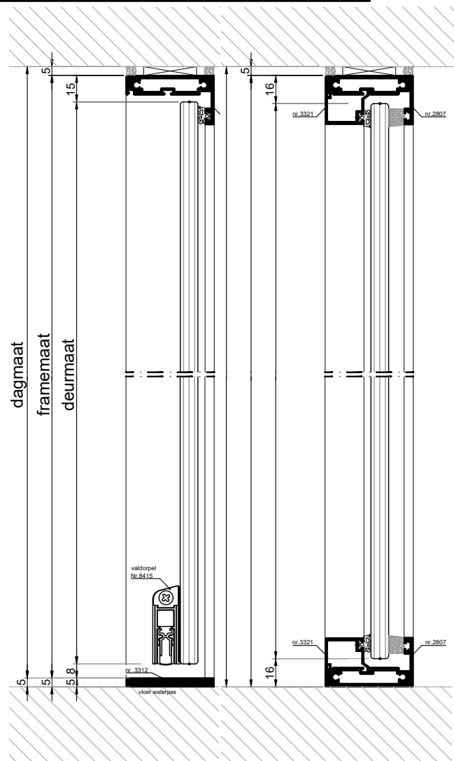
VERTICALE DOORSNEDE type TGDS-X
