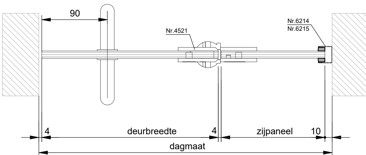
HORIZONTALE DOORSNEDE type TGZ-2
