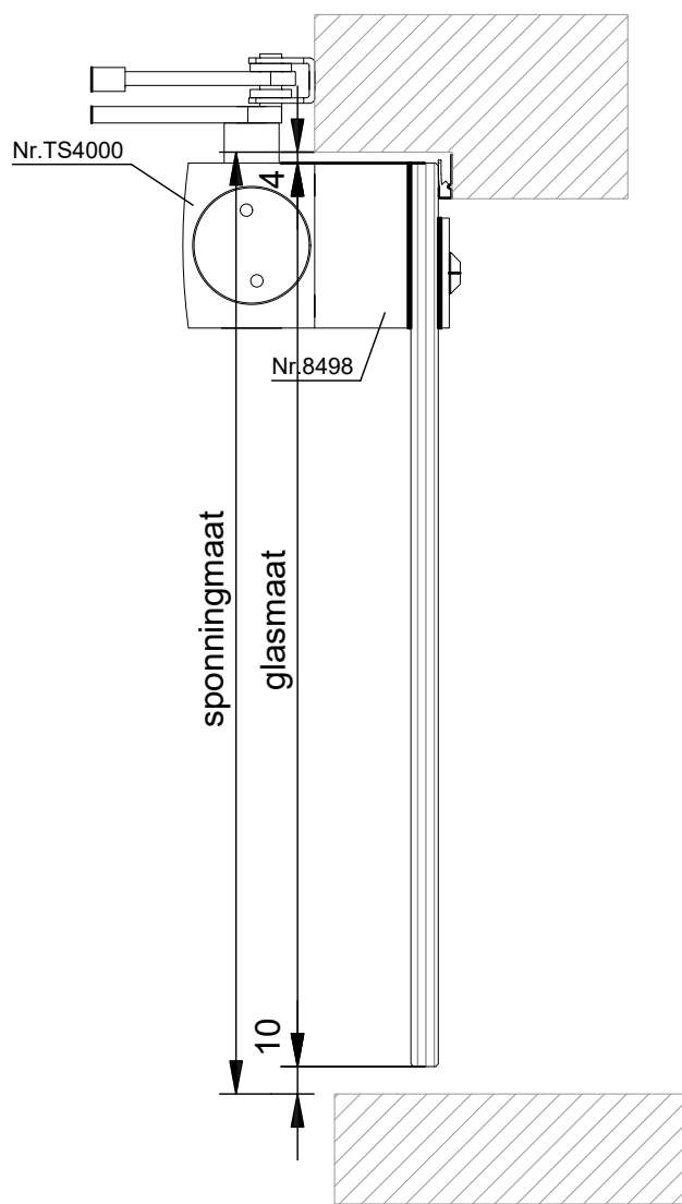
VERTICALE DOORSNEDE type TGD-1C
