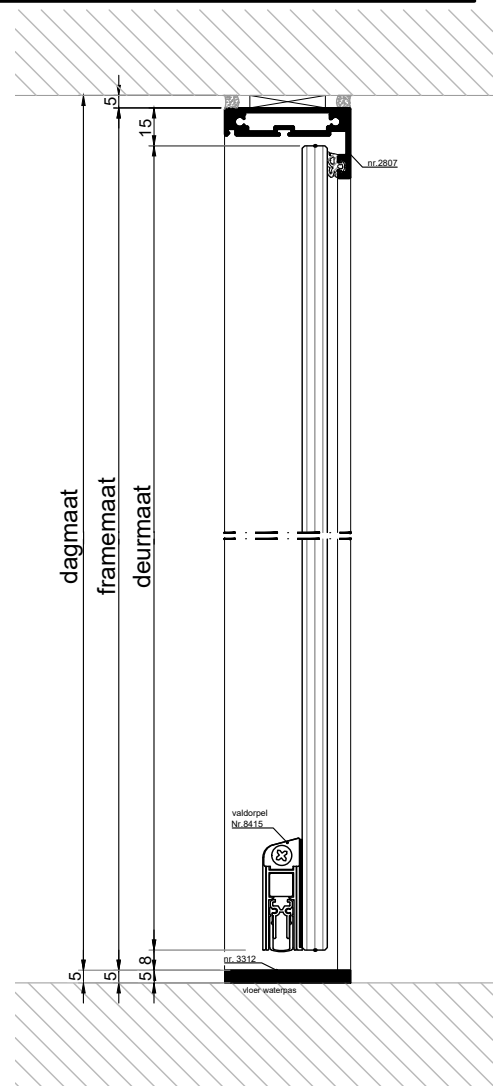
VERTICALE DOORSNEDE type TGDS-1B
