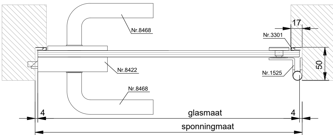
HORIZONTALE DOORSNEDE type TGD-1C
