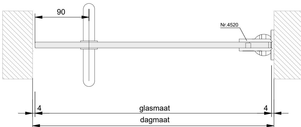
HORIZONTALE DOORSNEDE type TGZ-1
