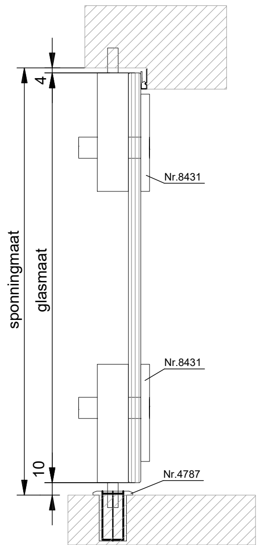
VERTICALE DOORSNEDE type TGD-14A
