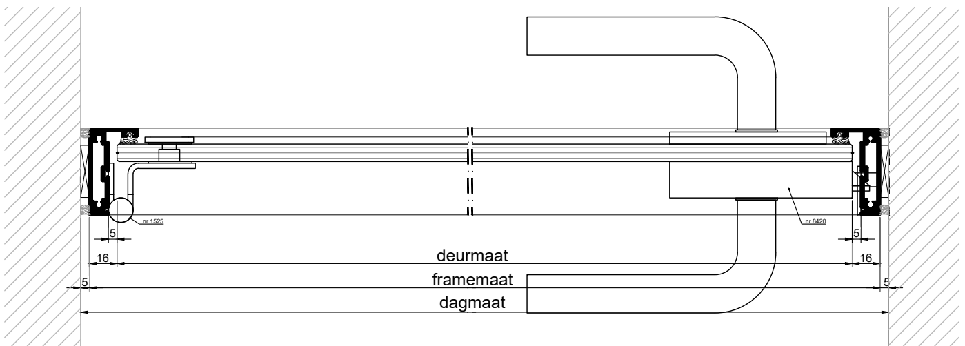
HORizontale Doorsnede type TGDS-1A
