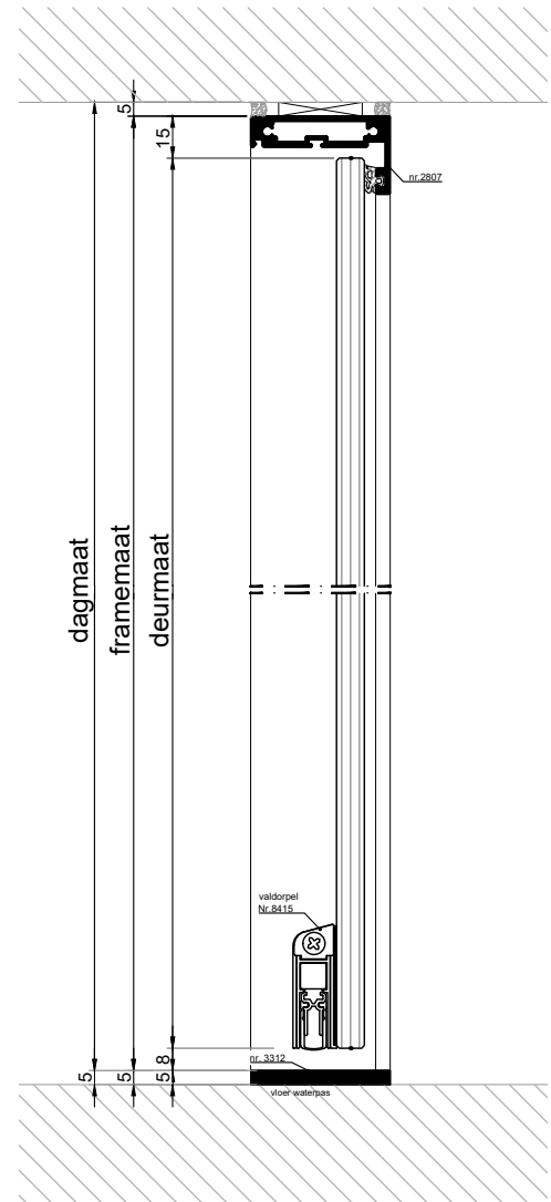
VERTICALE DOORSNEDE type TGDS-1A
