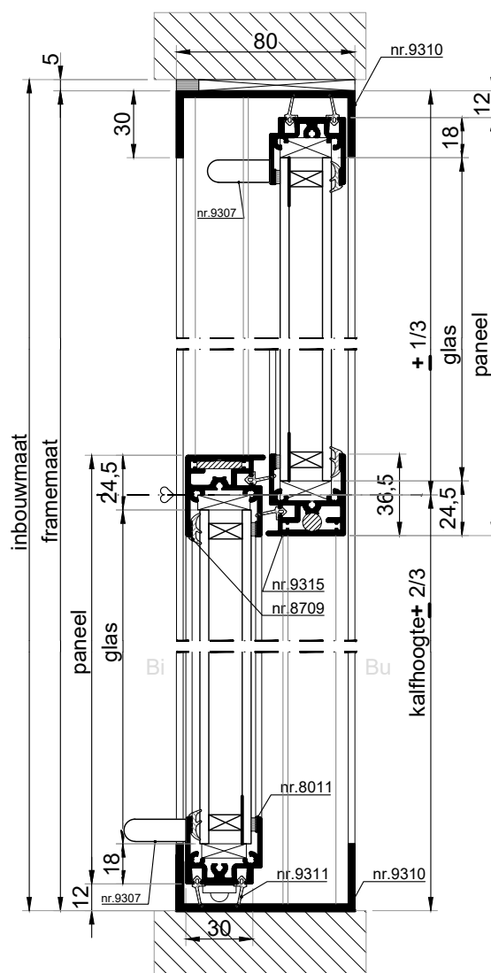
VERTECALE DOORSNEDE type VSV-30
