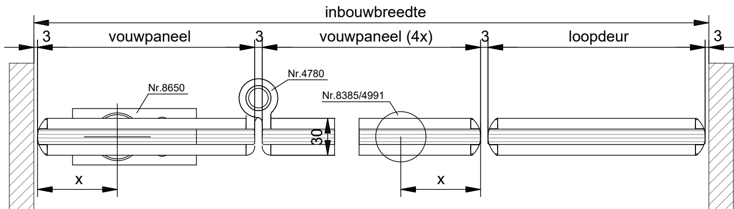
HORIZONTALE DOORSNEDE type TVD-5A
