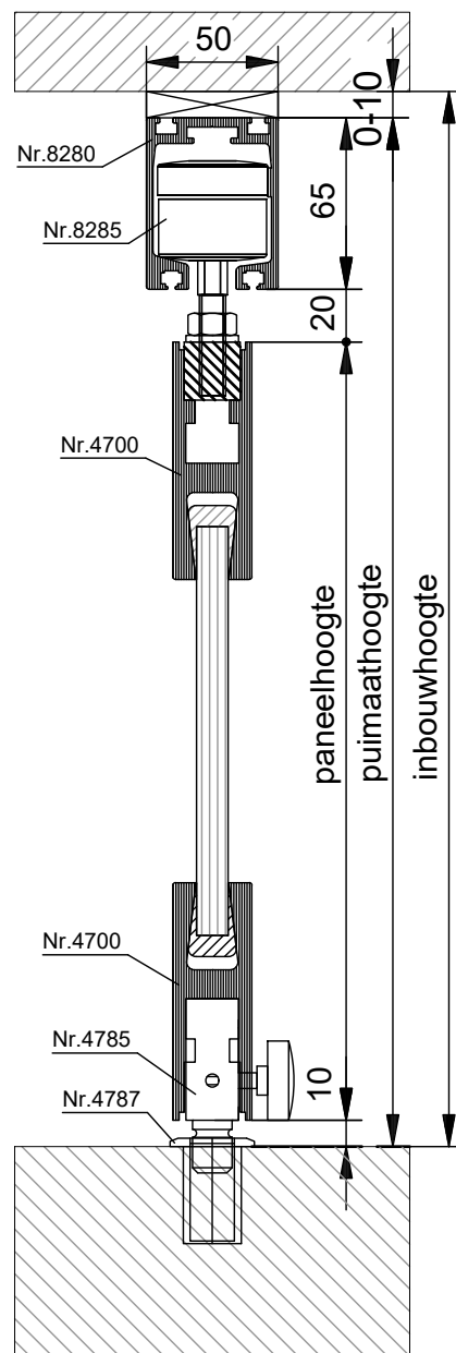
VERTICALE DOORSNEDE type THD-4A
