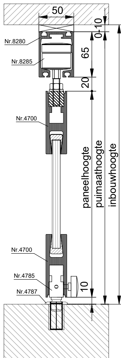
VERTICALE DOORSNEDE type THD-4B
