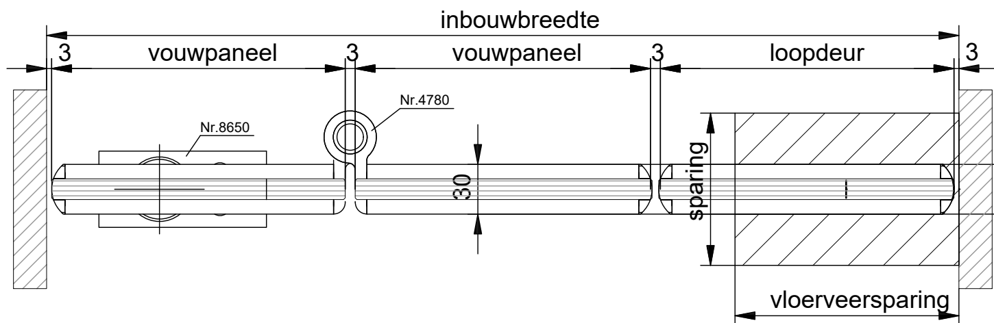
HORIZONTALE DOORSNEDE type TVD-3B vloerveer
