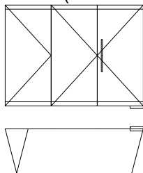
TVD-3B (zelfsluitend)
