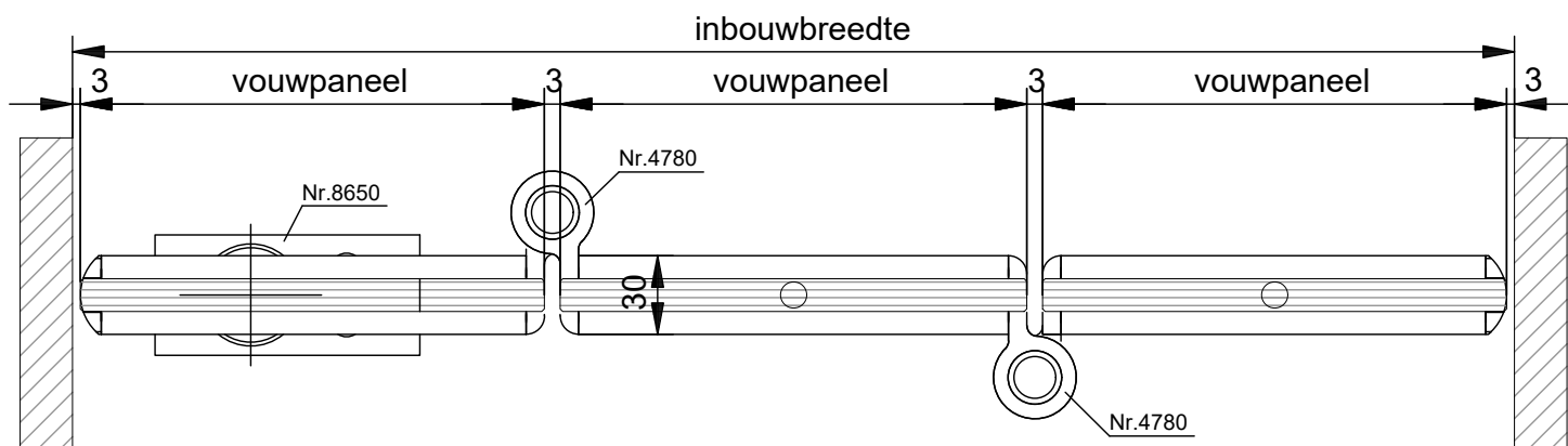
HORIZONTALE DOORSNEDE type THD-3A
