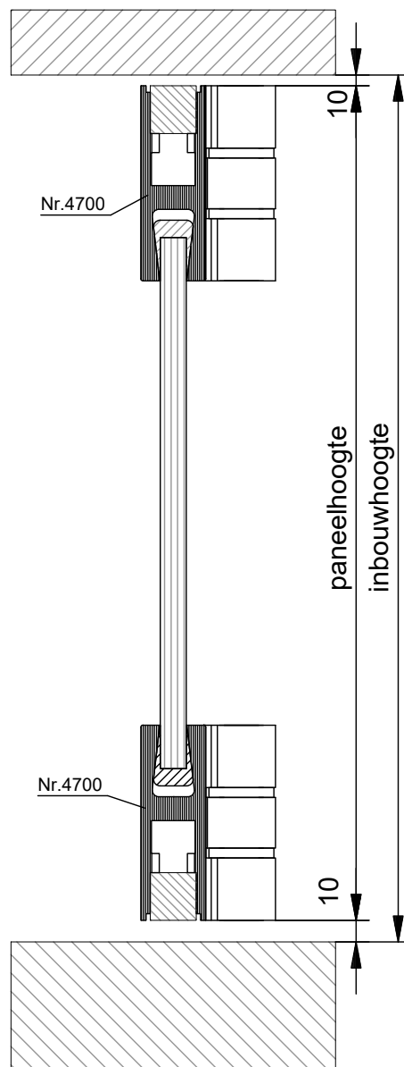
VERTICALE DOORSNEDE type TVD-2A
