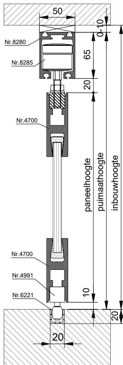
VERTICALE DOORSNEDE type TVD-6A
