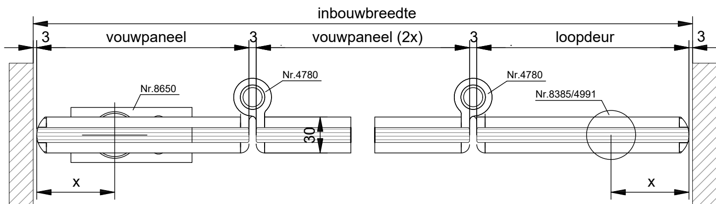
HORizontale DOORSNEDE type TVD-4A
