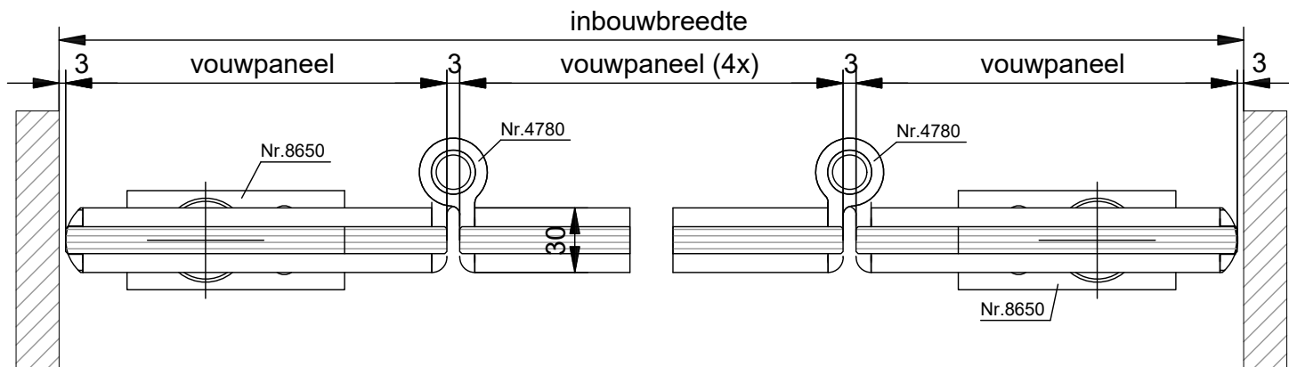
HORIZONTALE DOORSNEDE type TVD-6A
