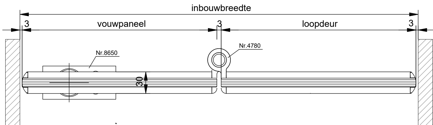
HORIZONTALE DOORSNEDE type TVD-2A
