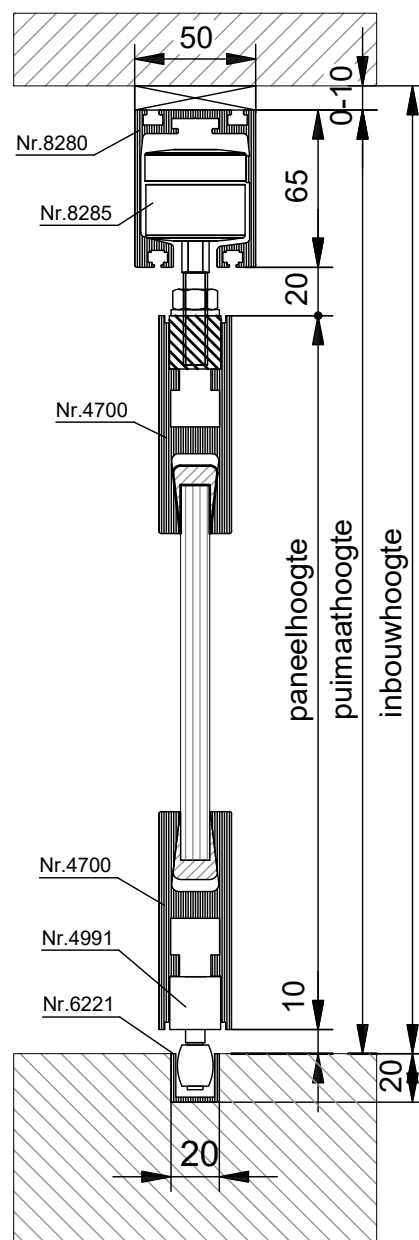
VERTICALE DOORSNEDE type TVD-4A
