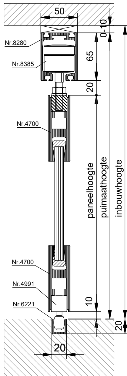
VERTICALE DOORSNEDE type TVD-3A
