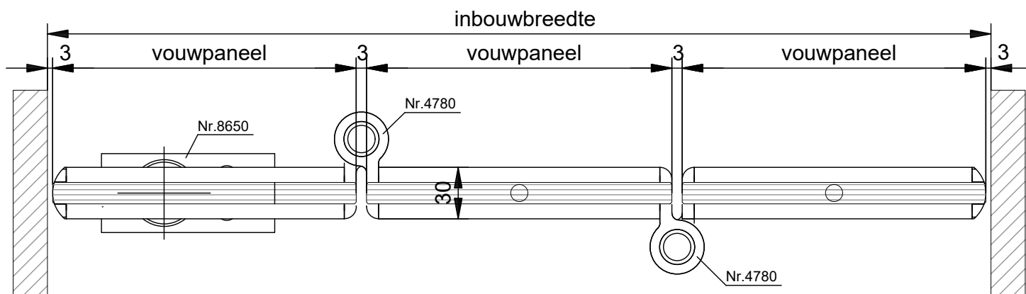
HORIZONTALE DOORSNEDE type THD-4A
