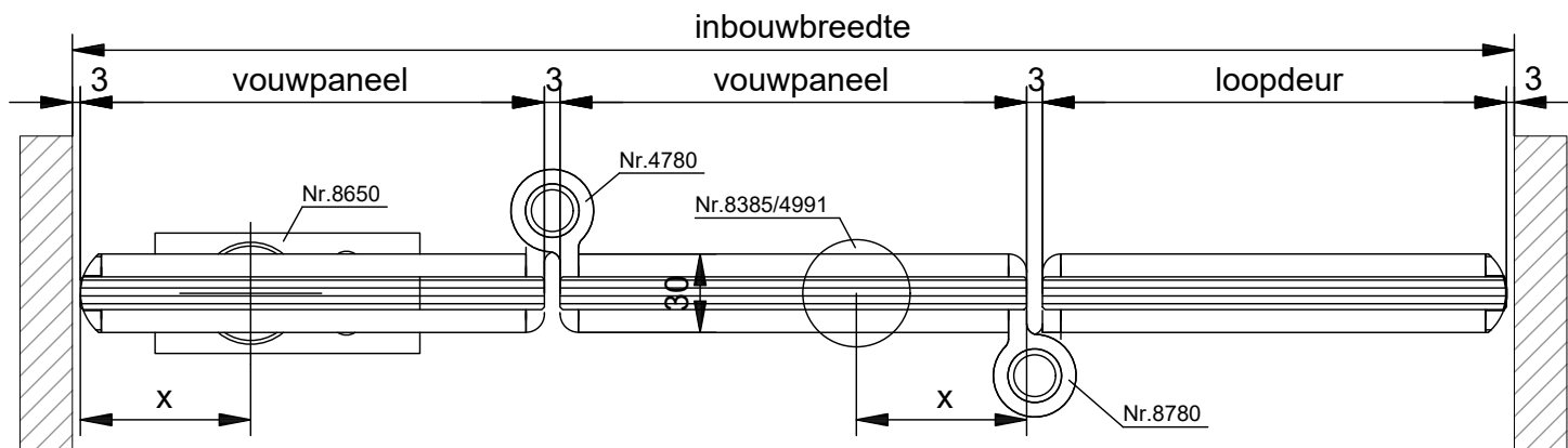
HORizontale DOORSNEDE type TVD-3A
