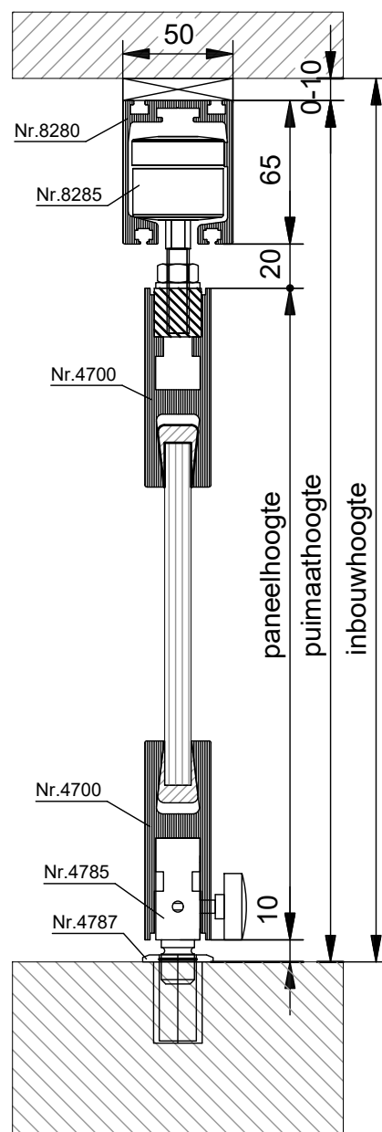
VERTICALE DOORSNEDE type THD-3A
