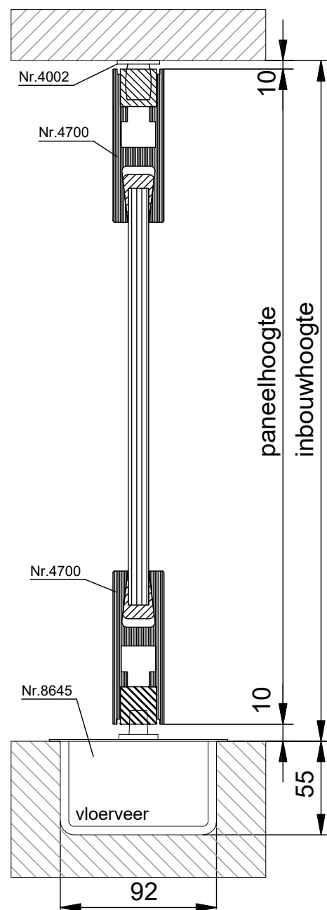
VERTICALE DOORSNEDE type TVD-3B vloerveer
