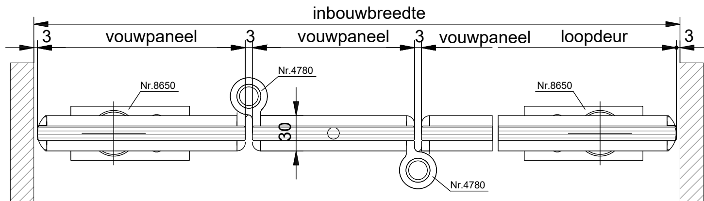
HORIZONTALE DOORSNEDE type THD-4B
