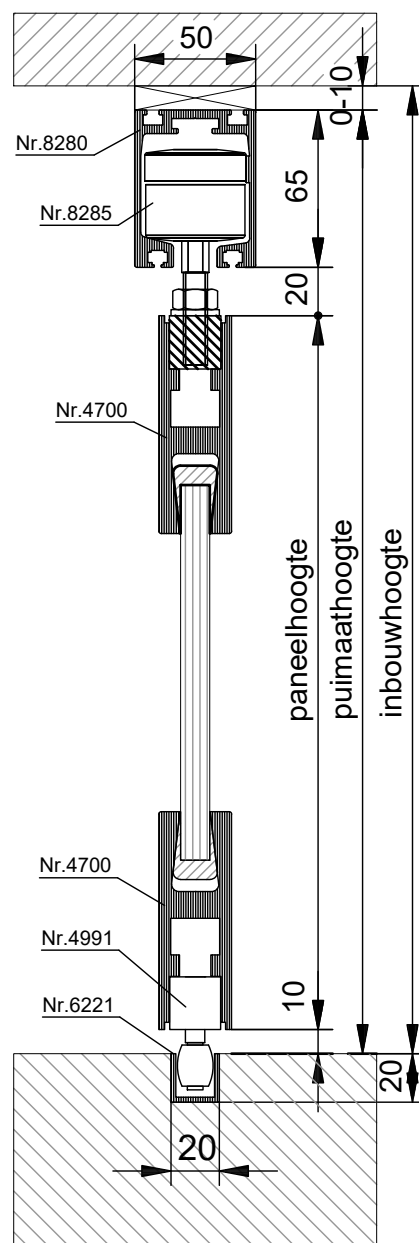
VERTICALE DOORSNEDE type TVD-5A
