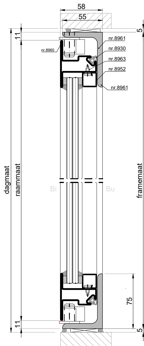
VERTECALE DOORSNEDE type MAS-3
