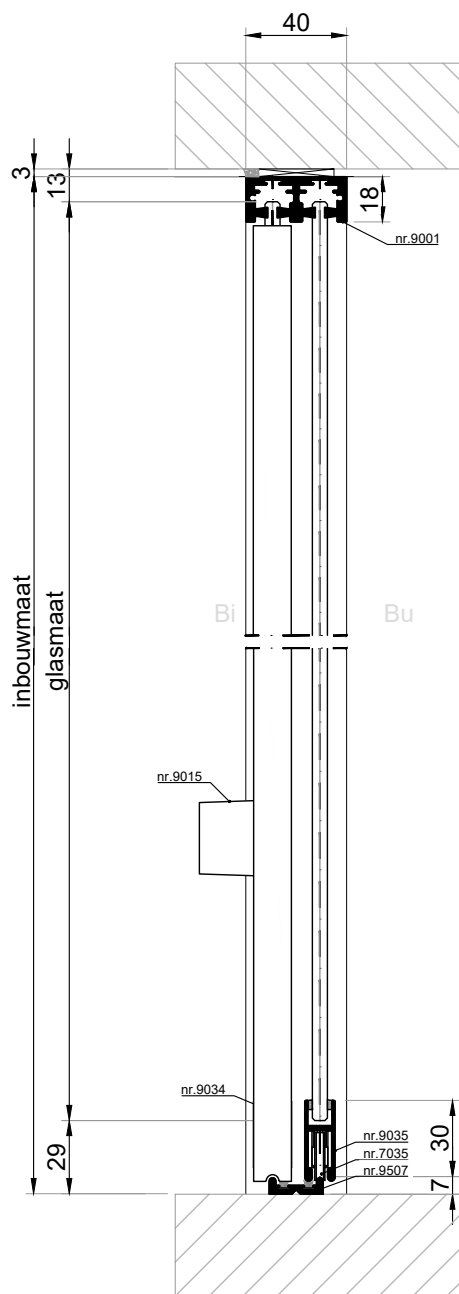
VERTICALE DOORSNEDE type HSV-2
