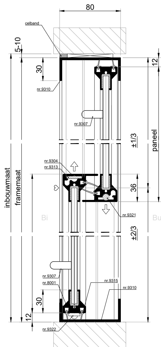
VERTECALE DOORSNEDE type VSV-3
