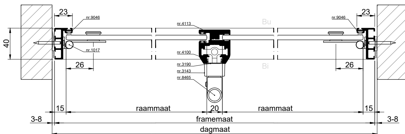
HORIZONTALE DOORSNEDE type SVR-7
