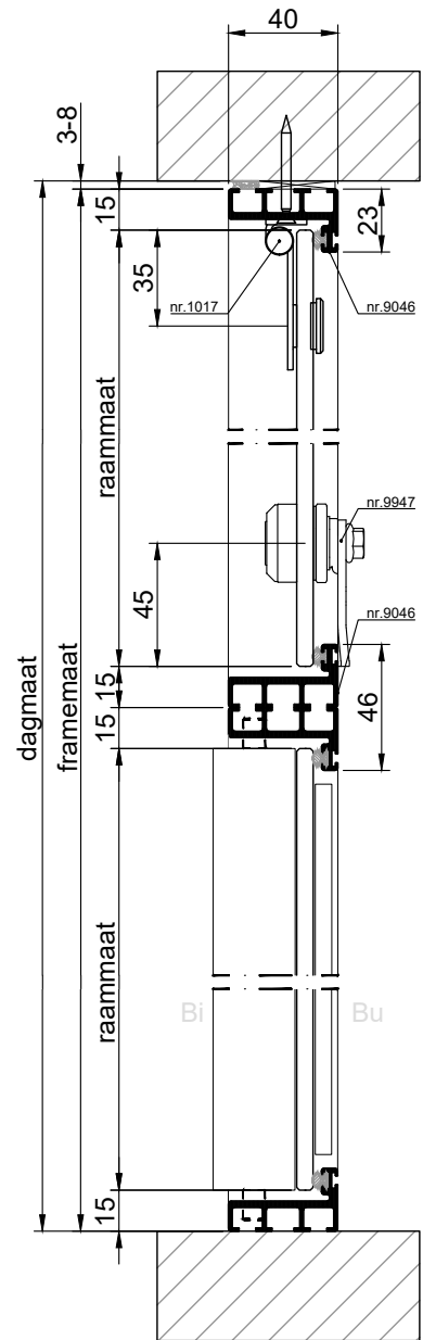
VERTICALE DOORSNEDE type SVC-10
