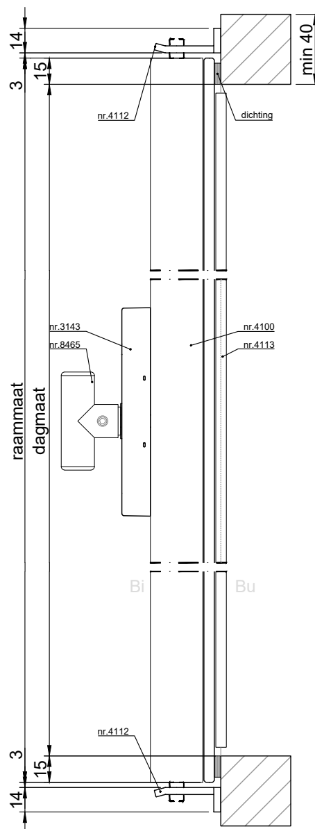
VERTICALE DOORSNEDE type SVR-5
