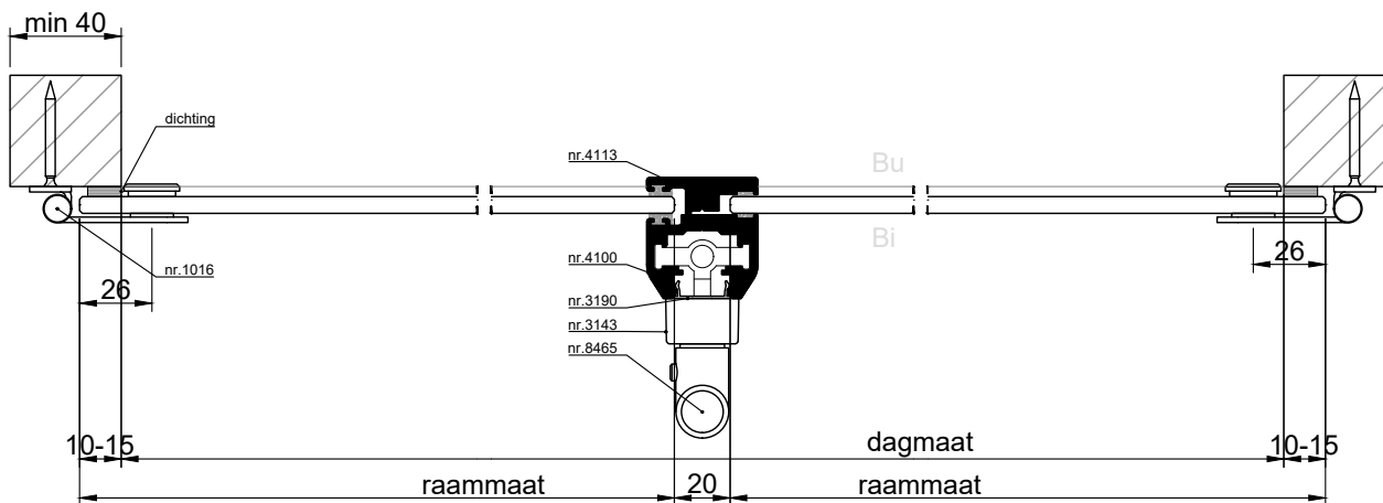
HORIZONTALE DOORSNEDE type SVR-5
