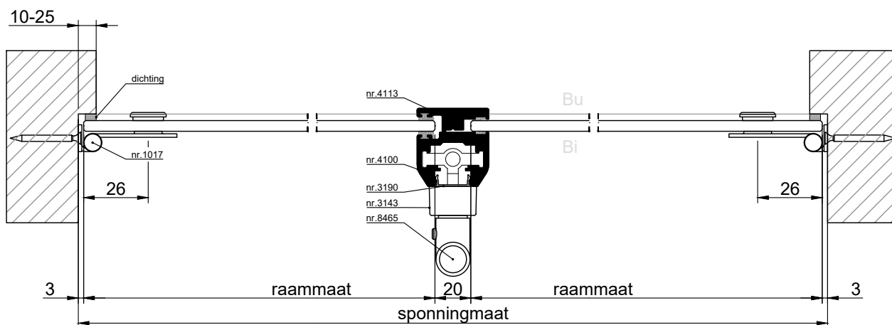
HORIZONTALE DOORSNEDE type SVR-6
