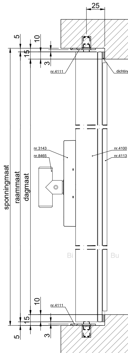
VERTICALE DOORSNEDE type SVR-6
