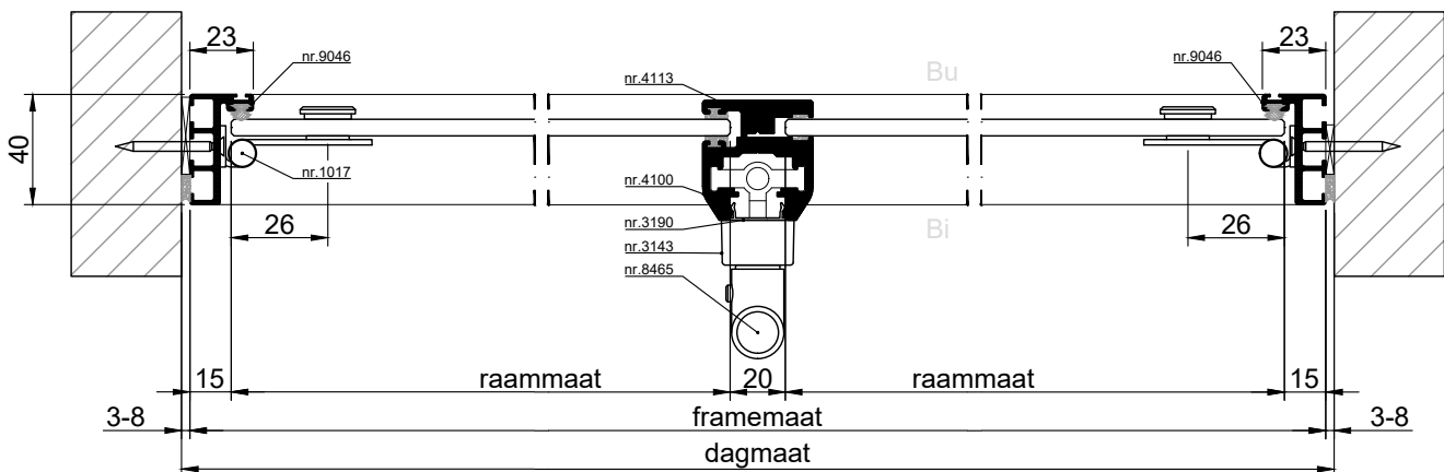
HORizontale Doorsnede type SVC-10
