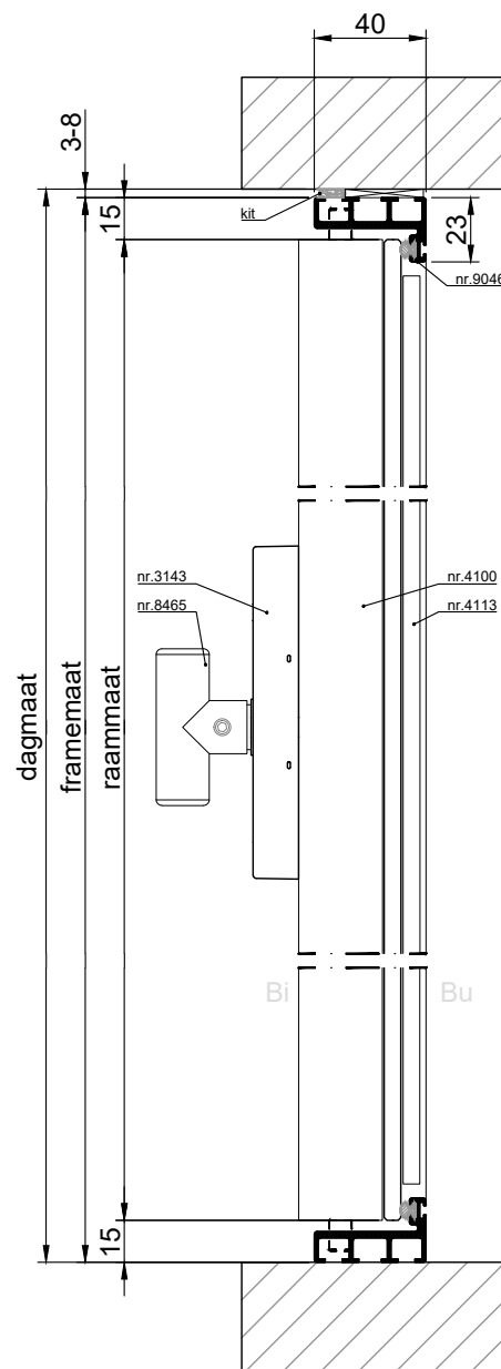
VERTICALE DOORSNEDE type SVR-7
