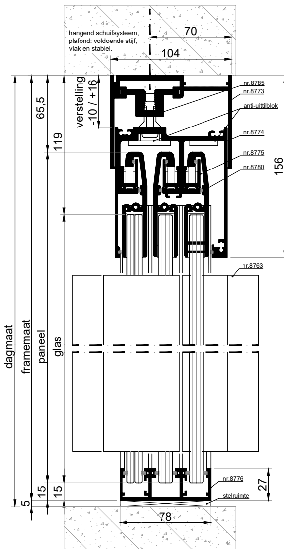
VERTICALE DOORSNEDE type BSH-33A
