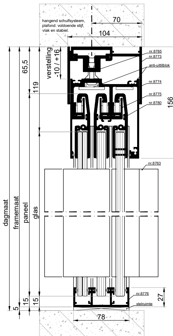
VERTICALE DOORSNEDE type BSH-35A
