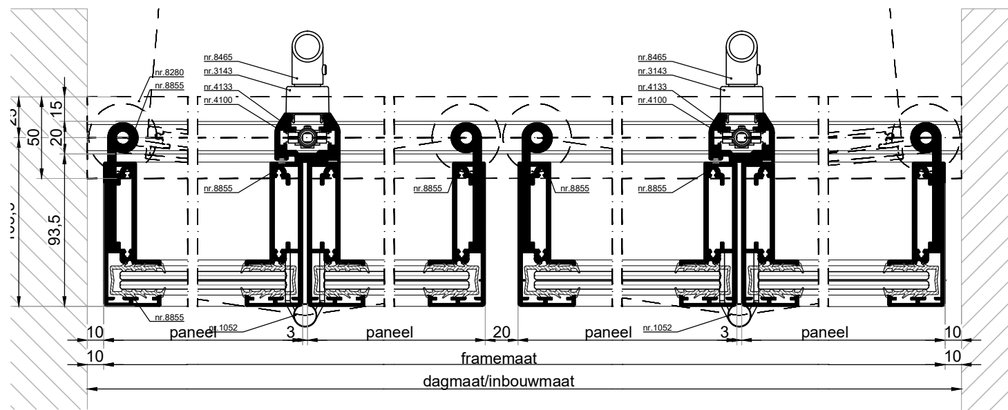
HORizontale DOORSNEDE type BSV-4
