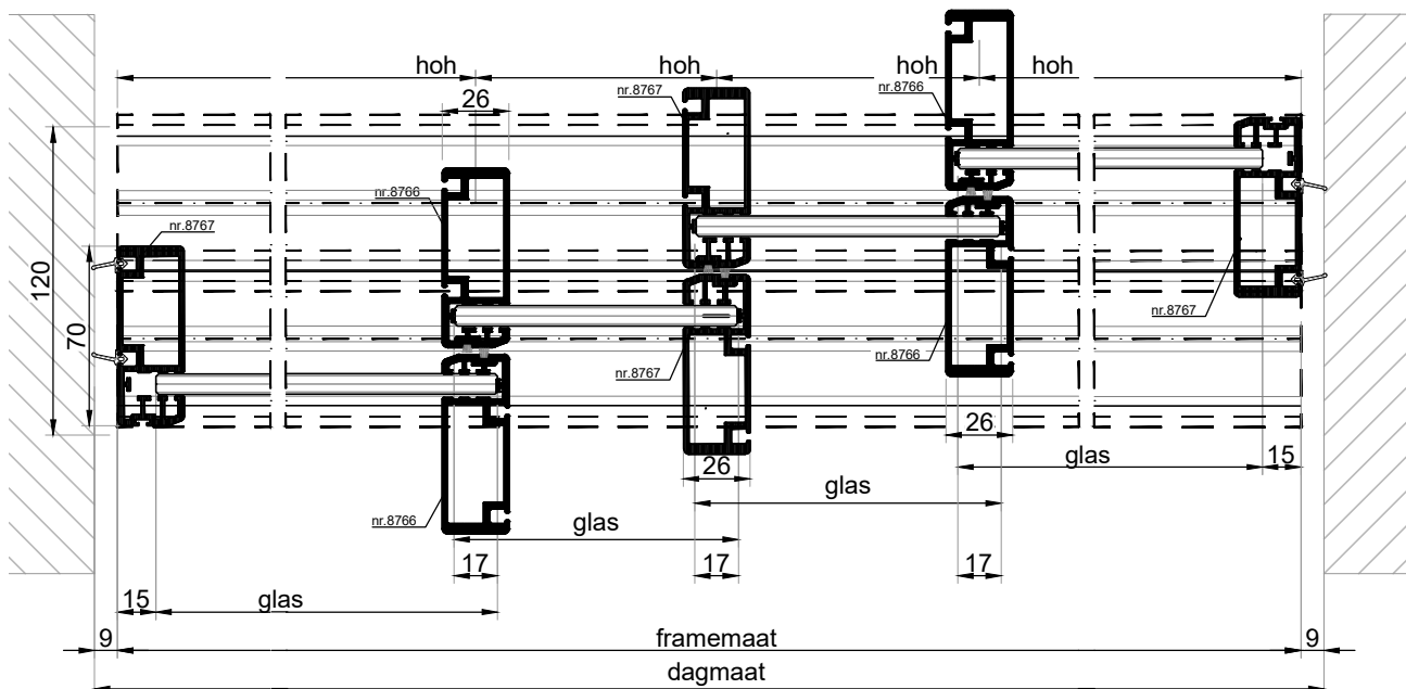
HORIZONTALE DOORSNEDE type BSH-44A
