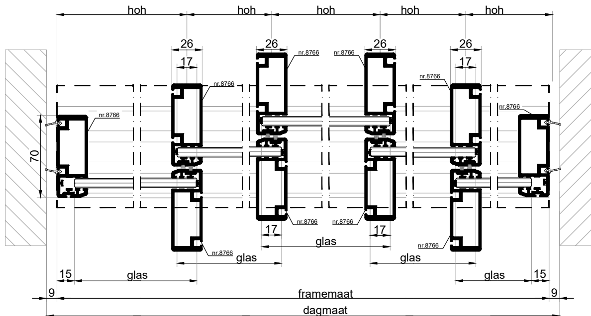
HORIZONTALE DOORSNEDE type BSH-35A
