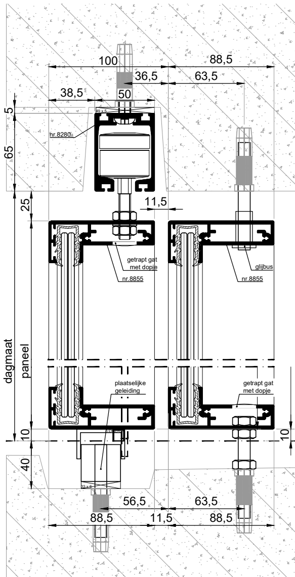
VERTICALE DOORSNEDE type BSH-10E
