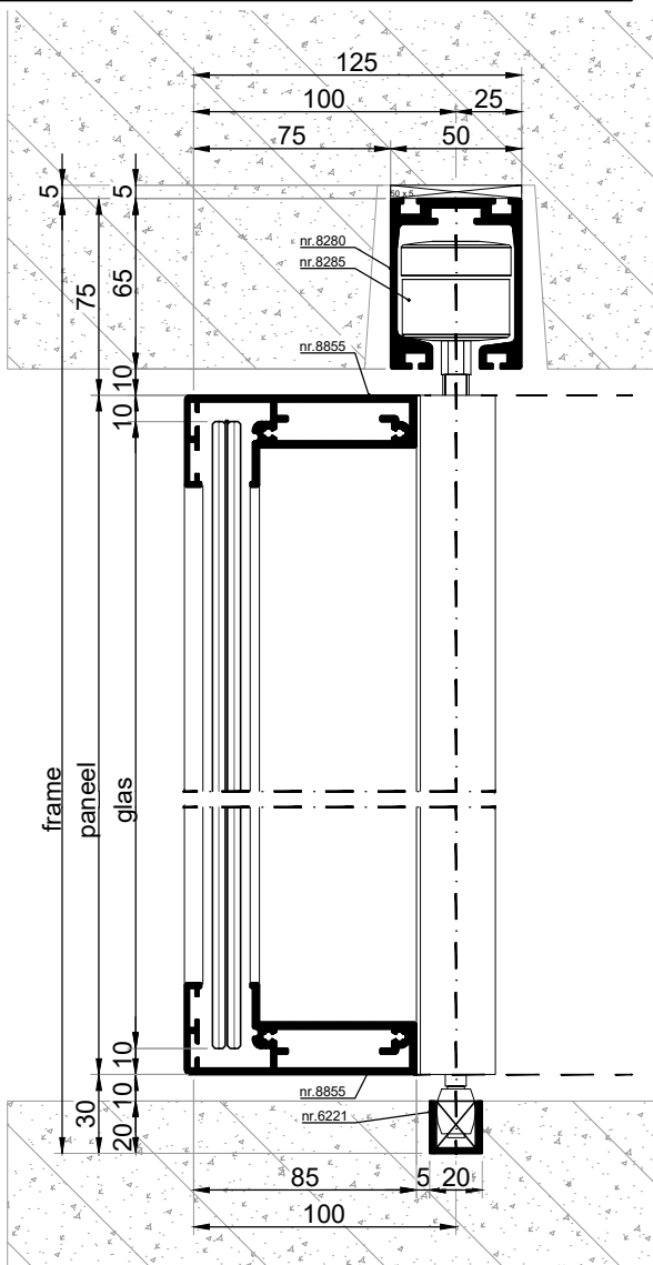
VERTICALE DOORSNEDE type BSV-2
