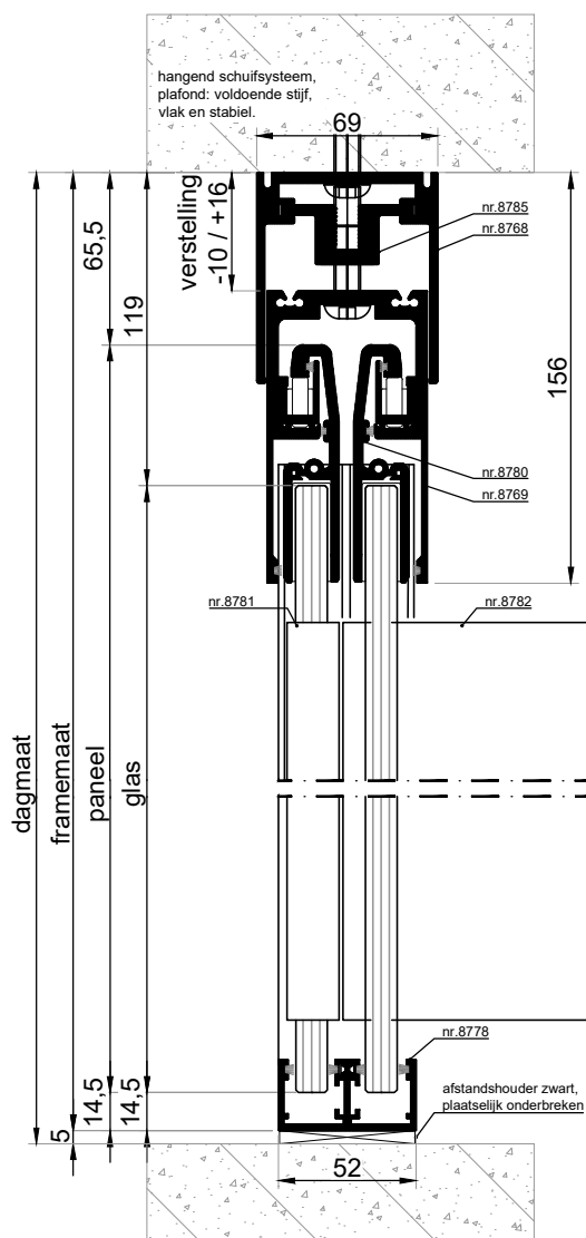
VERTICALE DOORSNEDE type BSH-22B
