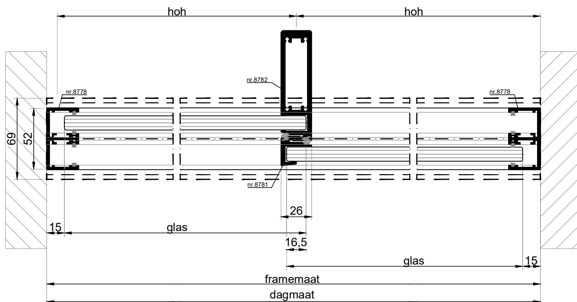
HORIZONTALE DOORSNEDE type BSH-22B
