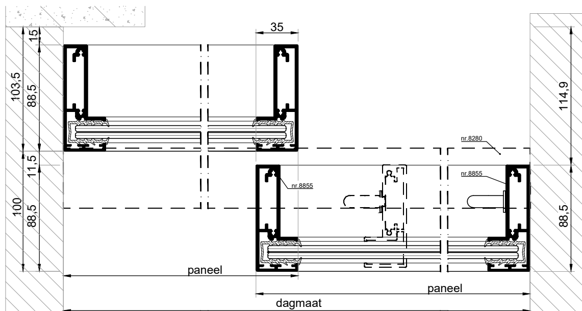
HORIZONTALE DOORSNEDE type BSH-10A
