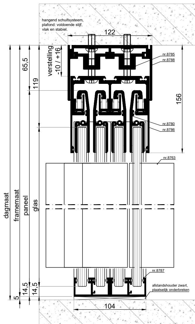
VERTICALE DOORSNEDE type BSH-44A
