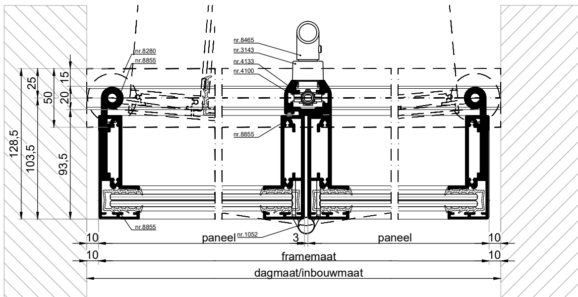
HORIZONTALE DOORSNEDE type BSV-2
