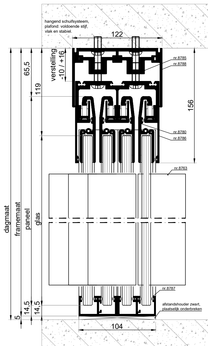
VERTICALE DOORSNEDE type BSH-45A
