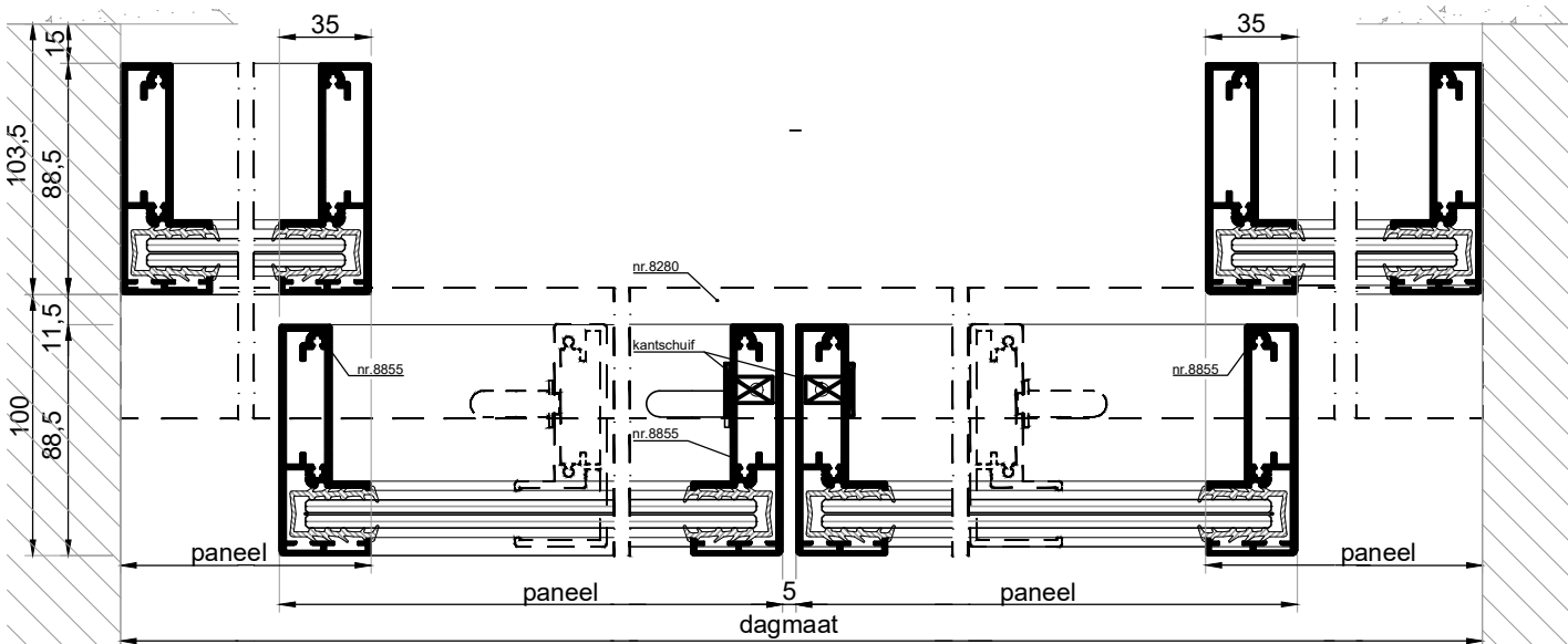
HORizontale Doorsnede type BSH-10E
