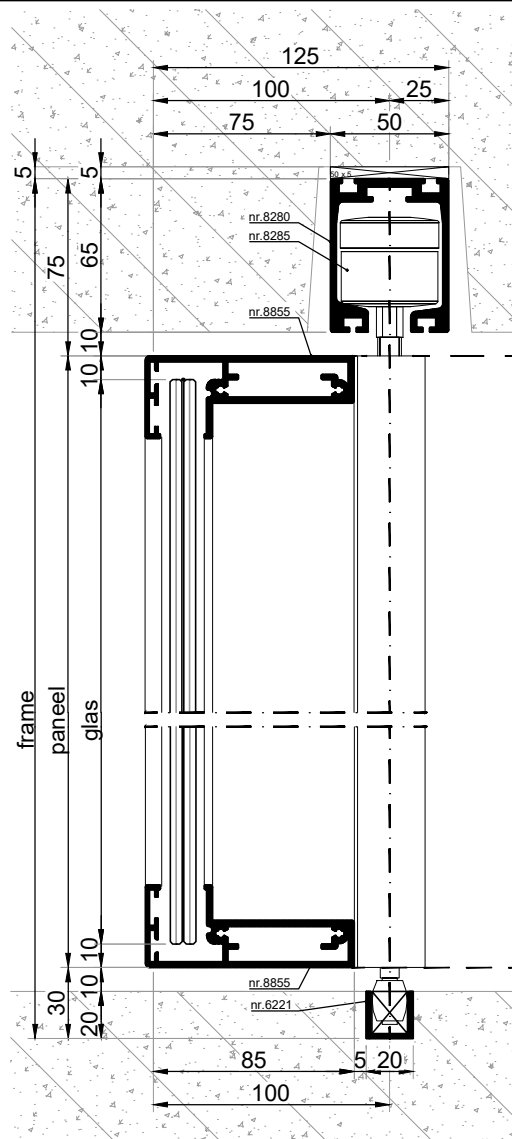
VERTICALE DOORSNEDE type BSV-4
