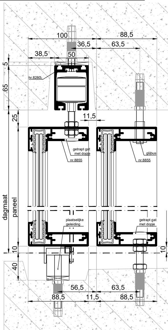
VERTICALE DOORSNEDE type BSH-10A
