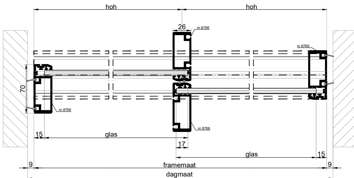
HORizontale DOORSNEDE type BSH-22A
