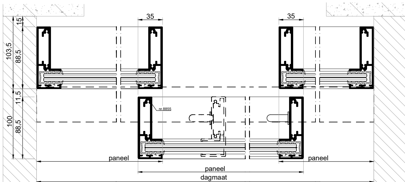
HORIZONTALE DOORSNEDE type BSH-10C
