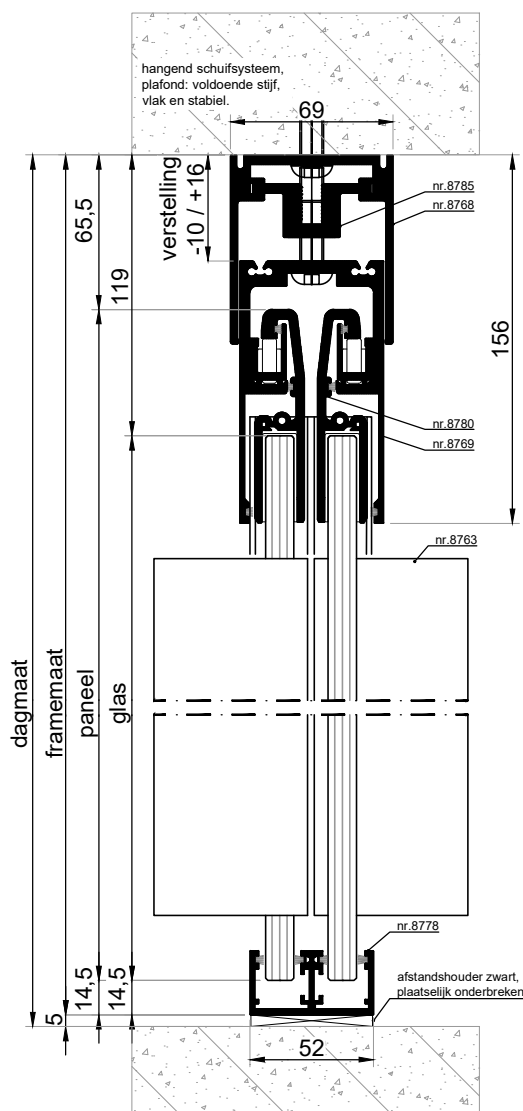
VERTICALE DOORSNEDE type BSH-22A
