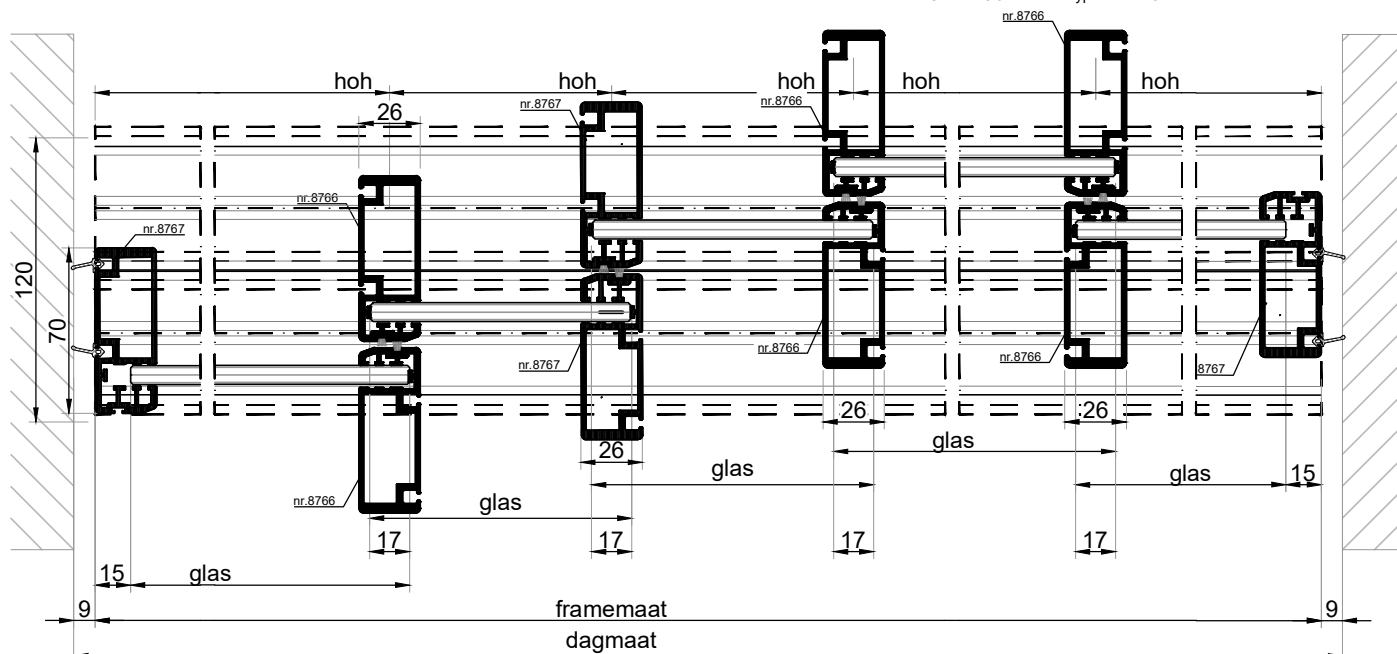
HORizontale DOORSNEDE type BSH-45A
