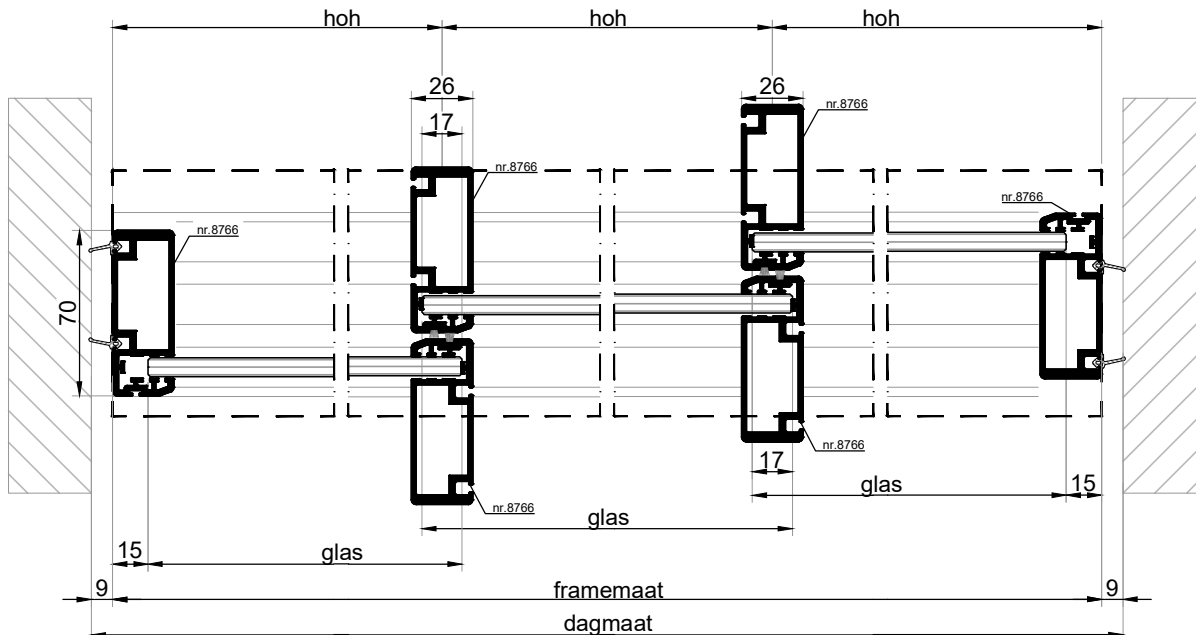
HORIZONTALE DOORSNEDE type BSH-33A
