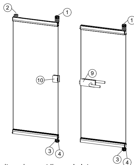
uitvoering met liggend slot
