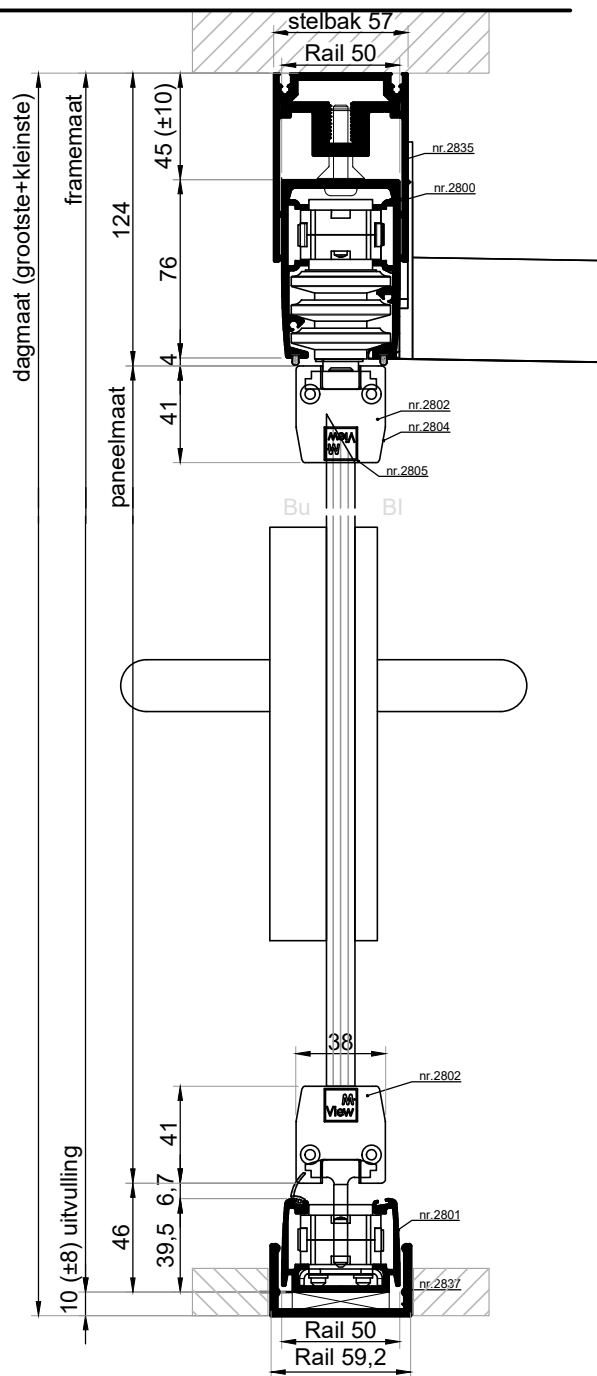
VERTICALE DOORSNEDE type MBG-2C
