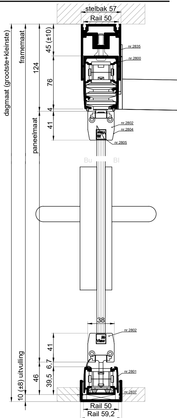
VERTECALE DOORSNEDE type MBU-2C
