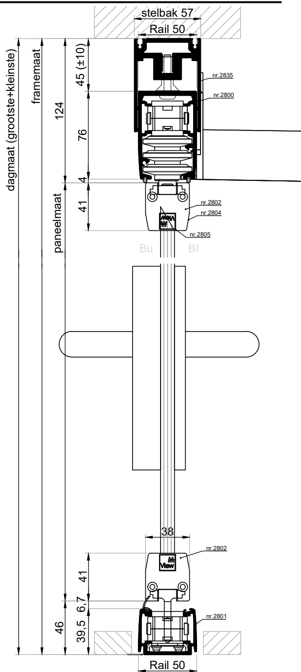
VERTICALE DOORSNEDE type MBR-1C
