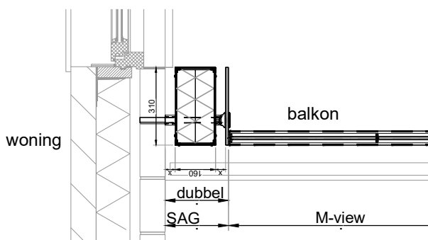
Type Box-10B-40x310 aan zijkant
