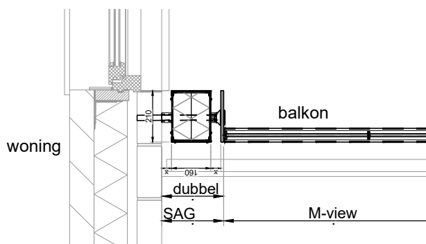
Type Box-10B-40x210 aan zijkant
