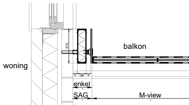
Type Box-10A-40x310 aan zijkant
