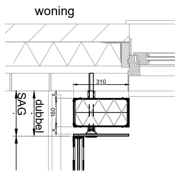
Type Box-10B-40x310 aan bovenzijde
