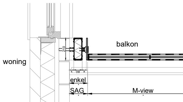
Type Box-10A-40x210 aan zijkant
