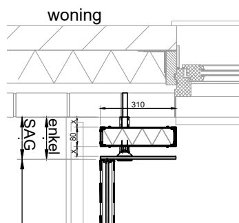
Type Box-10A-40x310 aan bovenzijde
