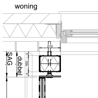
Type Box-10B-40x210 aan bovenzijde
