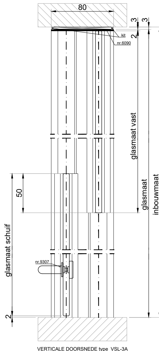
VERTICALE DOORSNEDE type VSL-3A
