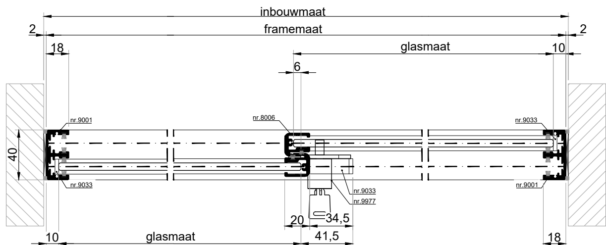
HORIZONTALE DOORSNEDE type HSL-4A
