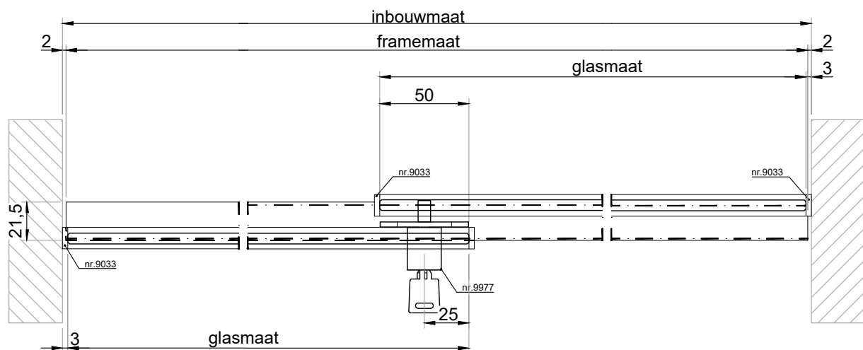
HORIZONTALE DOORSNEDE type HSL-5A
