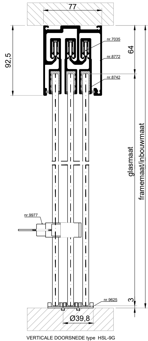
VERTICALE DOORSNEDE type HSL-9G
