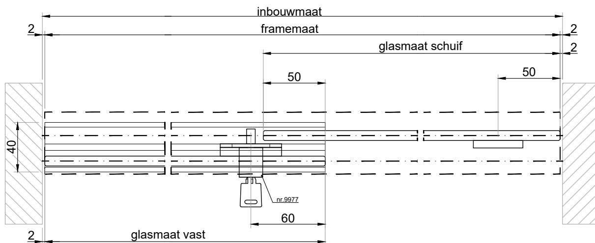
HORIZONTALE DOORSNEDE type HSL-10B
