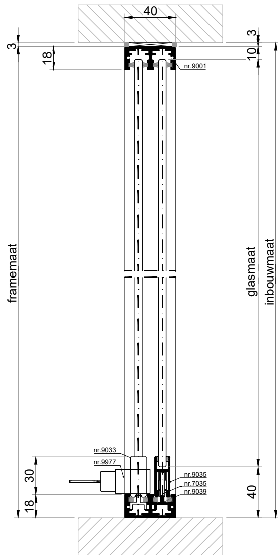
VERTECALE DOORSNEDE type HSL-4A
