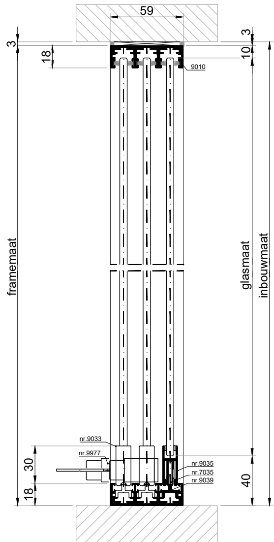
VERTICALE DOORSNEDE type HSL-2G
