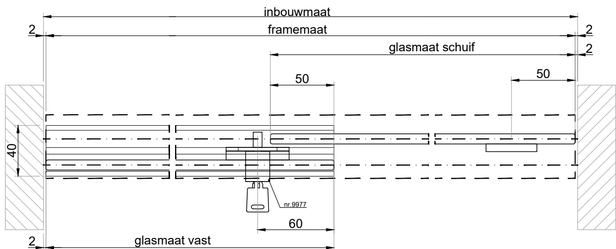
HORIZONTALE DOORSNEDE type HSL-10B
