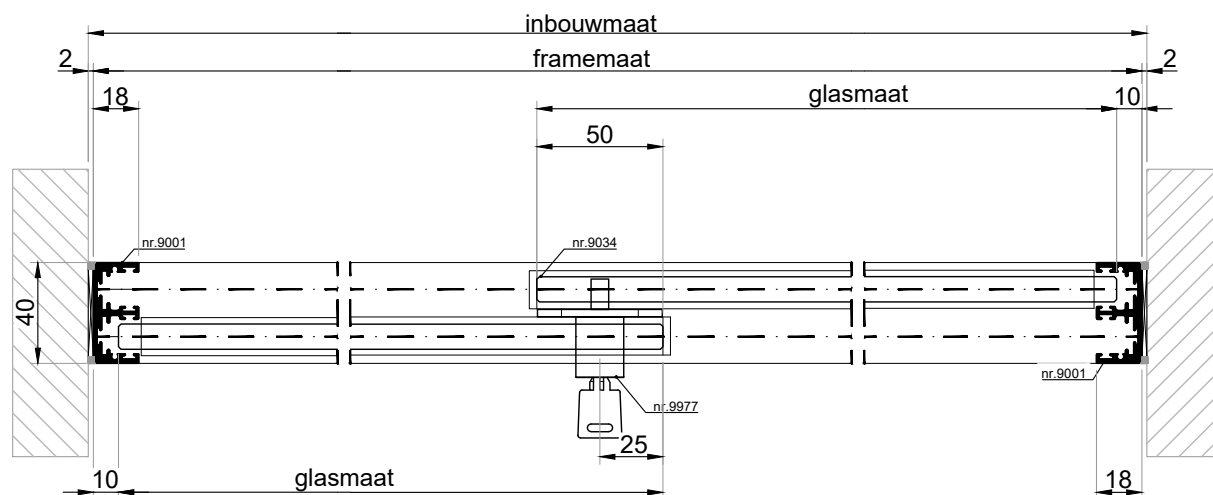
HORIZONTALE DOORSNEDE type HSL-3A
