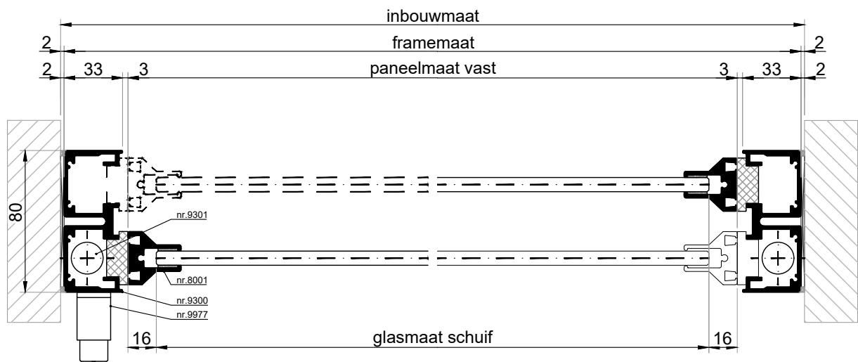
HORIZONTALE DOORSNEDE type VSL-4A
