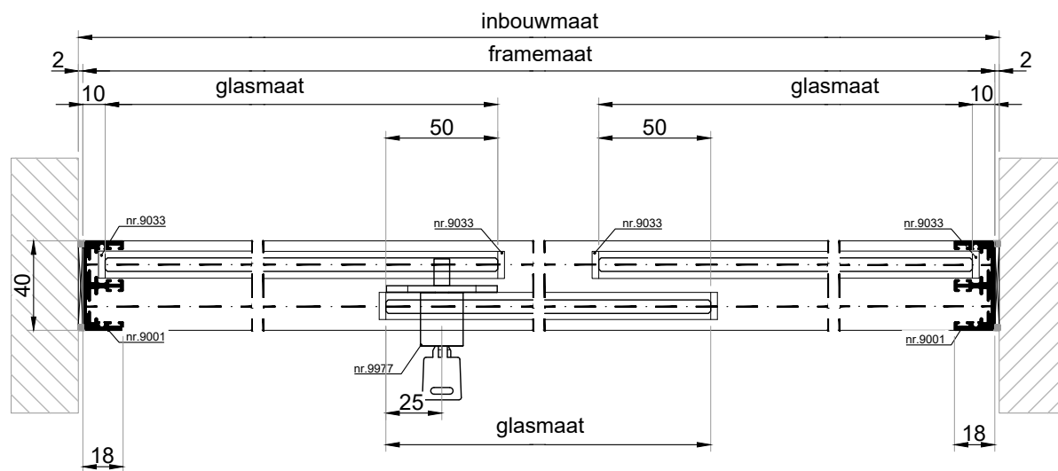
HORIZONTALE DOORSNEDE type HSL-2D
