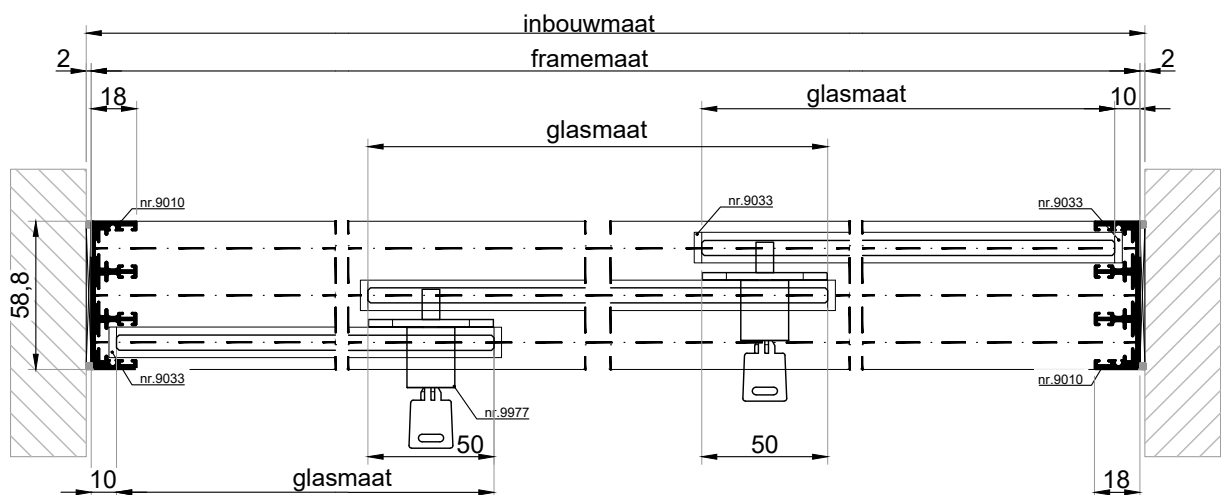
HORizontale Doorsnede type HSL-2G
