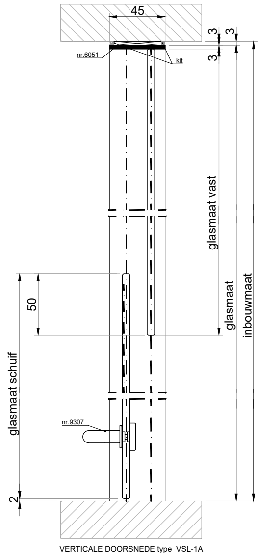
VERTICALE DOORSNEDE type VSL-1A
