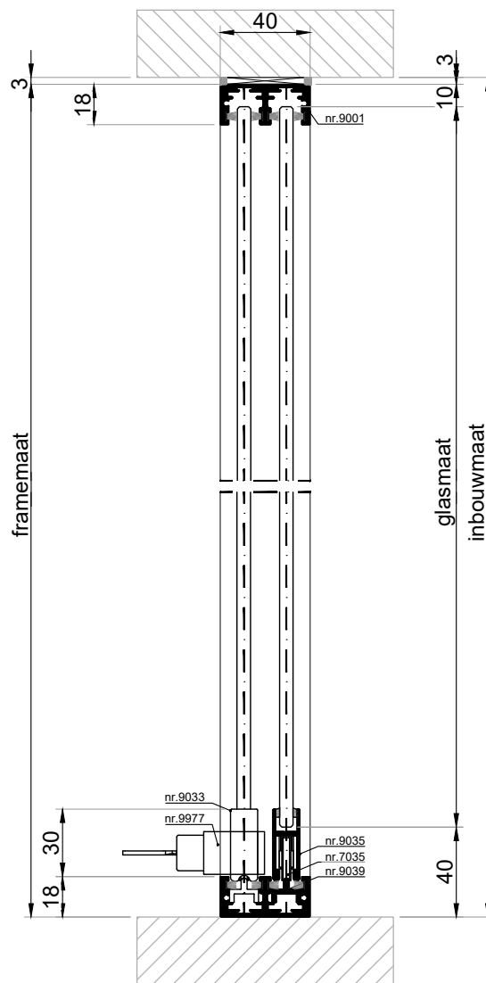
VERTECALE DOORSNEDE type HSL-4A
