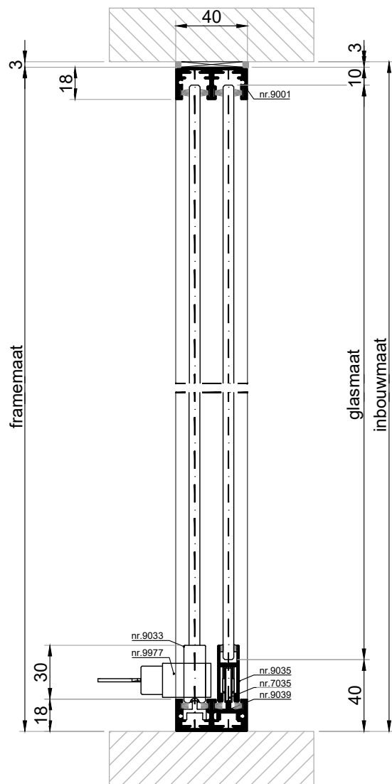
VERTECALE DOORSNEDE type HSL-4E
