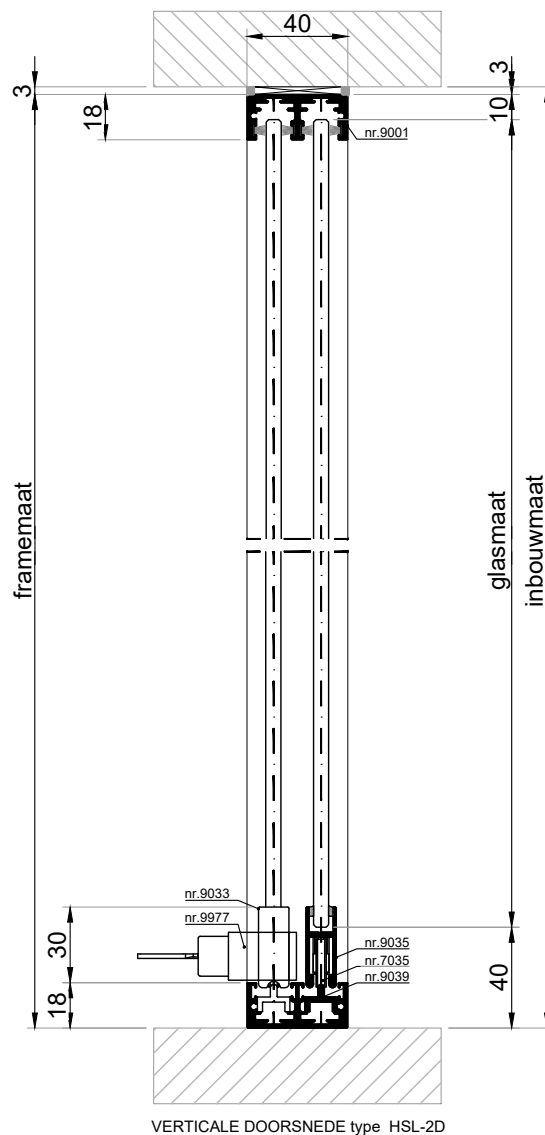
VERTICALE DOORSNEDE type HSL-2D
