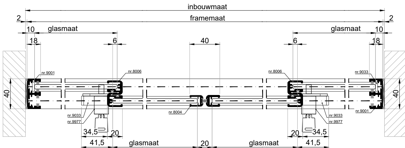
HORIZONTALE DOORSNEDE type HSL-4E
