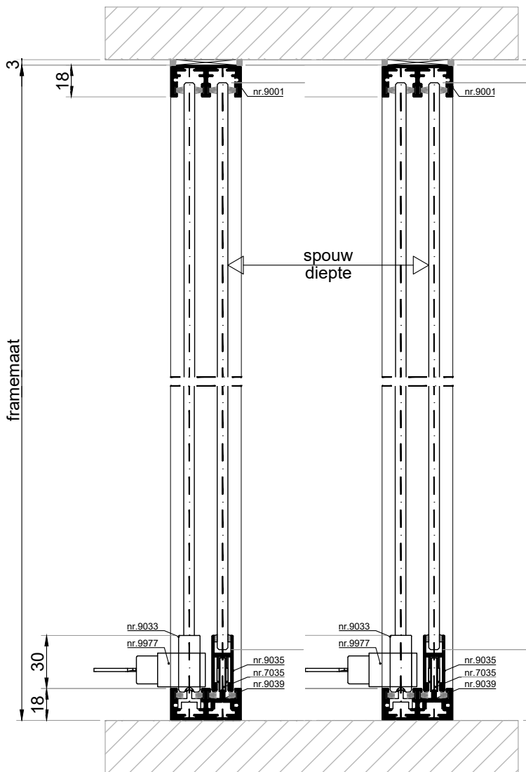
VERTICALE DOORSNEDE type HSL-4AD
