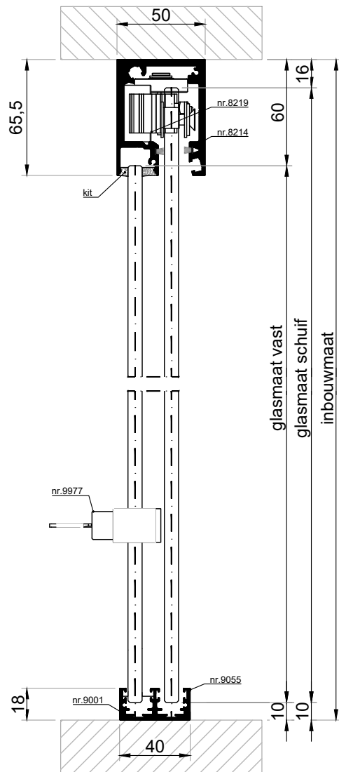
VERTICALE DOORSNEDE type HSL-10B
