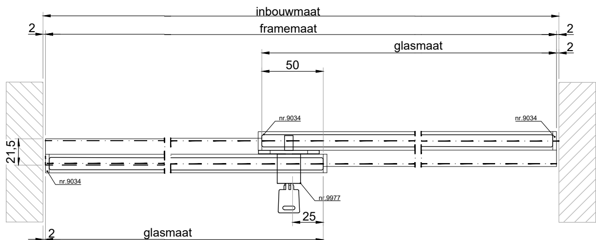
HORIZONTALE DOORSNEDE type HSL-6A
