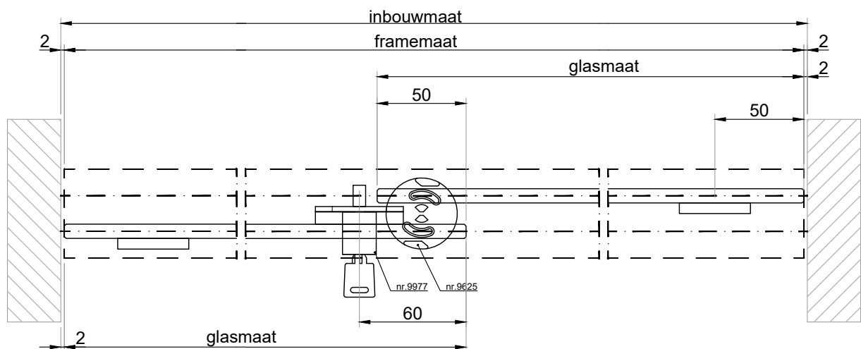
HORIZONTALE DOORSNEDE type HSL-9A
