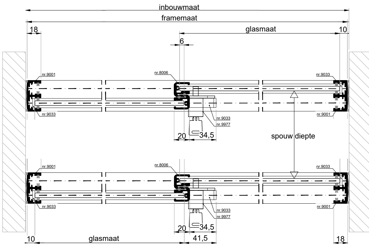
HORIZONTALE DOORSNEDE type HSL-4AD
