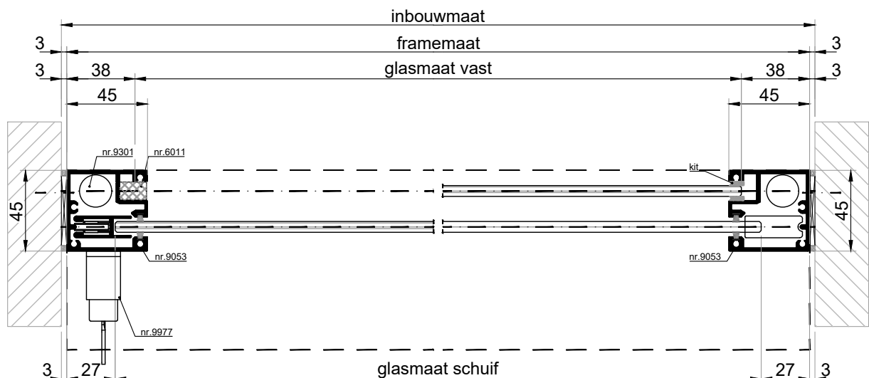
HORIZONTALE DOORSNEDE type VSL-1A
