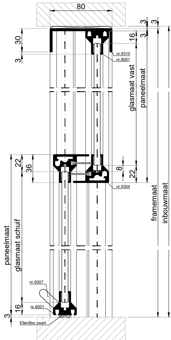
VERTICALE DOORSNEDE type VSL-4A
