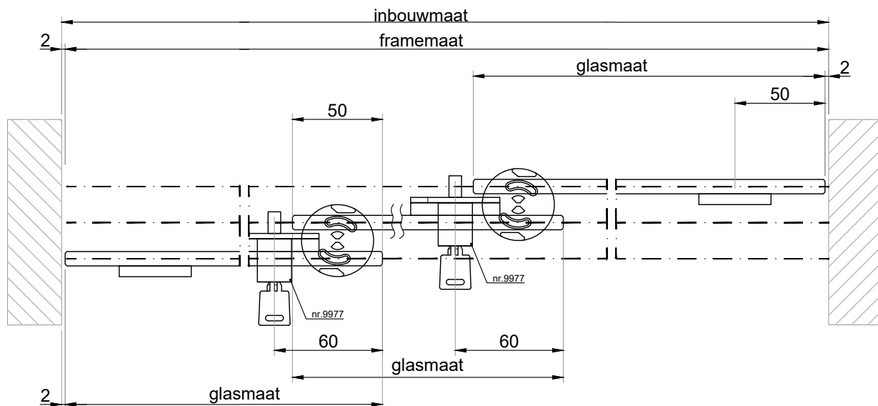
HORIZONTALE DOORSNEDE type HSL-9G
