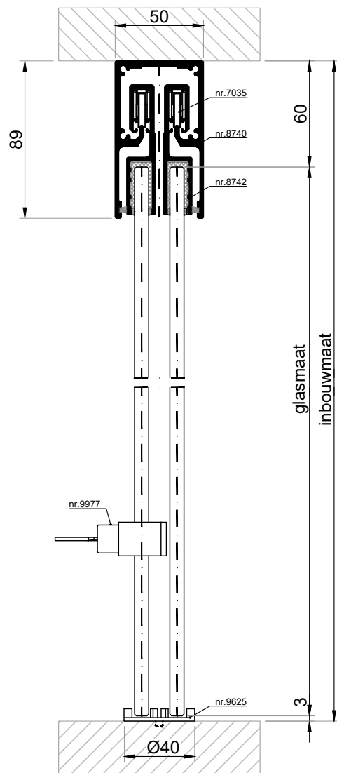
VERTICALE DOORSNEDE type HSL-9A
