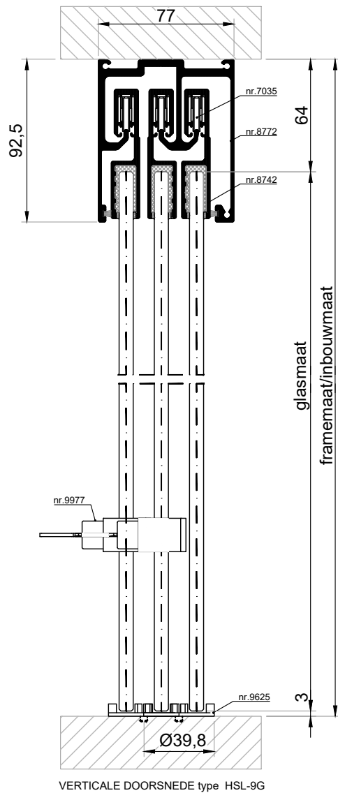
VERTICALE DOORSNEDE type HSL-9G
