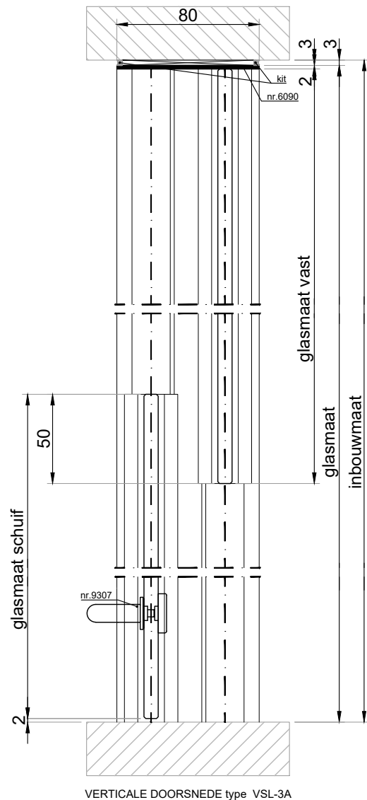
VERTICALE DOORSNEDE type VSL-3A
