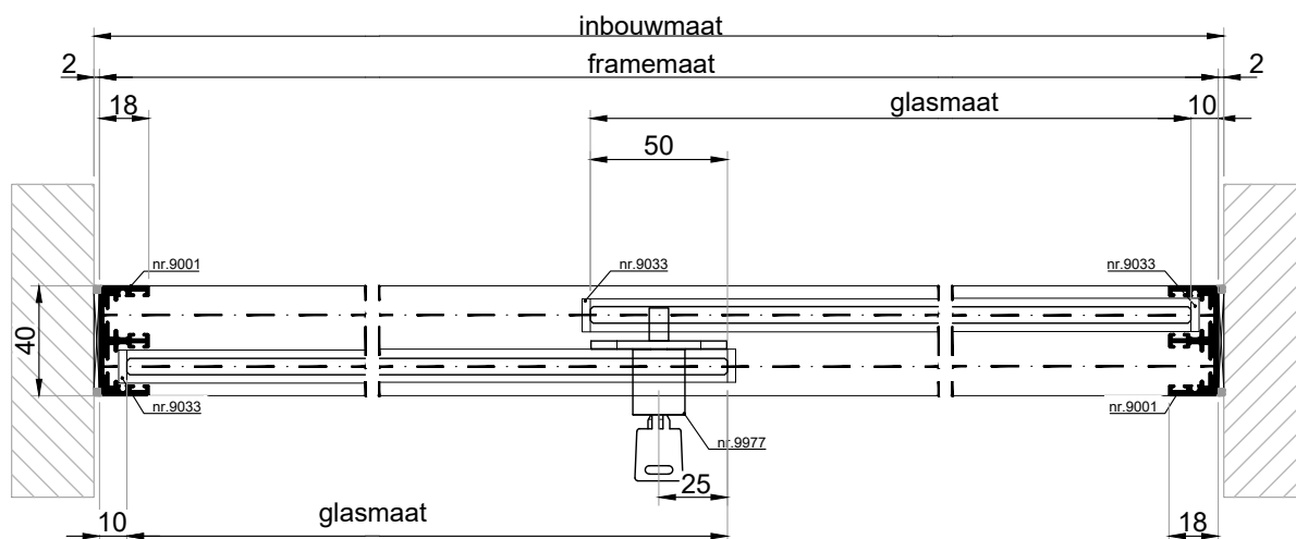
HORIZONTALE DOORSNEDE type HSL-2A
