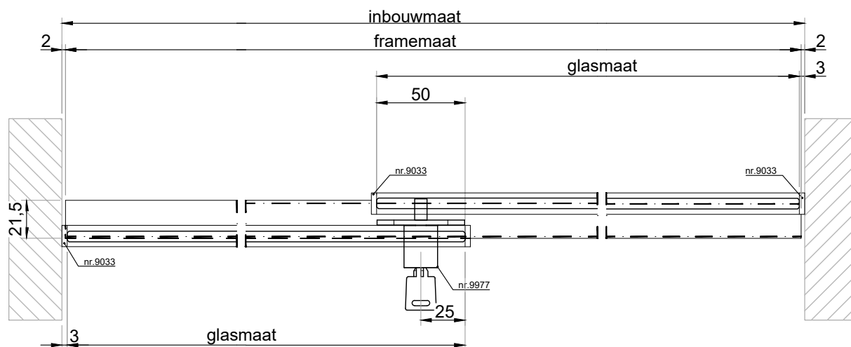
HORIZONTALE DOORSNEDE type HSL-5A
