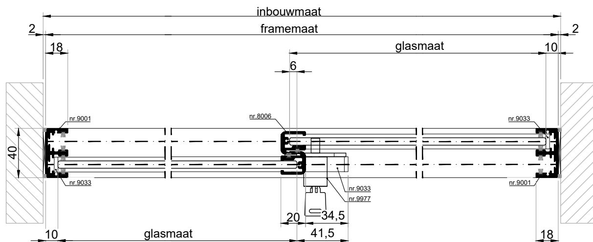
HORIZONTALE DOORSNEDE type HSL-4A
