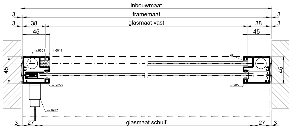
HORizontale DOORSNEDE type VSL-2A
