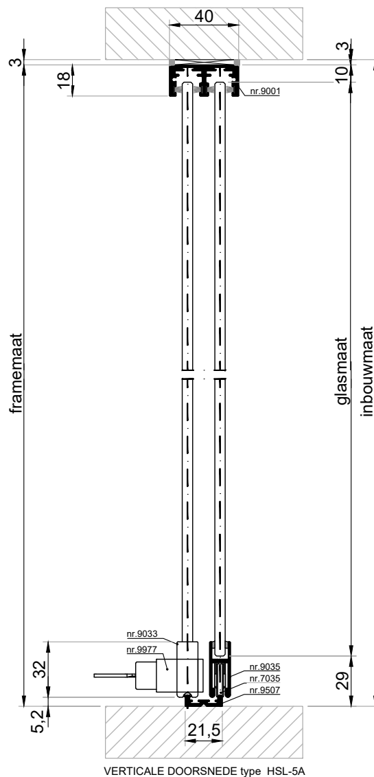
VERTICALE DOORSNEDE type HSL-5A
