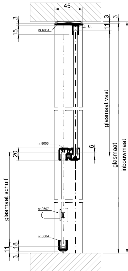
VERTICALE DOORSNEDE type VSL-2A
