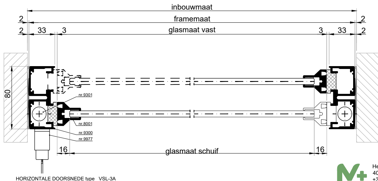
HORIZONTALE DOORSNEDE type VSL-3A
