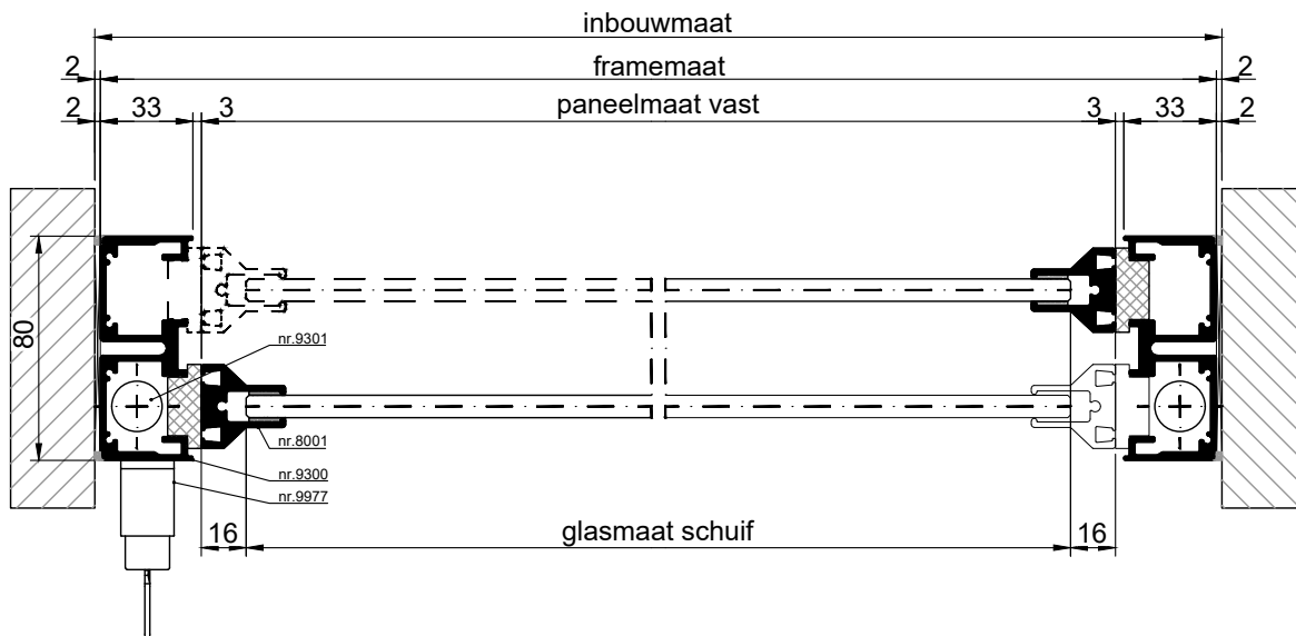
HORizontale Doorsnede type VSL-4A
