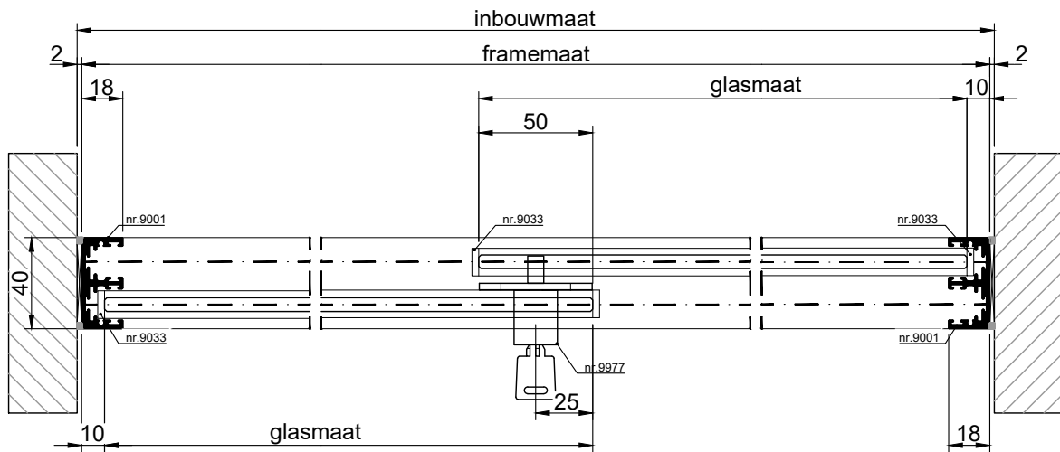
HORizontale Doorsnede type HSL-2A
