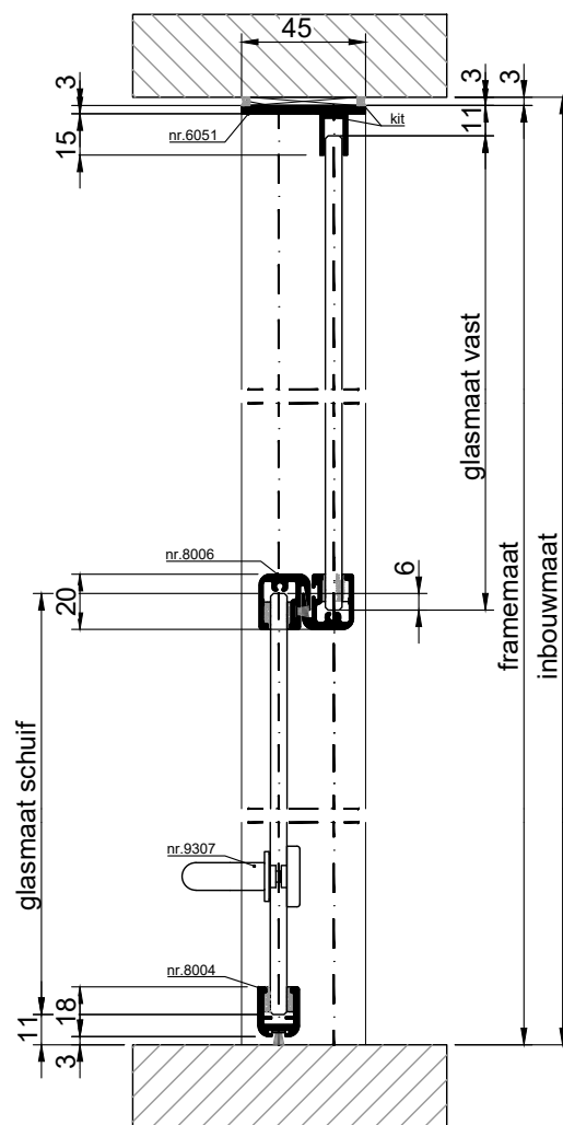
VERTICALE DOORSNEDE type VSL-2A
