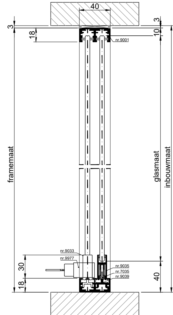
VERTICALE DOORSNEDE type HSL-2D
