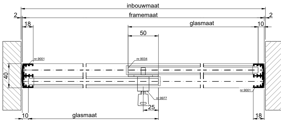
HORIZONTALE DOORSNEDE type HSL-3A
