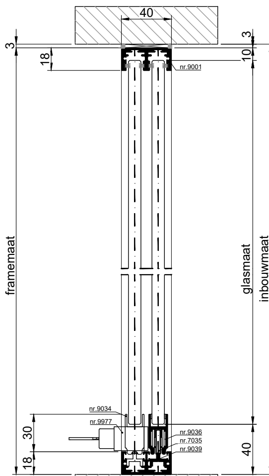
VERTICALE DOORSNEDE type HSL-3A
