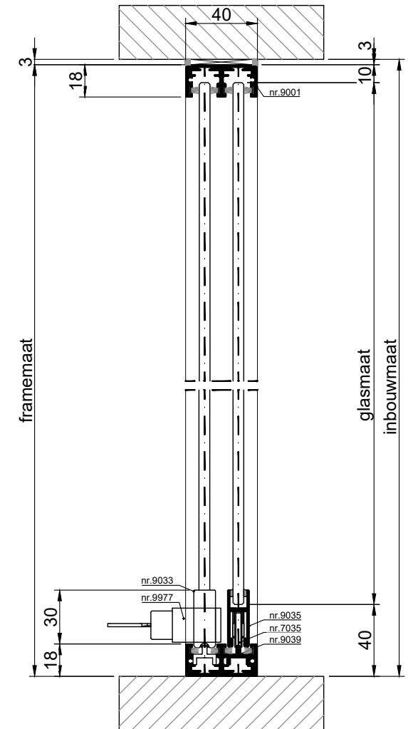
VERTICALE DOORSNEDE type HSL-4E
