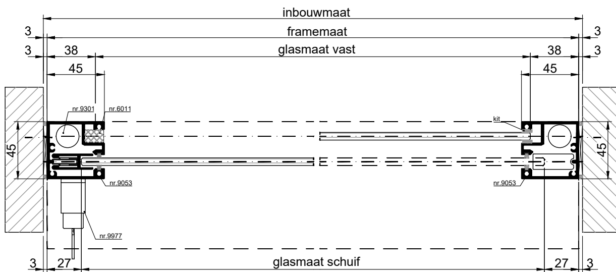
HORIZONTALE DOORSNEDE type VSL-1A
