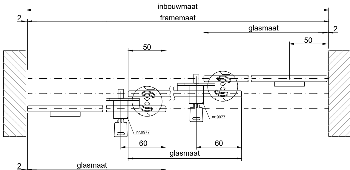
HORIZONTALE DOORSNEDE type HSL-9G
