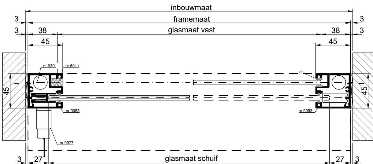
HORIZONTALE DOORSNEDE type VSL-2A
