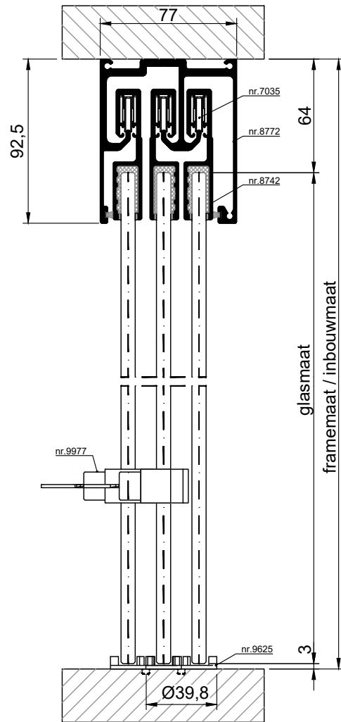
VERTICALE DOORSNEDE type HSL-9G
