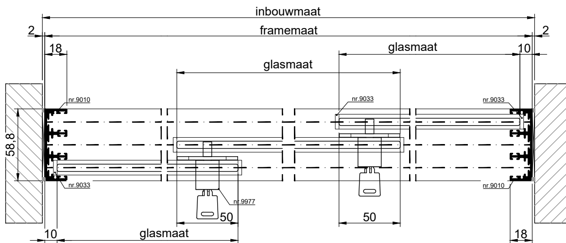
HORIZONTALE DOORSNEDE type HSL-2G
