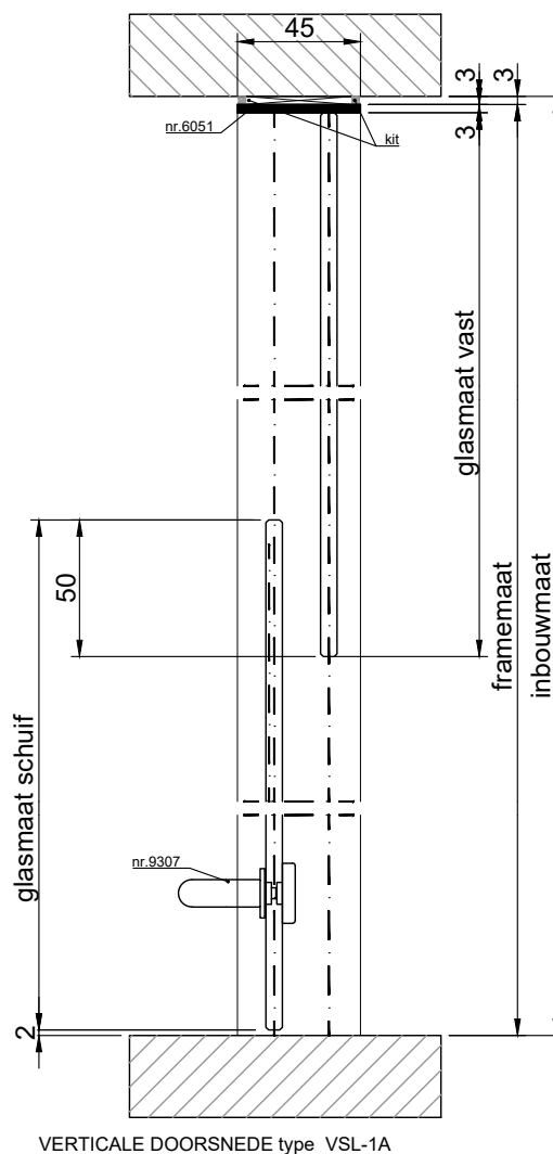
VERTICALE DOORSNEDE type VSL-1A
