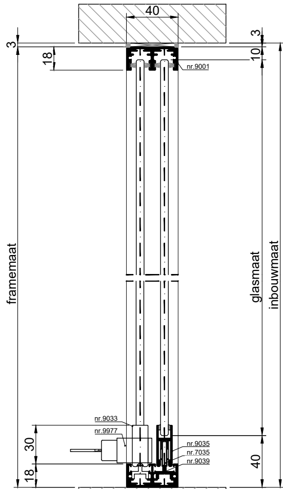
VERTICALE DOORSNEDE type HSL-2A
