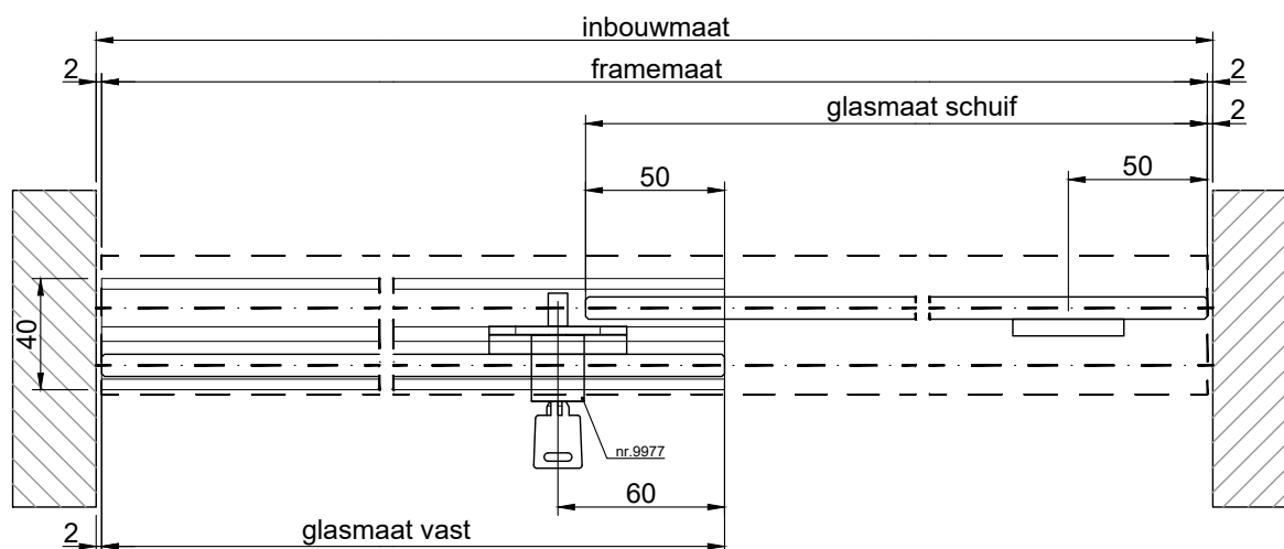
HORIZONTALE DOORSNEDE type HSL-10B
