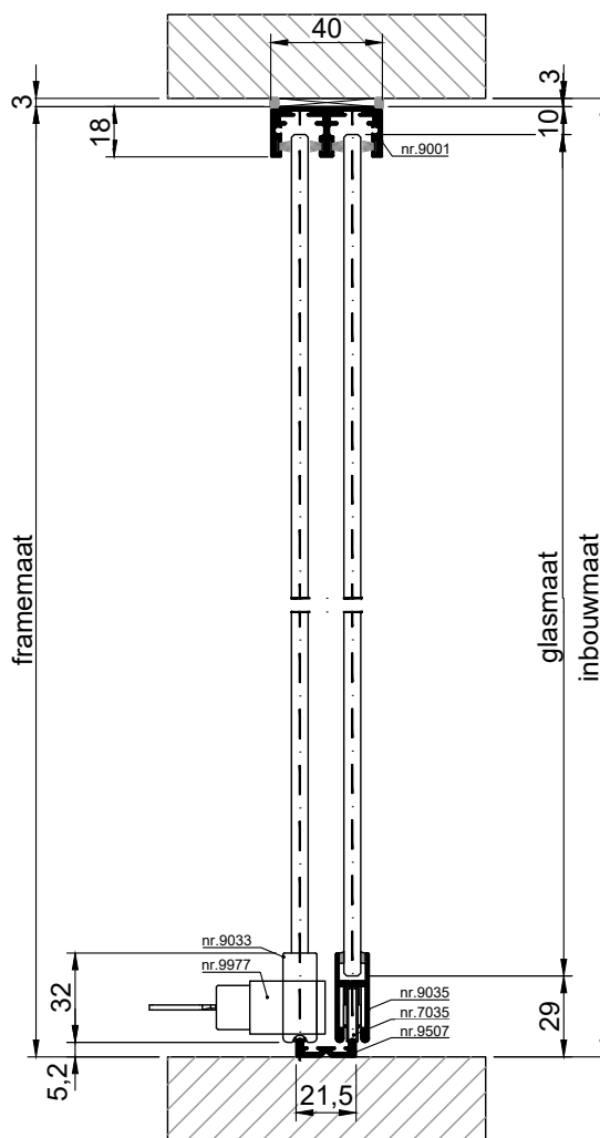
VERTICALE DOORSNEDE type HSL-5A
