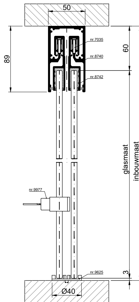
VERTICALE DOORSNEDE type HSL-9A
