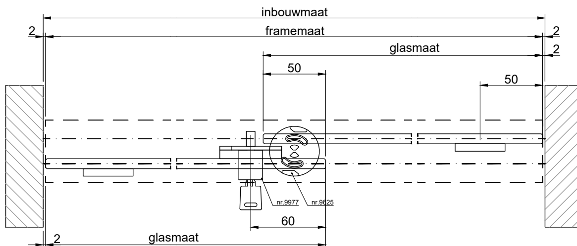
HORizontALE DOORSNEDE type HSL-9A
