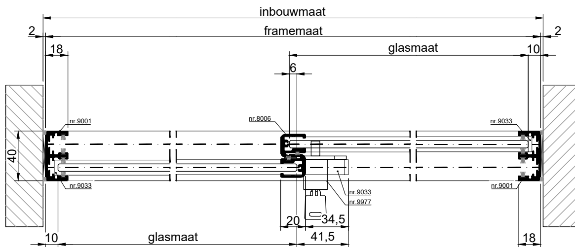
HORIZONTALE DOORSNEDE type HSL-4A
