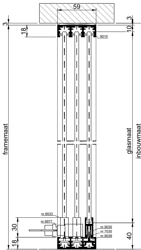
VERTICALE DOORSNEDE type HSL-2G
