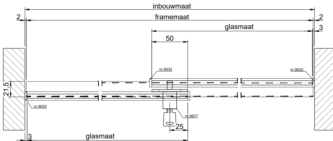
HORIZONTALE DOORSNEDE type HSL-5A
