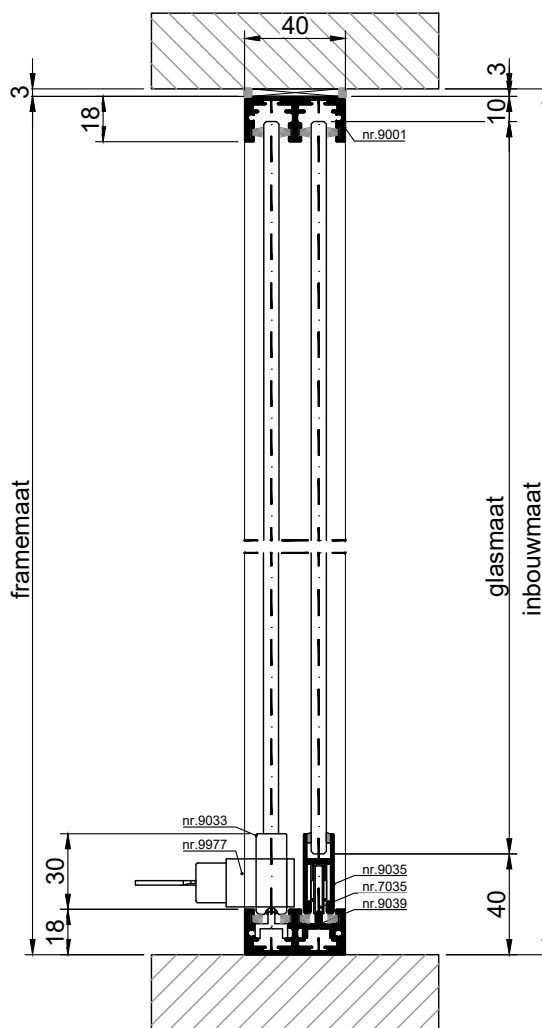
VERTICALE DOORSNEDE type HSL-4A
