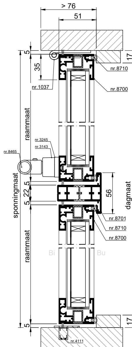
VERTICALE DOORSNEDE type AMC-20
