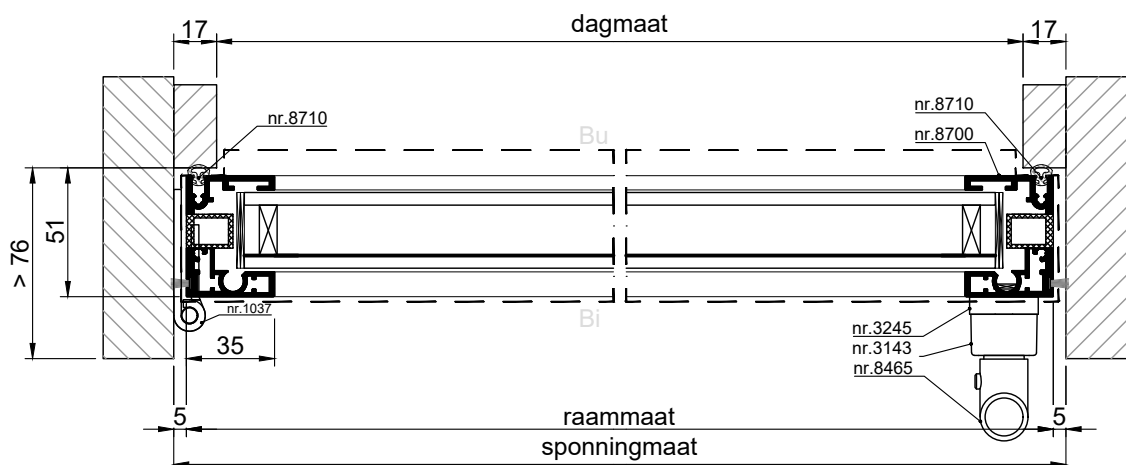
HORIZONTALE DOORSNEDE type AMC-20
