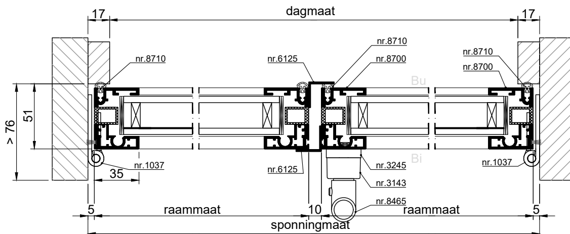
HORIZONTALE DOORSNEDE type AMS-20
