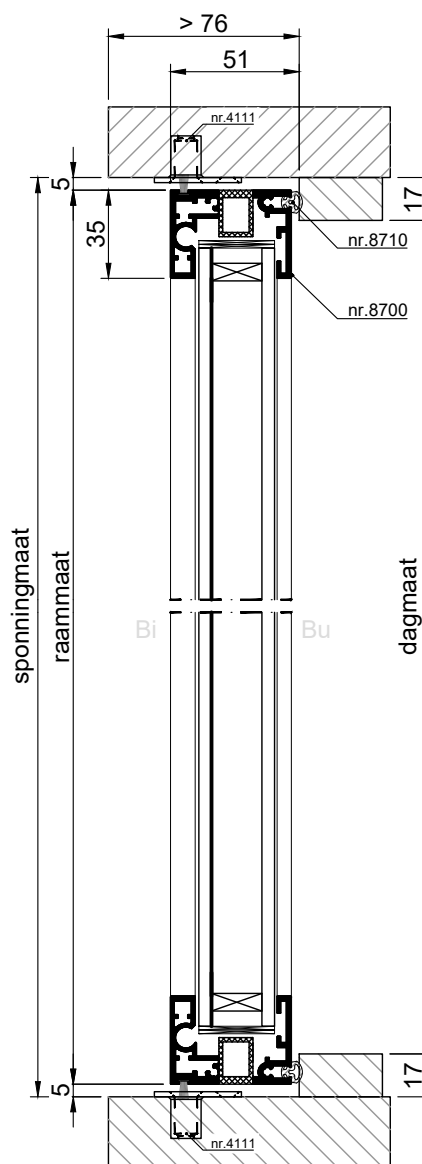
VERTICALE DOORSNEDE type AMD-20
