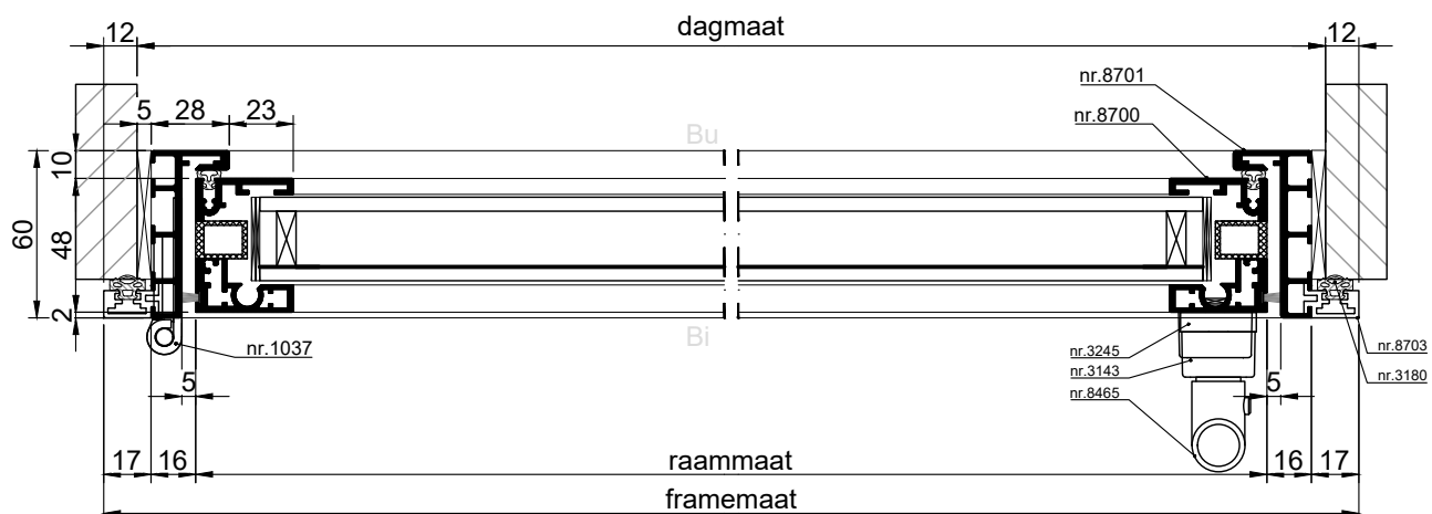
HORIZONTALE DOORSNEDE type AMD-10
