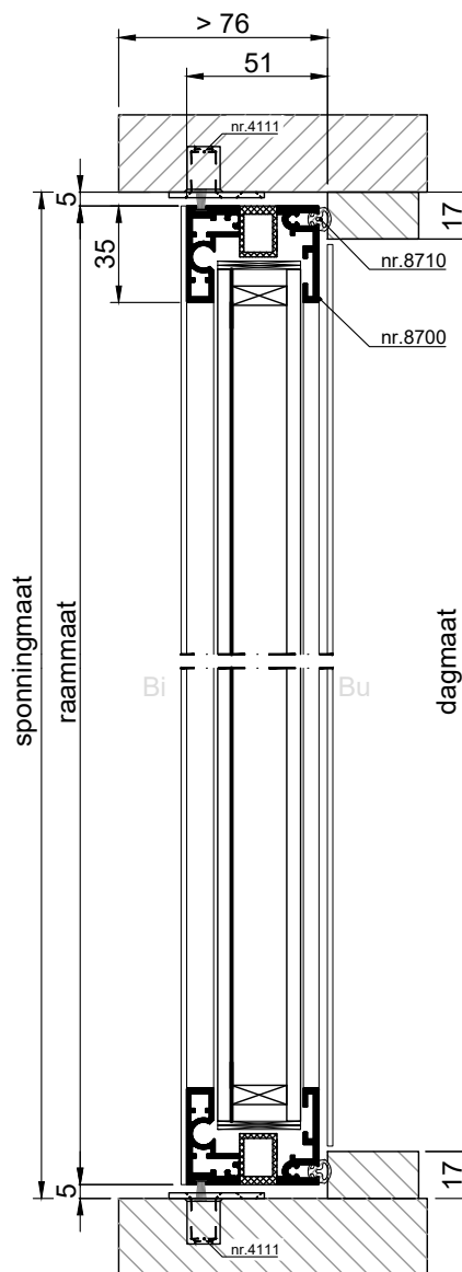
VERTICALE DOORSNEDE type AMS-20
