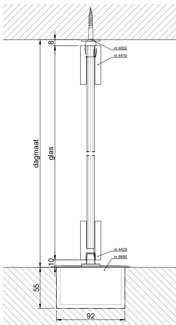
VERTICALE DOORSNEDE type TPS-1A
