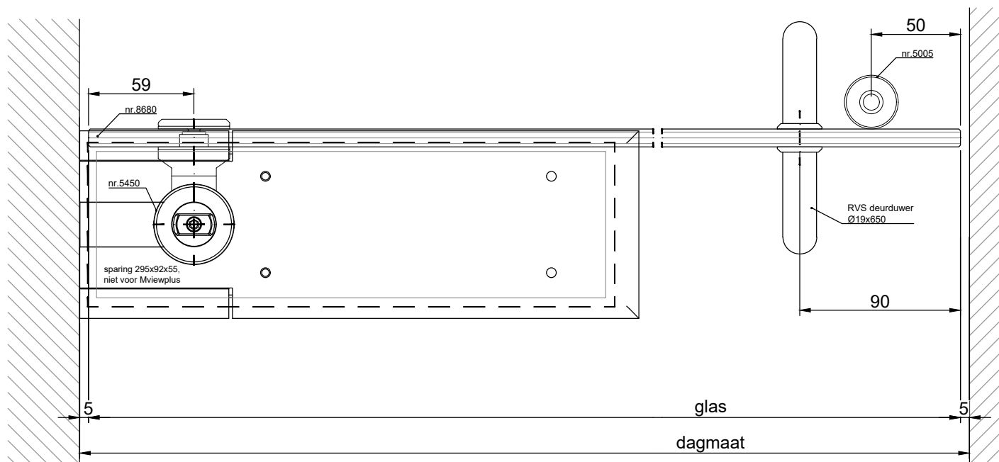
HORizontale DOORSNEDE type TPM-1F
