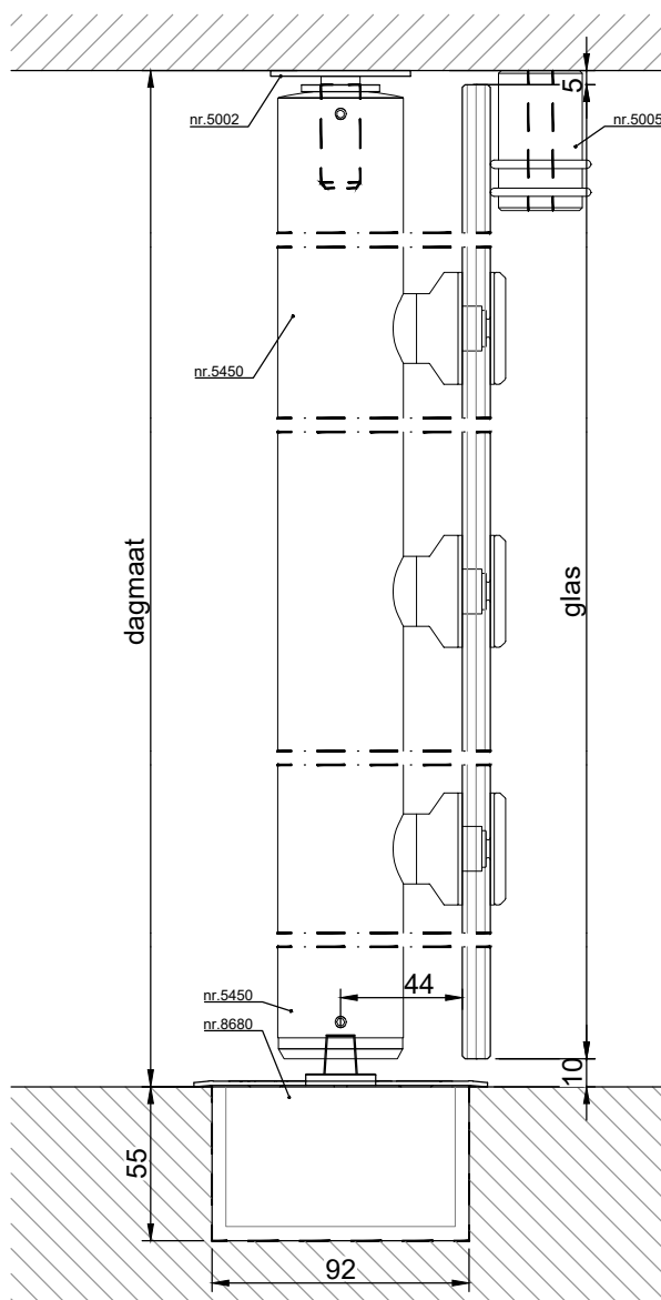
VERTICALE DOORSNEDE type TPM-1F
