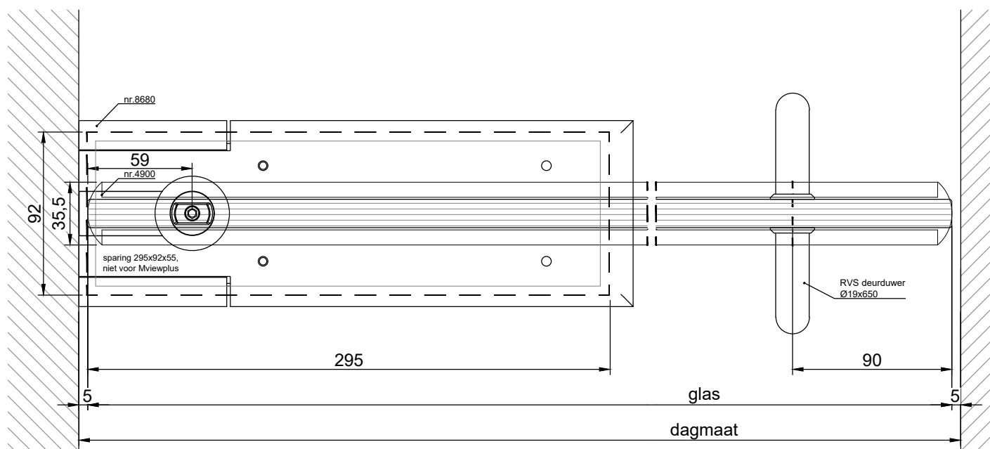
HORIZONTALE DOORSNEDE type TPT-1C
