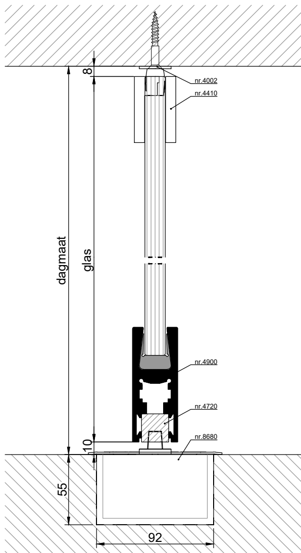
VERTICALE DOORSNEDE type TPT-1C
