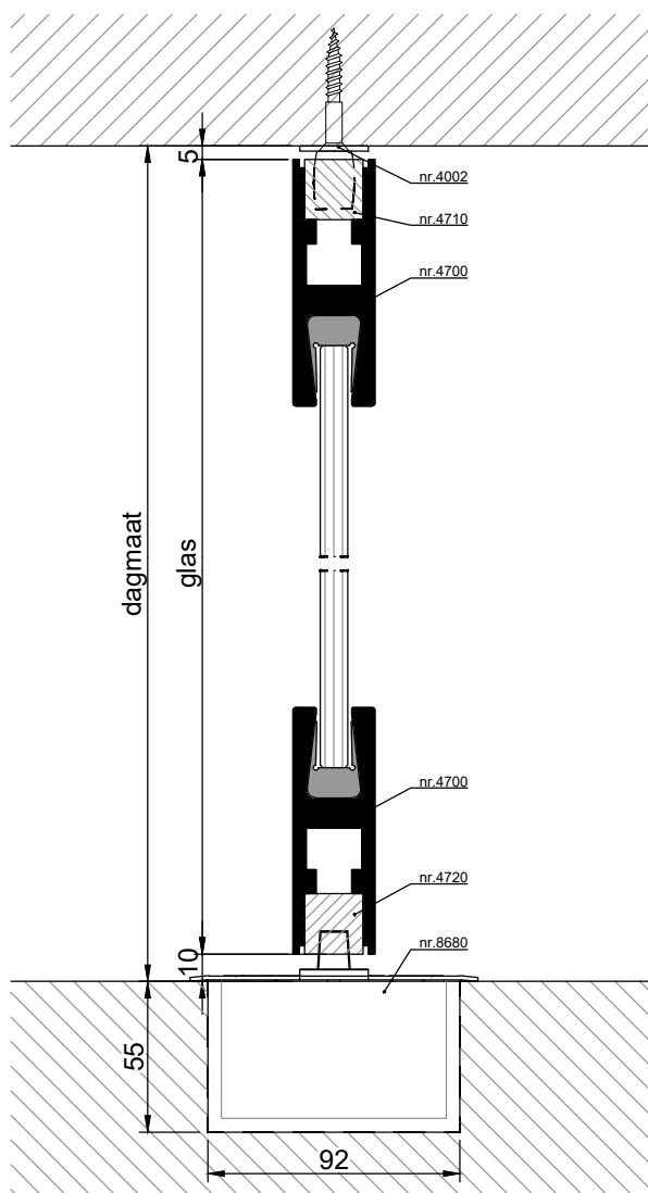
VERTICALE DOORSNEDE type TPP-1A
