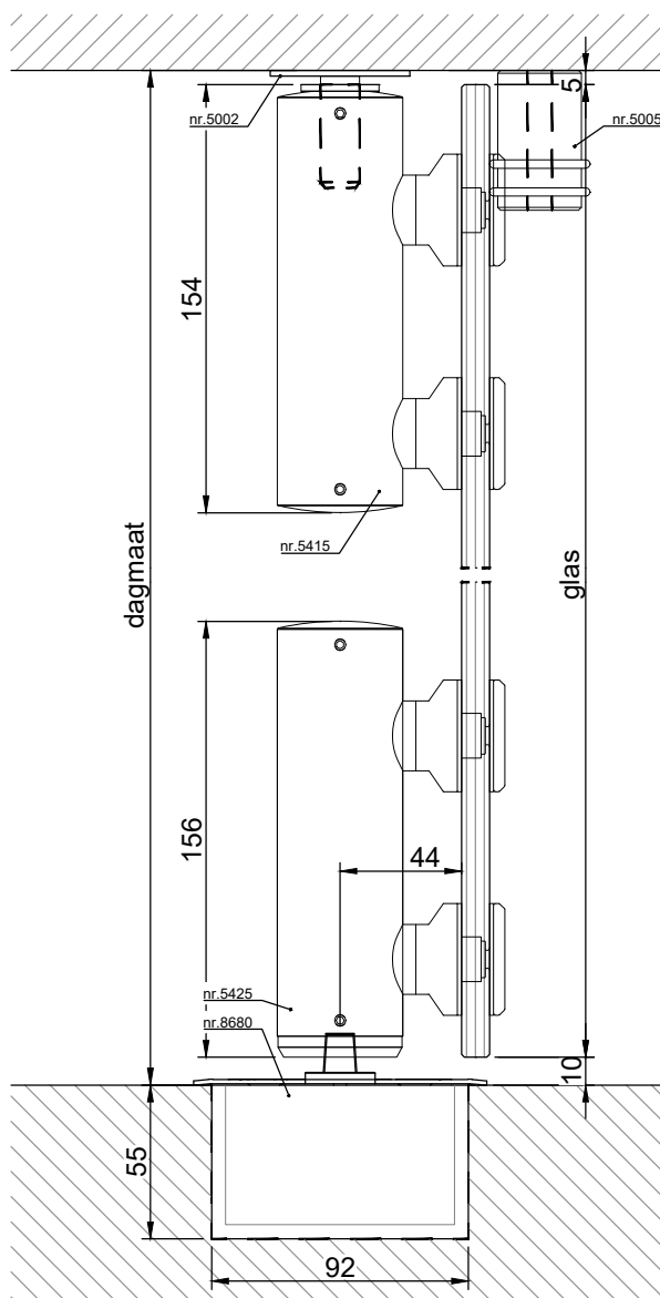
VERTICALE DOORSNEDE type TPM-1E
