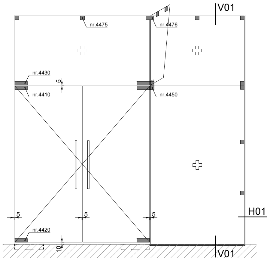
TOTAL GLAS PUI TYPE 21 GESTABILISEERD MET GLASKLEMMEN
