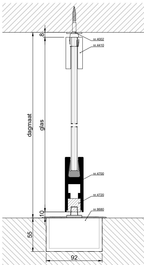
VERTICALE DOORSNEDE type TPT-1A
