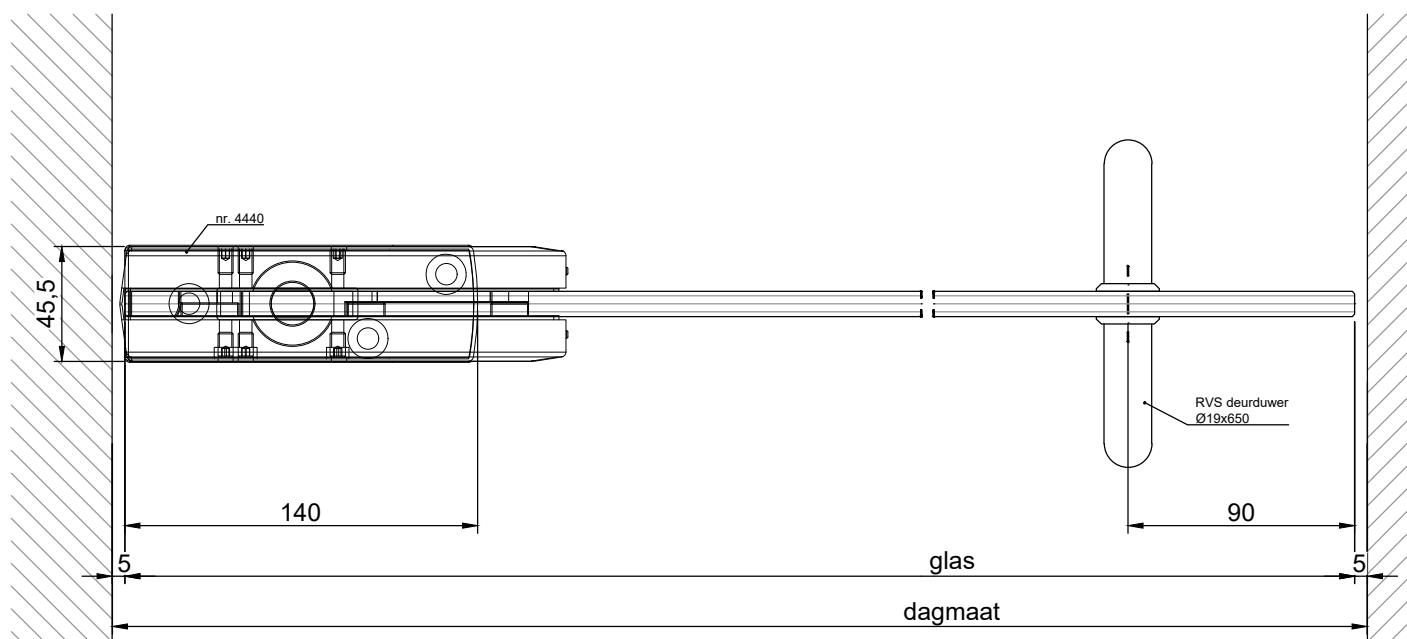
HORIZONTALE DOORSNEDE type TPS-1B
