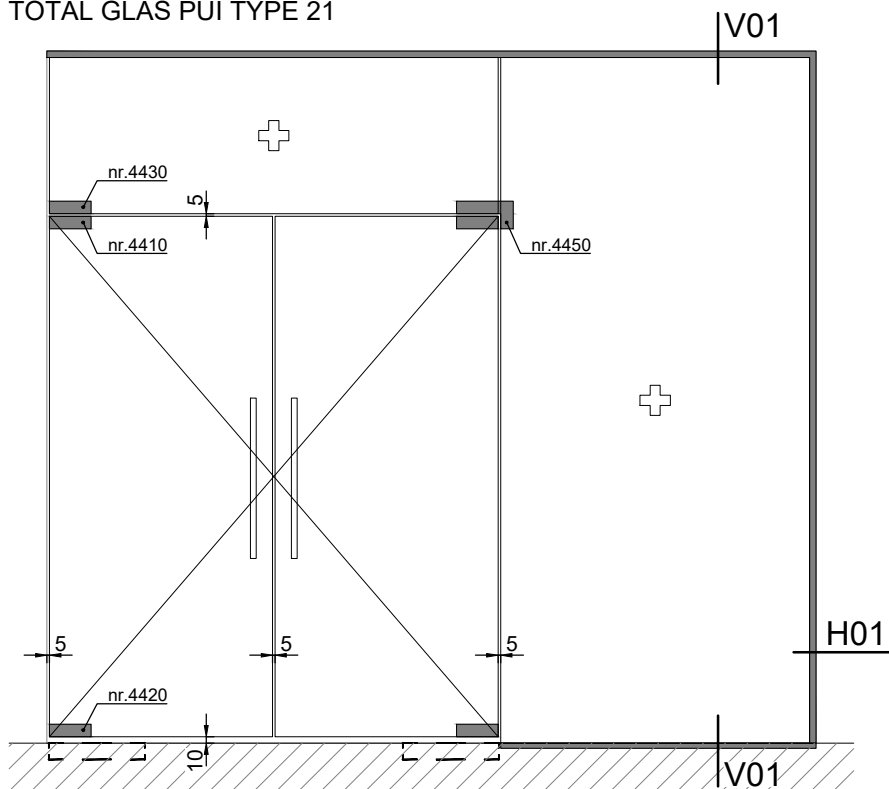
TOTAL GLAS PUI TYPE 21
