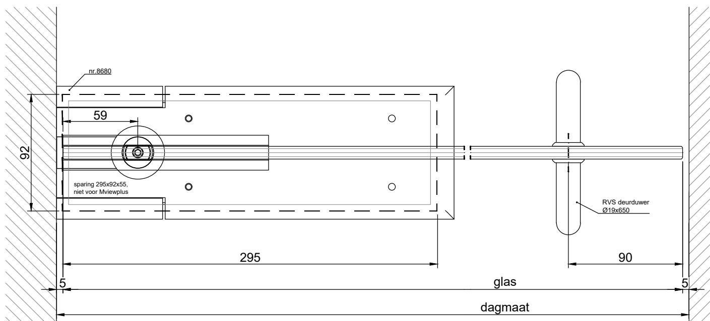
HORizontale DOORSNEDE type TPS-1A
