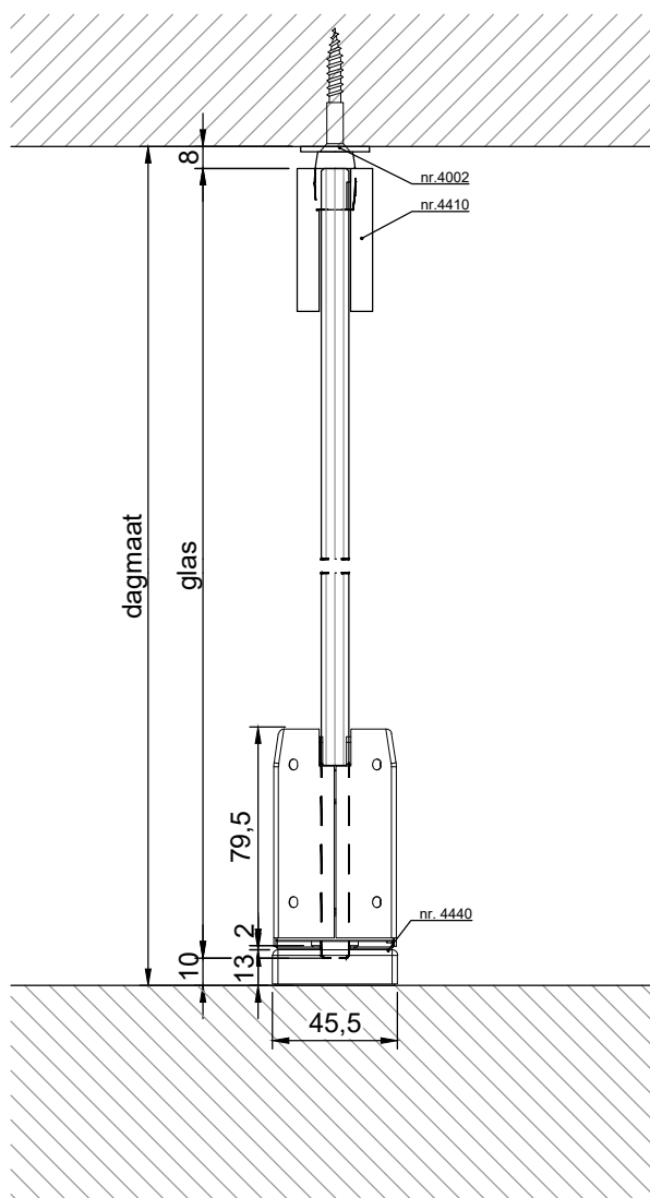
VERTICALE DOORSNEDE type TPS-1B
