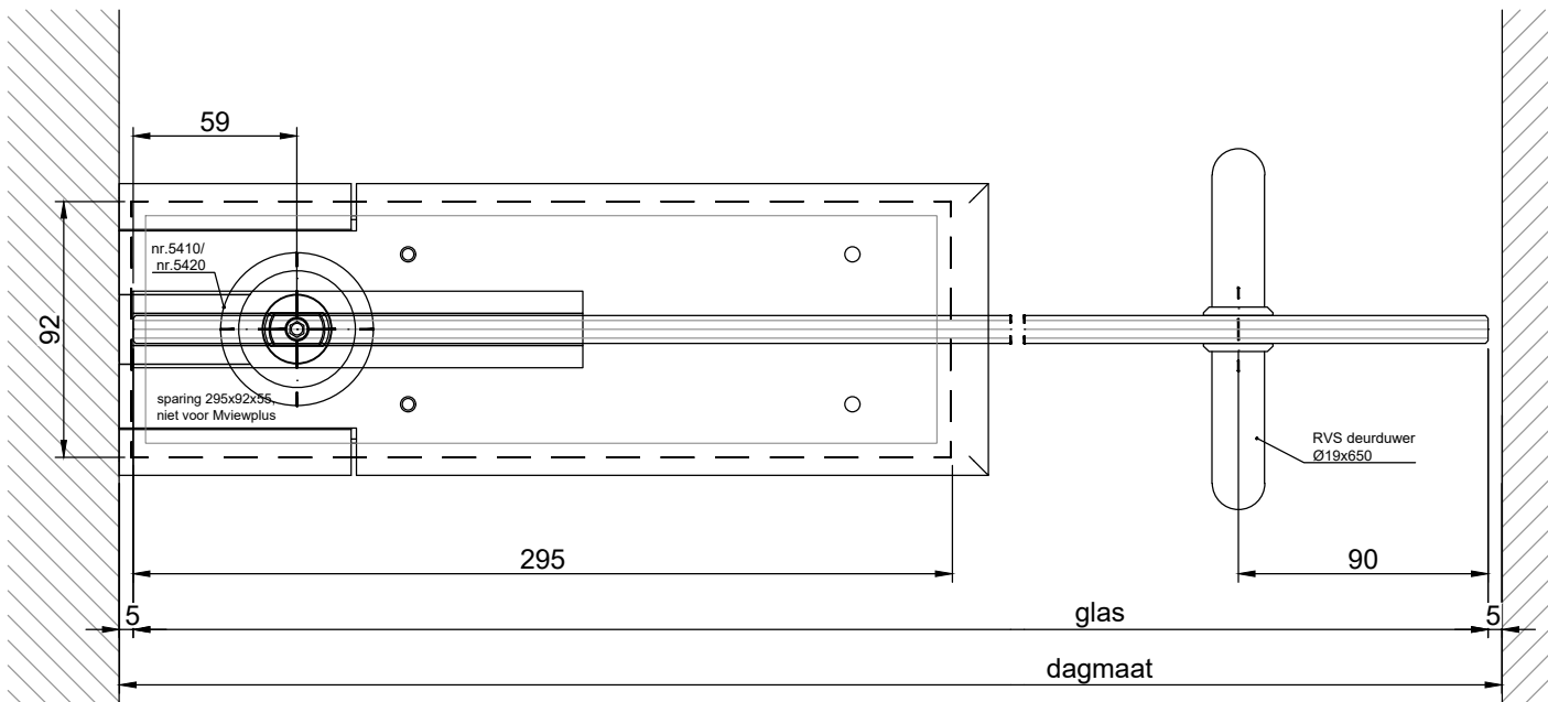
HORizontale Doorsnede type TPM-1D
