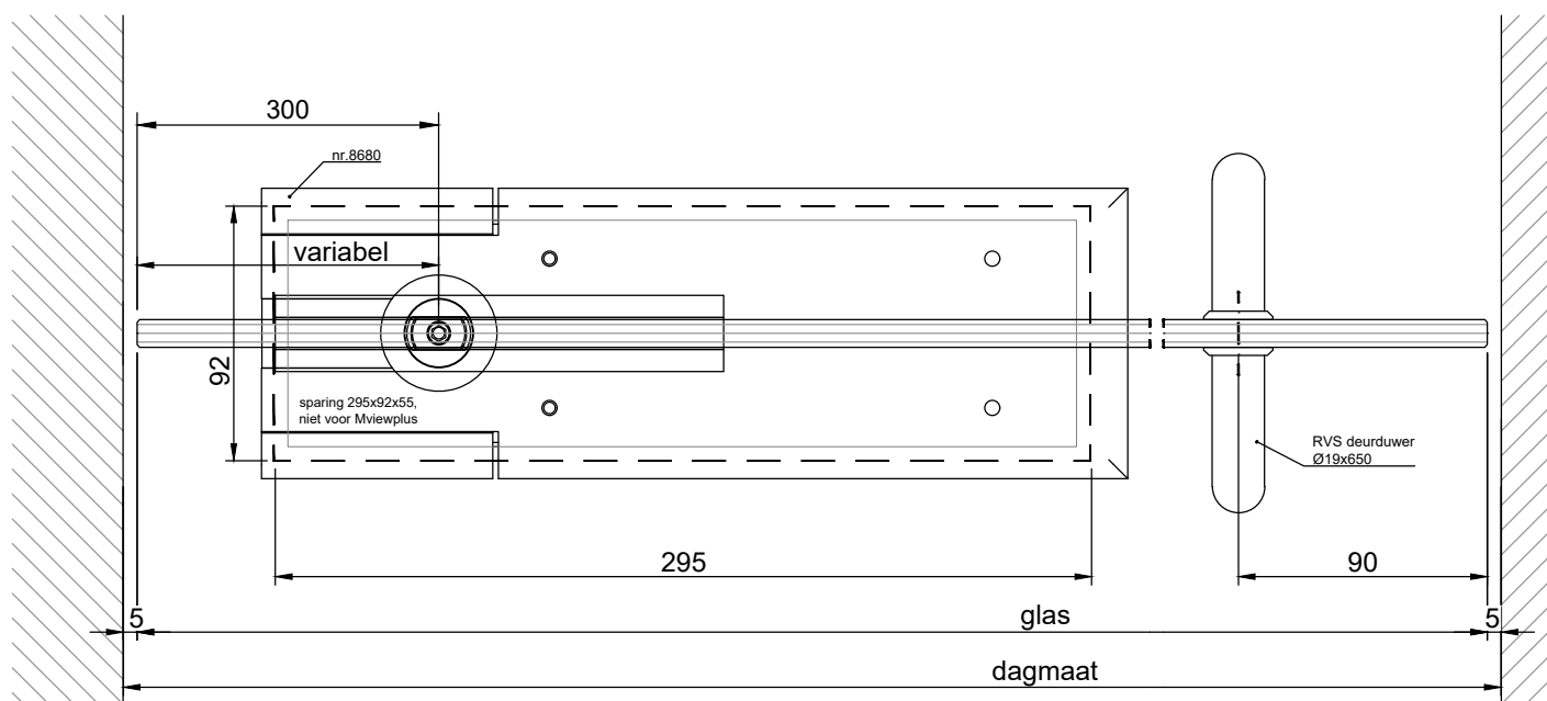
HORIZONTALE DOORSNEDE type TPS-1A300*
