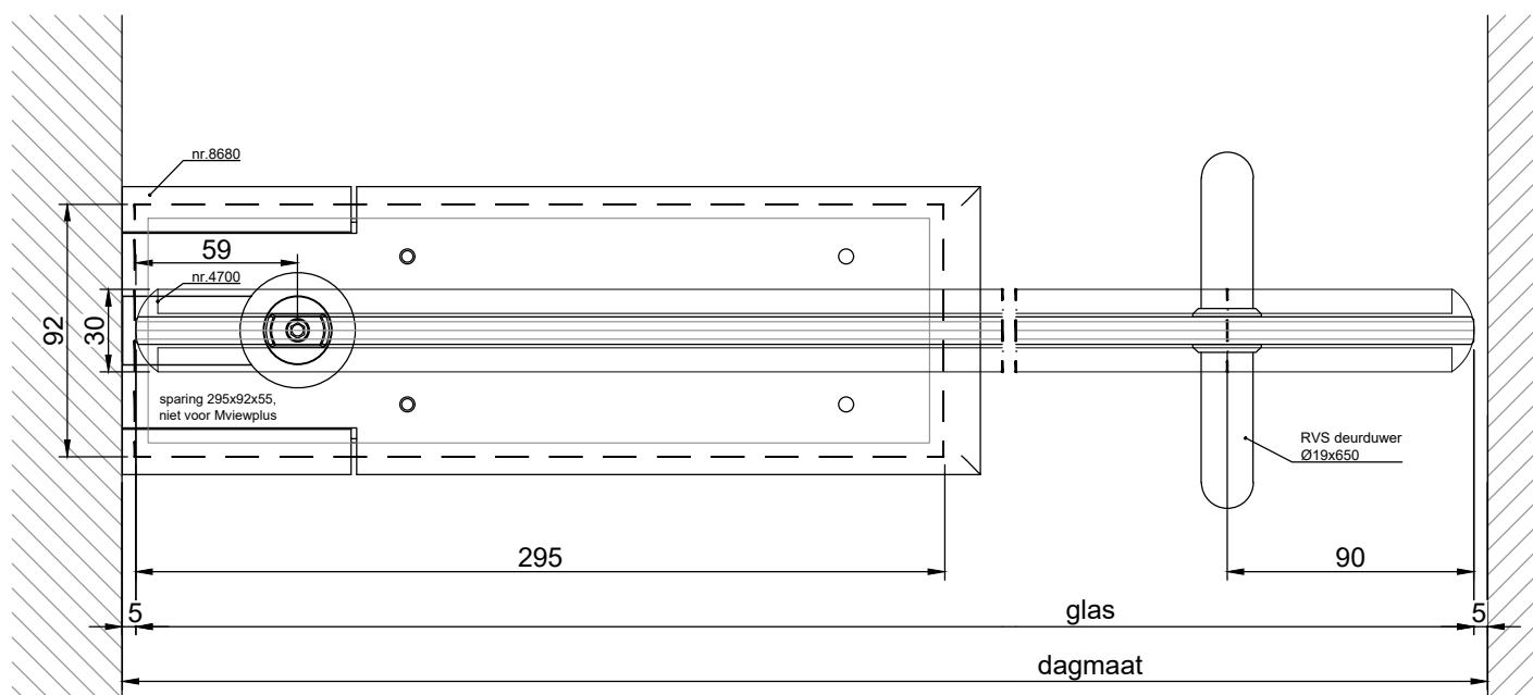
HORIZONTALE DOORSNEDE type TPP-1A
