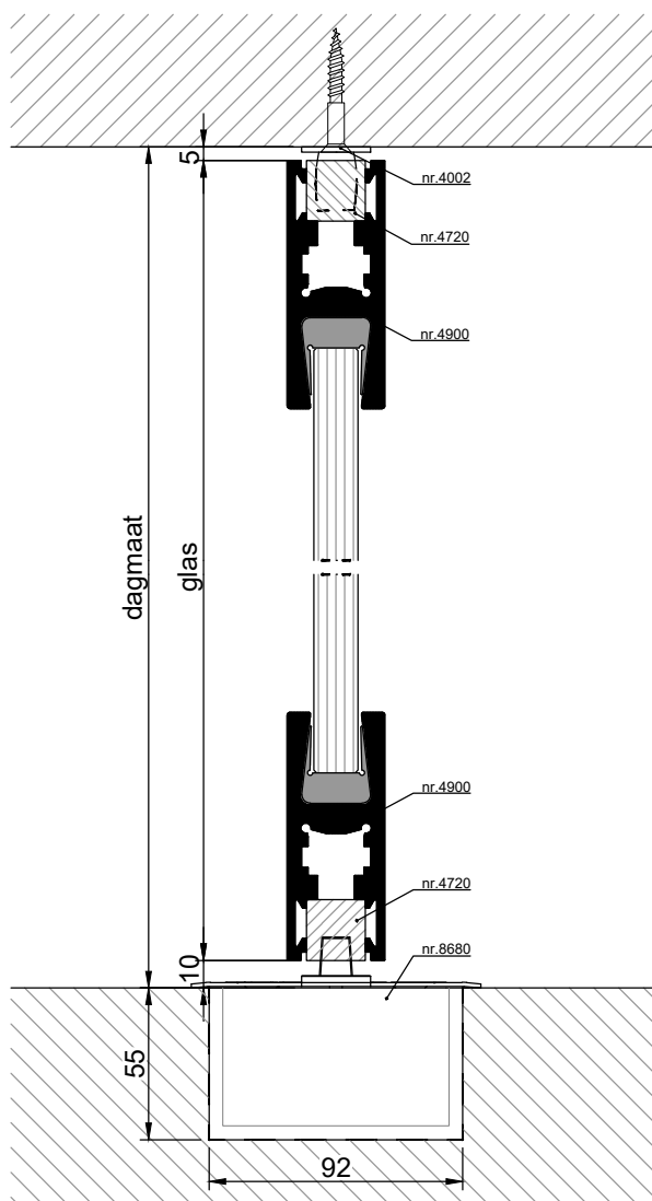
VERTICALE DOORSNEDE type TPP-1C
