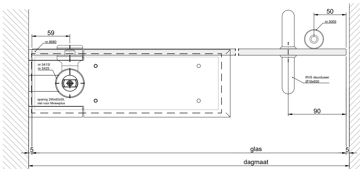
HORIZONTALE DOORSNEDE type TPM-1E
