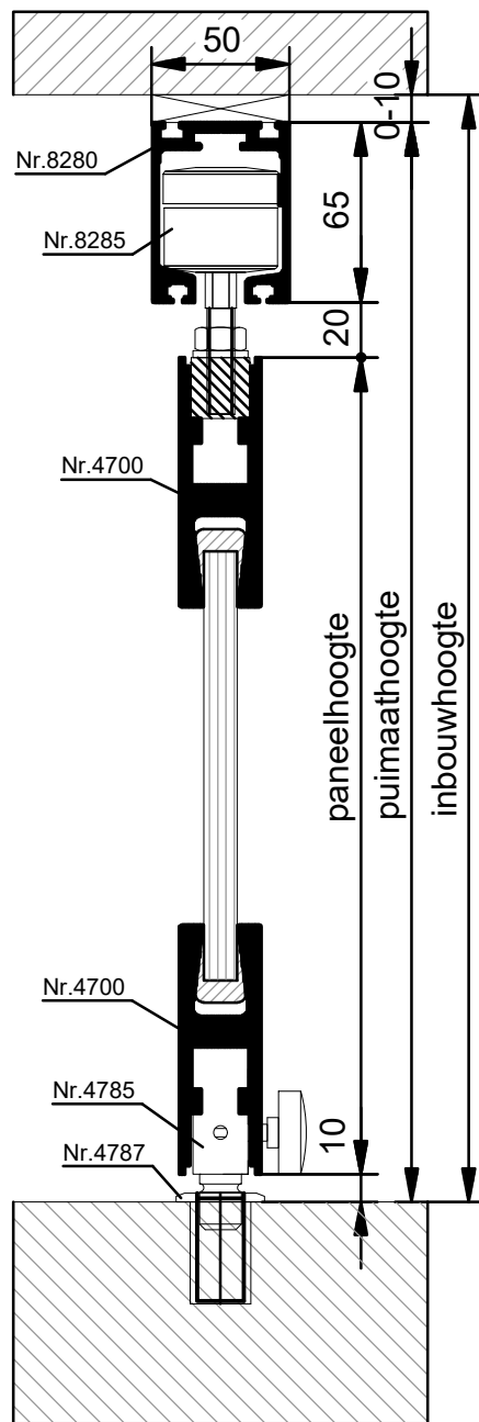
VERTICALE DOORSNEDE THP-3A
