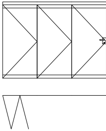
TYPE TVD-3A
