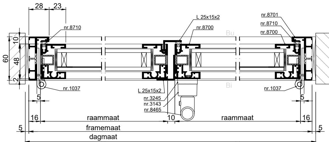
HORIZONTALE DOORSNEDE type AMS-10
