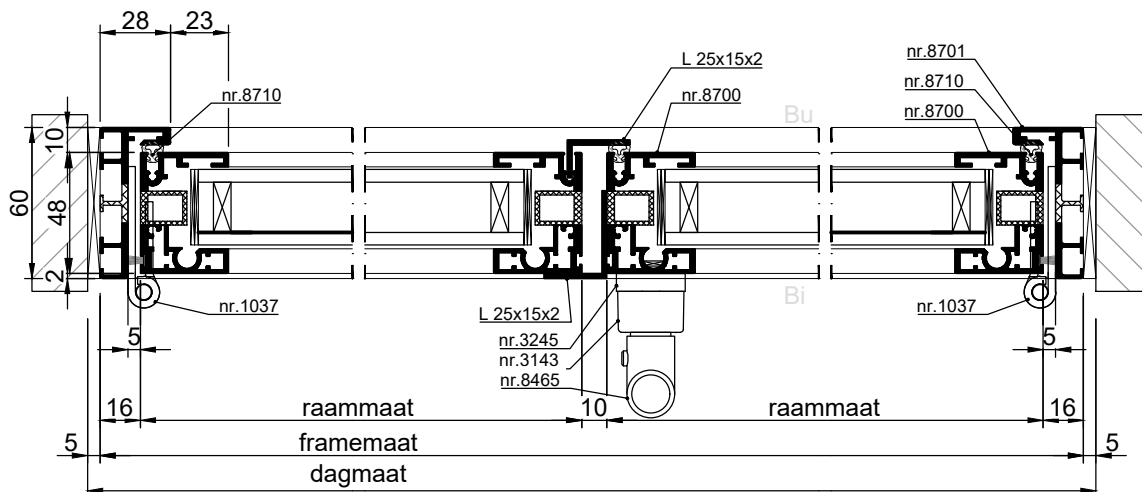
HORIZONTALE DOORSNEDE type AMC-30
