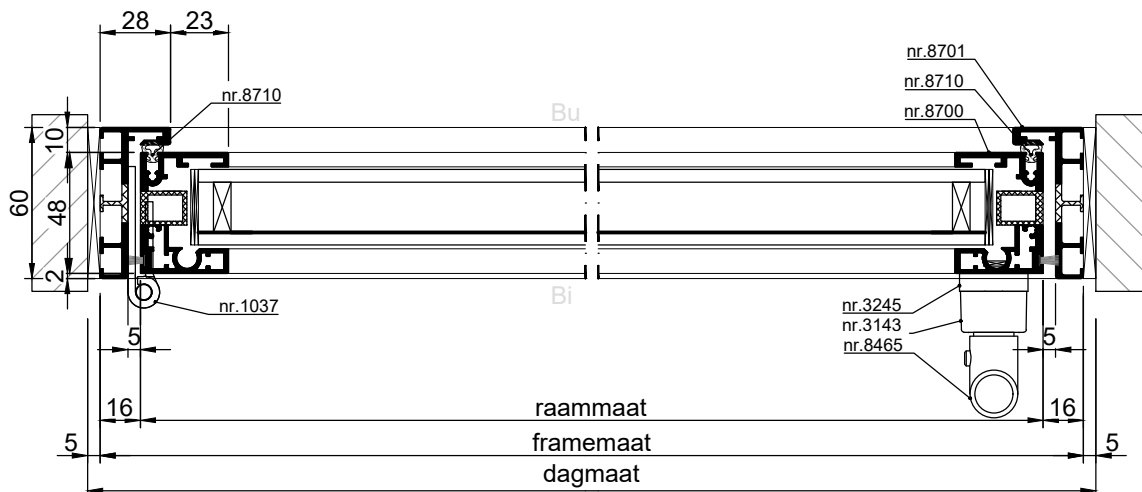
HORIZONTALE DOORSNEDE type AMD-10
