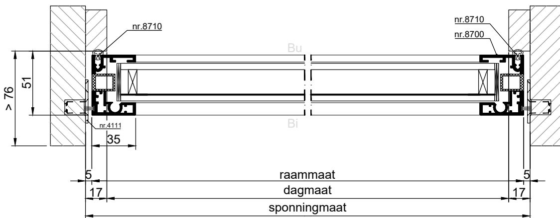
HORIZONTALE DOORSNEDE type AMK-20
