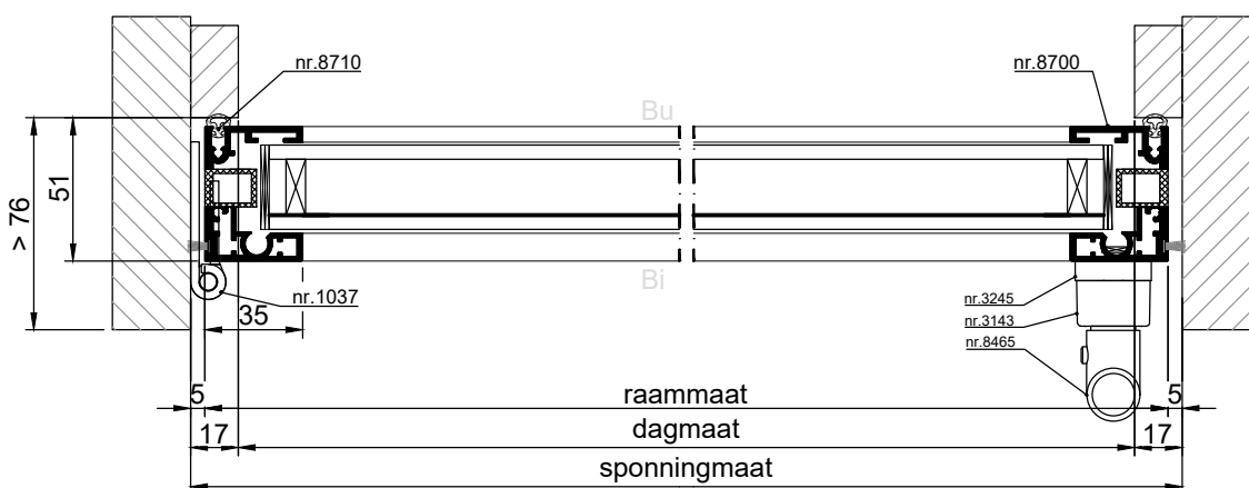
HORIZONTALE DOORSNEDE type AMD-20
