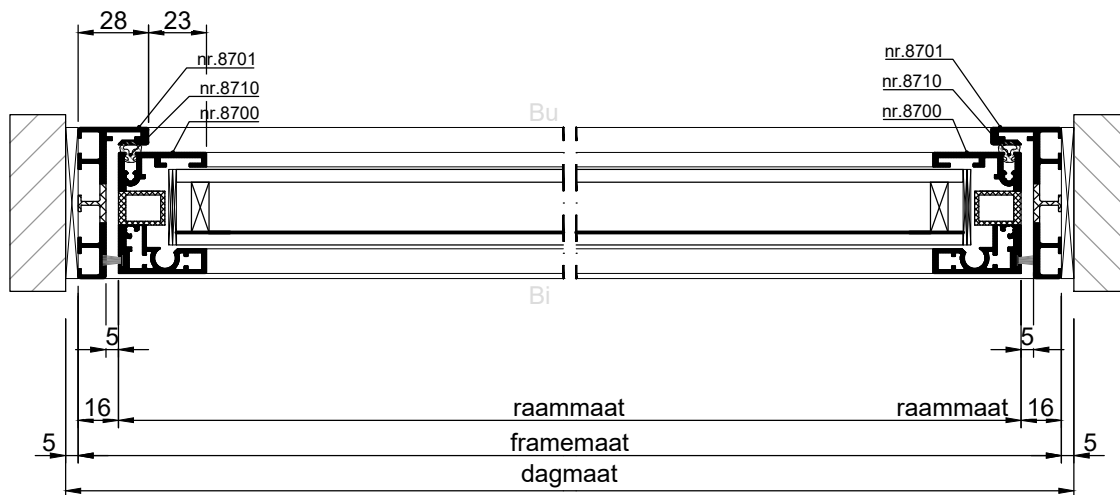
HORIZONTALE DOORSNEDE type AMK-10
