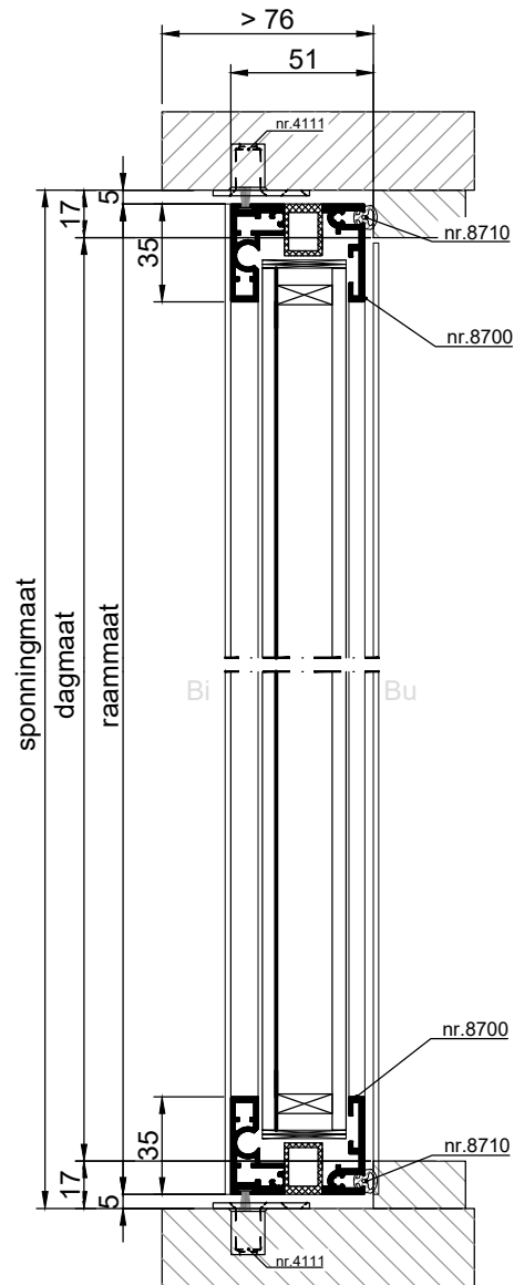
VERTICALE DOORSNEDE type AMS-20
