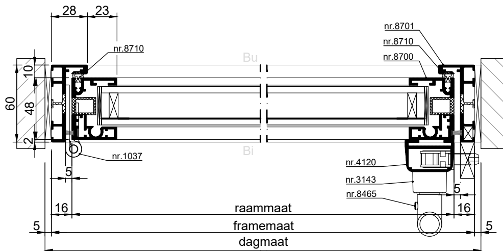
HORIZONTALE DOORSNEDE type AMD-11
