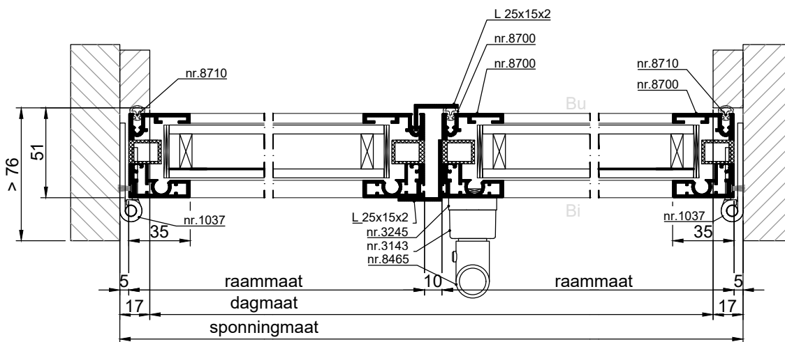
HORIZONTALE DOORSNEDE type AMS-20
