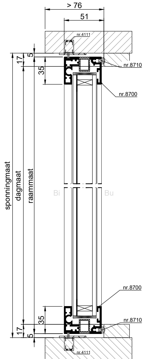
VERTICALE DOORSNEDE type AMD-20
