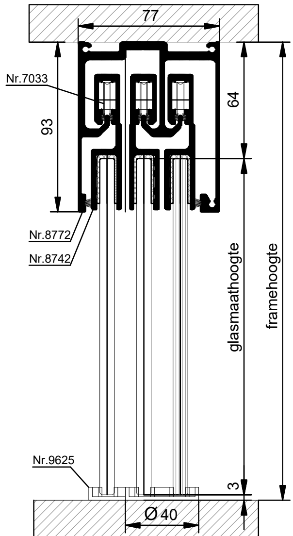
VERTICALE DOORSNEDE HSL-9G
