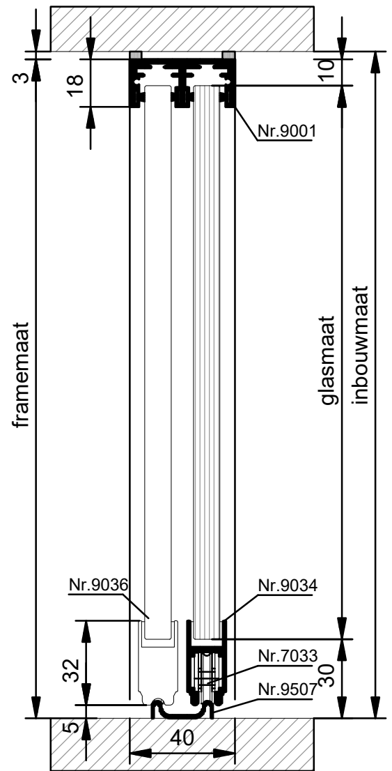
VERTICALE DOORSNEDE HSL-6A
