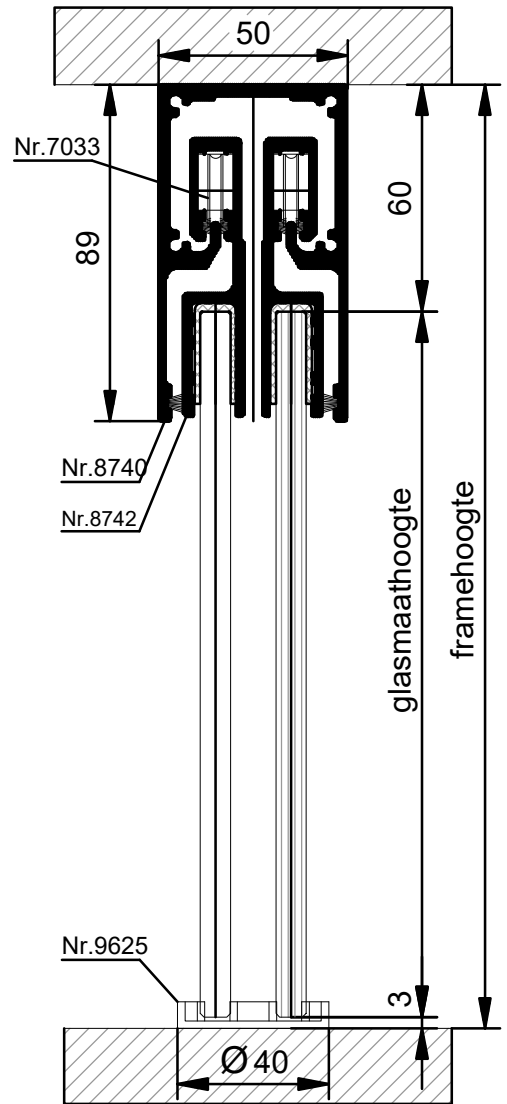
VERTICALE DOORSNEDE HSL-9A
