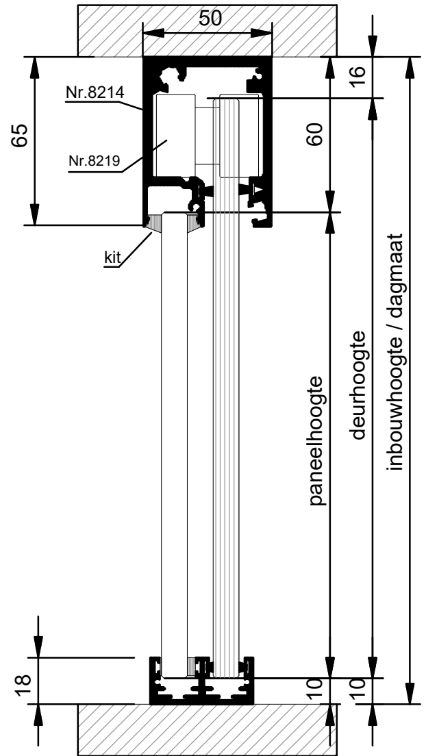
VERTICALE DOORSNEDE HSL-10B
