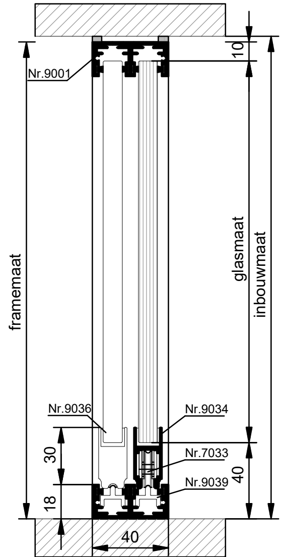
VERTICALE DOORSNEDE HSL-3A
