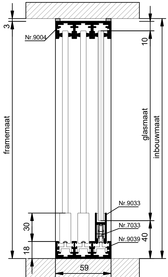
VERTICALE DOORSNEDE HSL-2G
