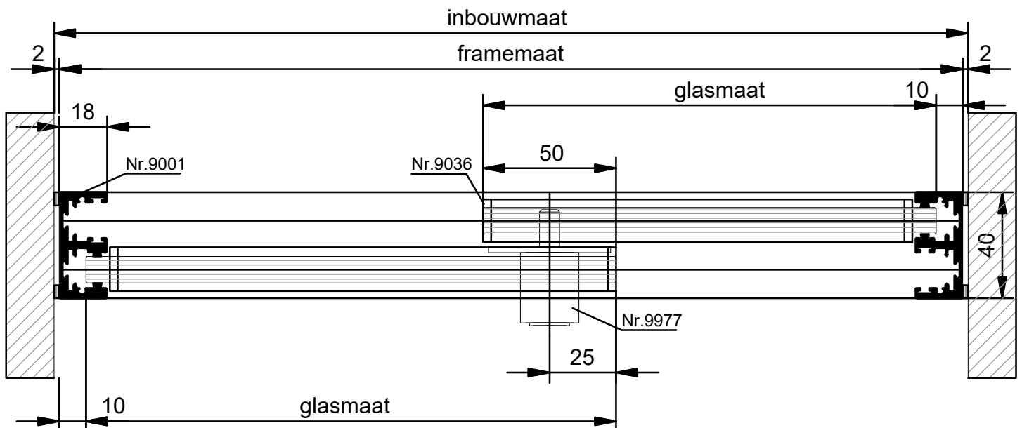
HORIZONTALE DOORSNEDE HSL-3A
