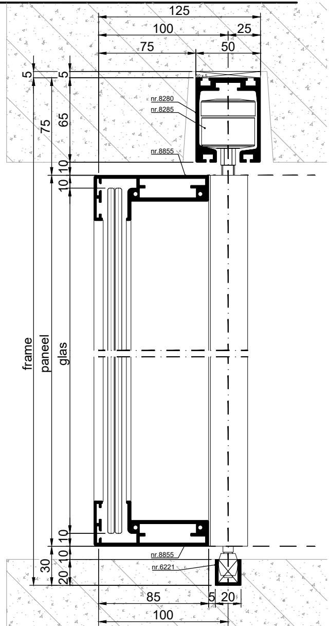
VERTICALE DOORSNEDE type BSV-4
