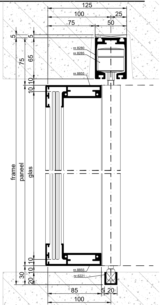
VERTICALE DOORSNEDE type BSV-2
