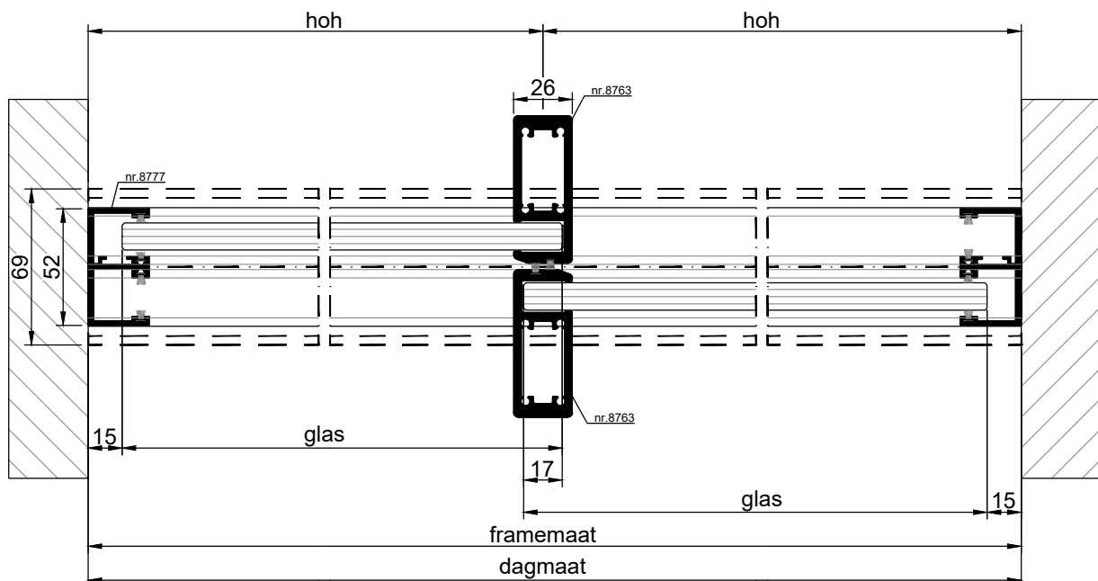
HORIZONTALE DOORSNEDE type BSH-22A
