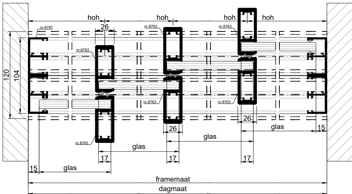
HORIZONTALE DOORSNEDE type BSH-44A
