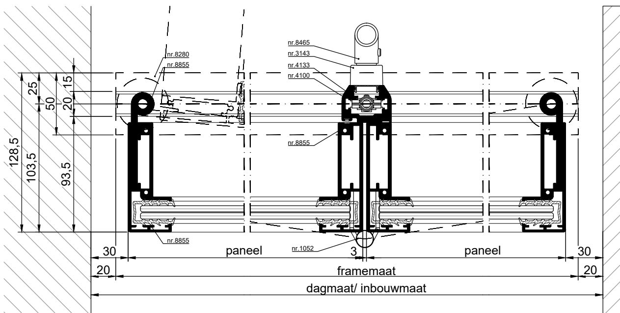
HORIZONTALE DOORSNEDE type BSV-2
