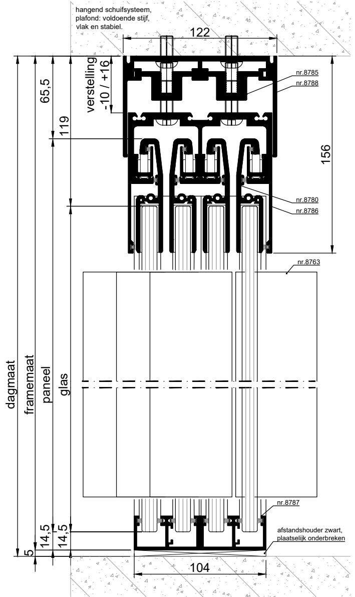
VERTICALE DOORSNEDE type BSH-44A
