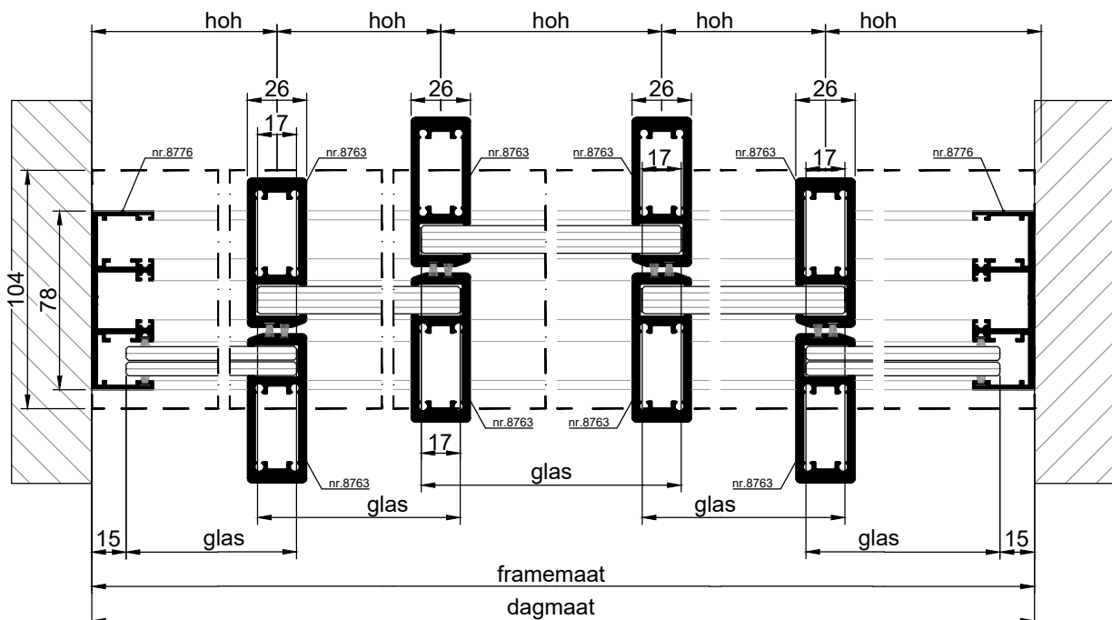
HORIZONTALE DOORSNEDE type BSH-35A
