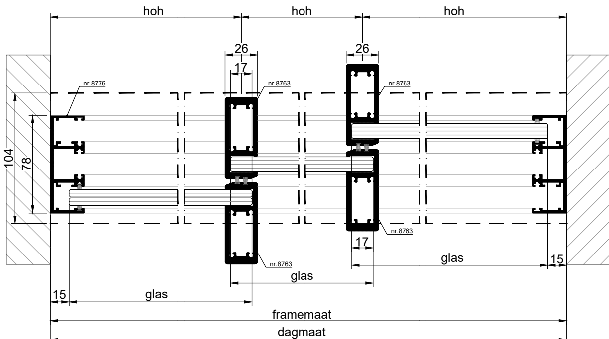
HORIZONTALE DOORSNEDE type BSH-33A
