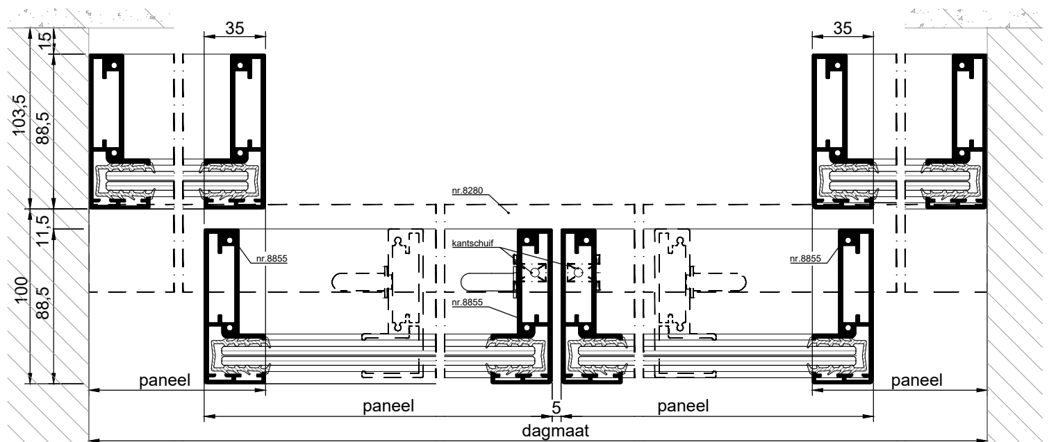
HORIZONTALE DOORSNEDE type BSH-10C
