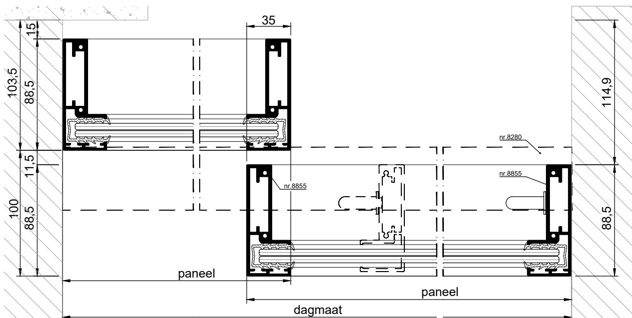
HORIZONTALE DOORSNEDE type BSH-10A
