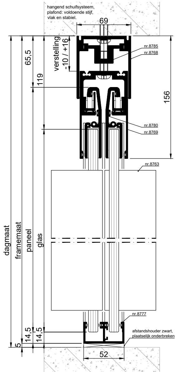
VERTICALE DOORSNEDE type BSH-22A
