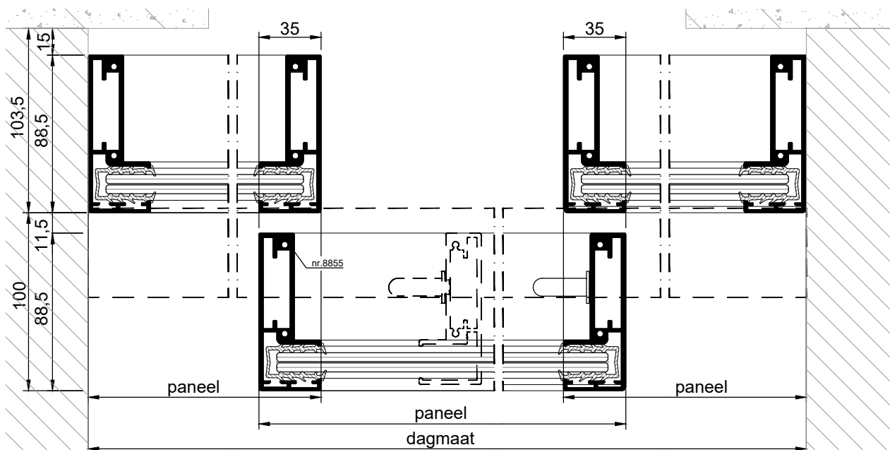
HORIZONTALE DOORSNEDE type BSH-10C
