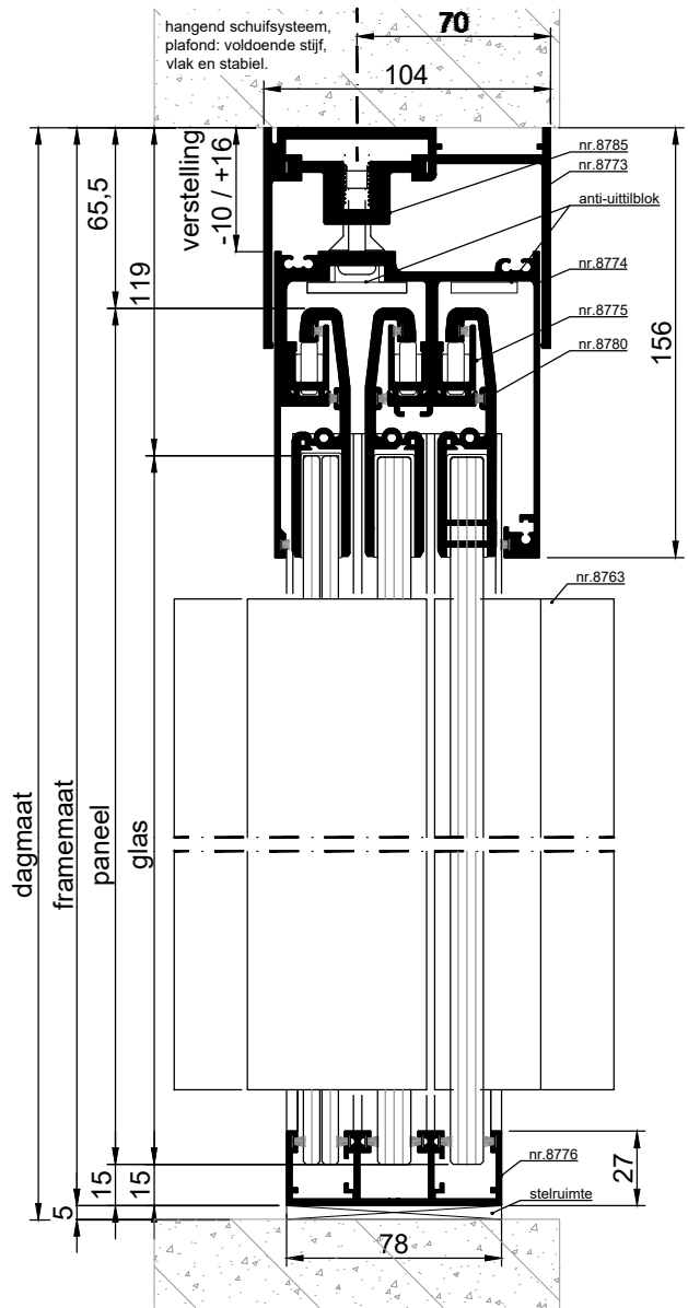
VERTICALE DOORSNEDE type BSH-33A
