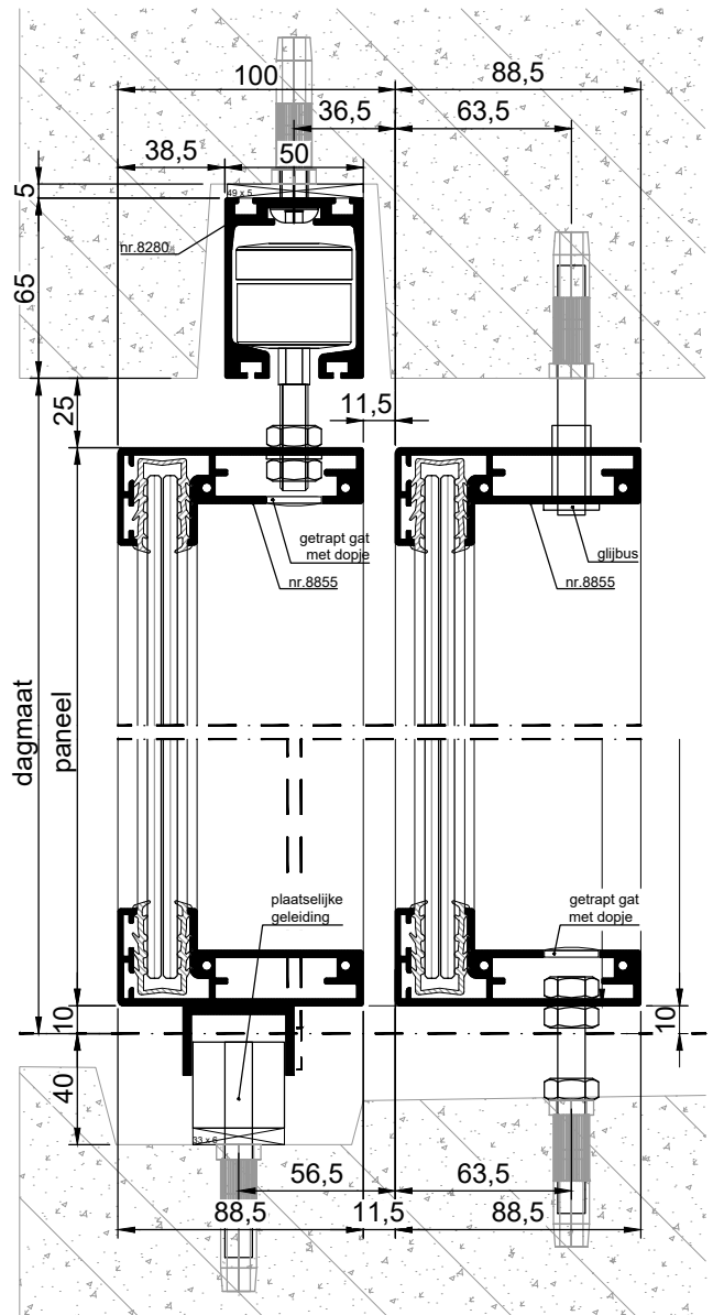
VERTICALE DOORSNEDE type BSH-10A
