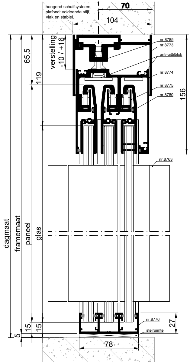
VERTICALE DOORSNEDE type BSH-35A
