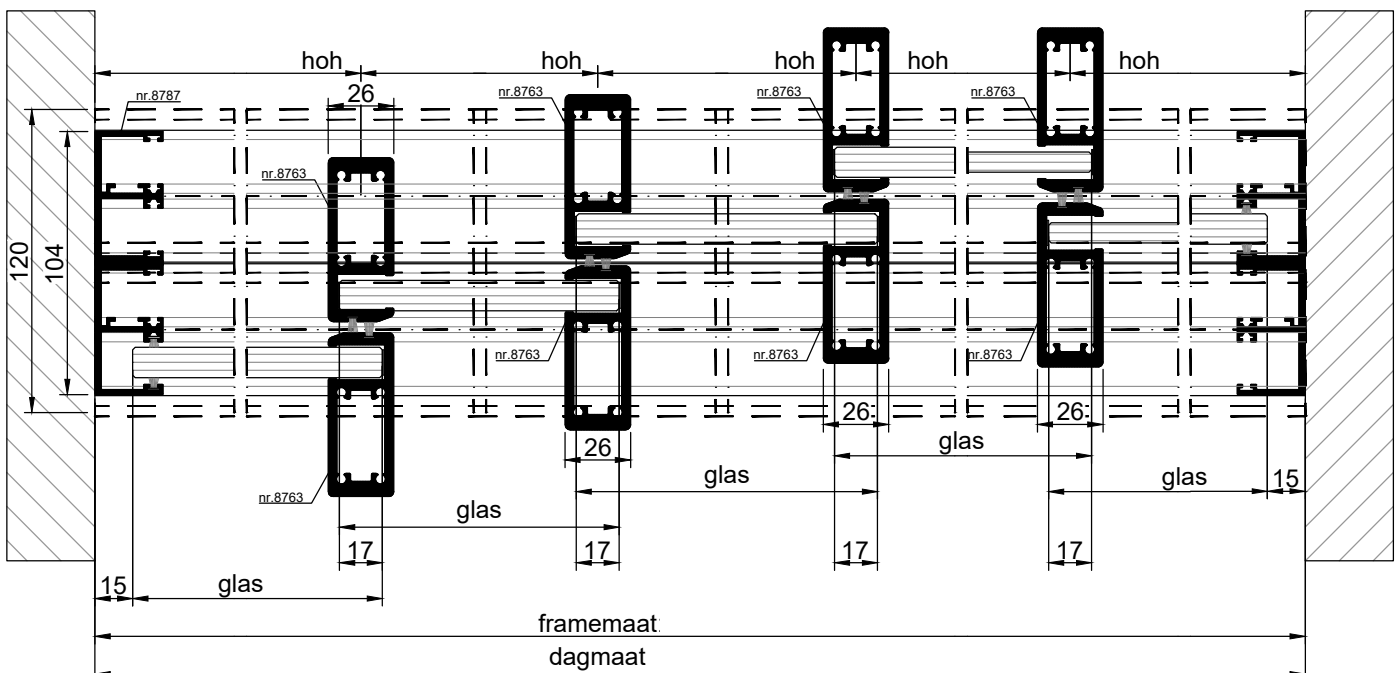
HORIZONTALE DOORSNEDE type BSH-45A
