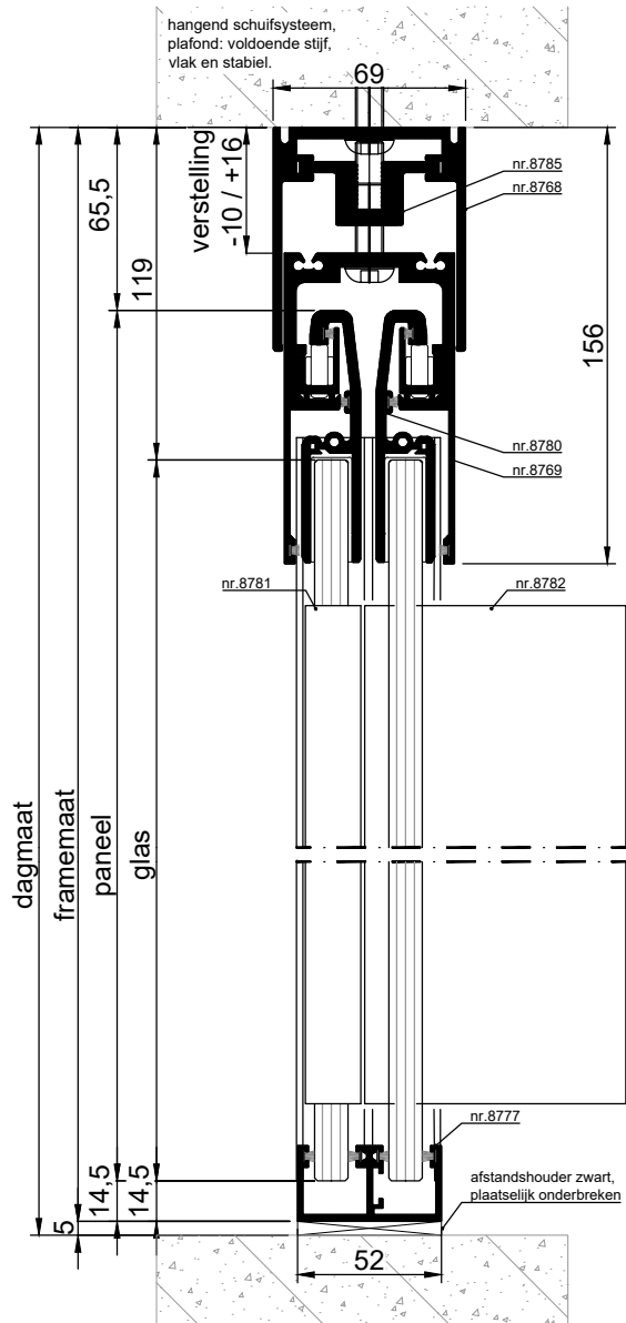
VERTICALE DOORSNEDE type BSH-22B
