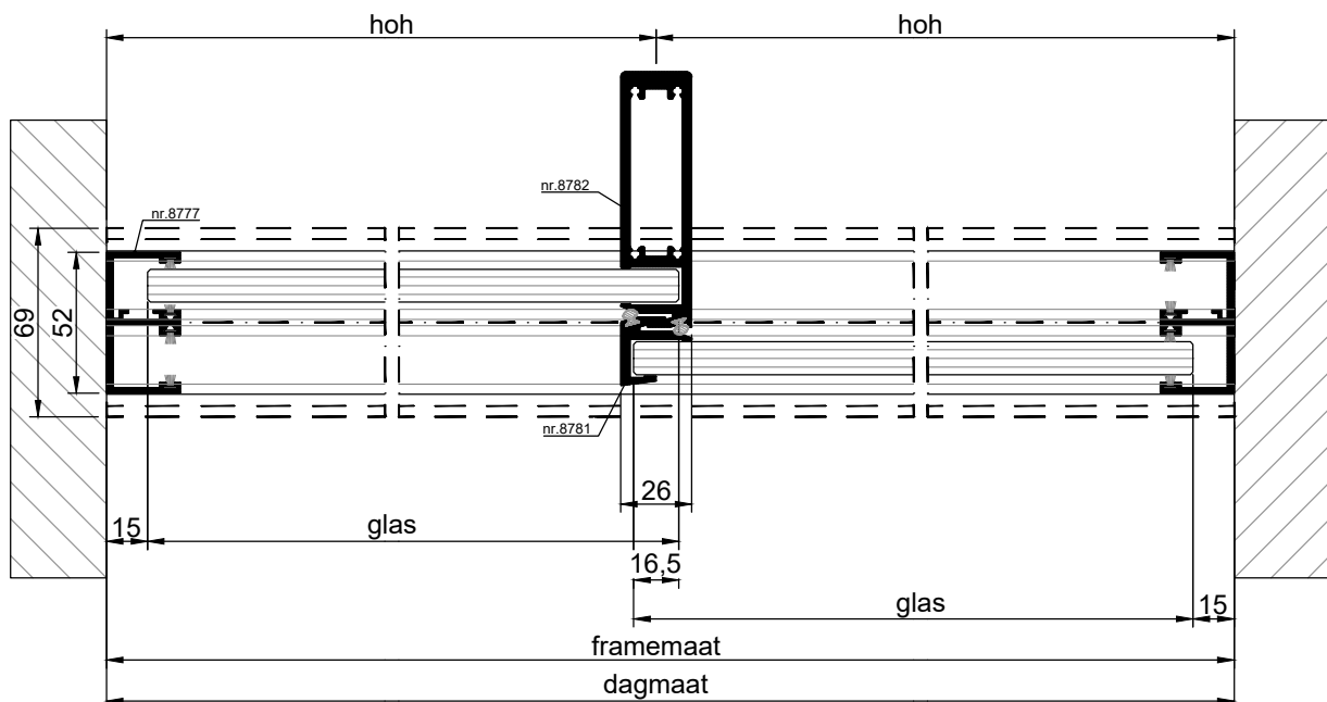
HORIZONTALE DOORSNEDE type BSH-22B
