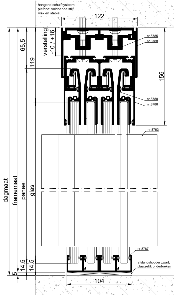
VERTICALE DOORSNEDE type BSH-45A
