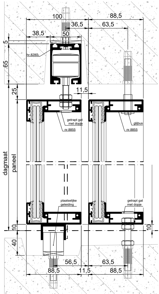
VERTICALE DOORSNEDE type BSH-10E
