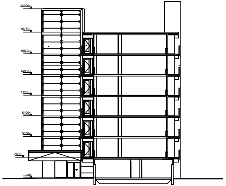
ZIJEAANZICHT GEVELFRAGMENT
